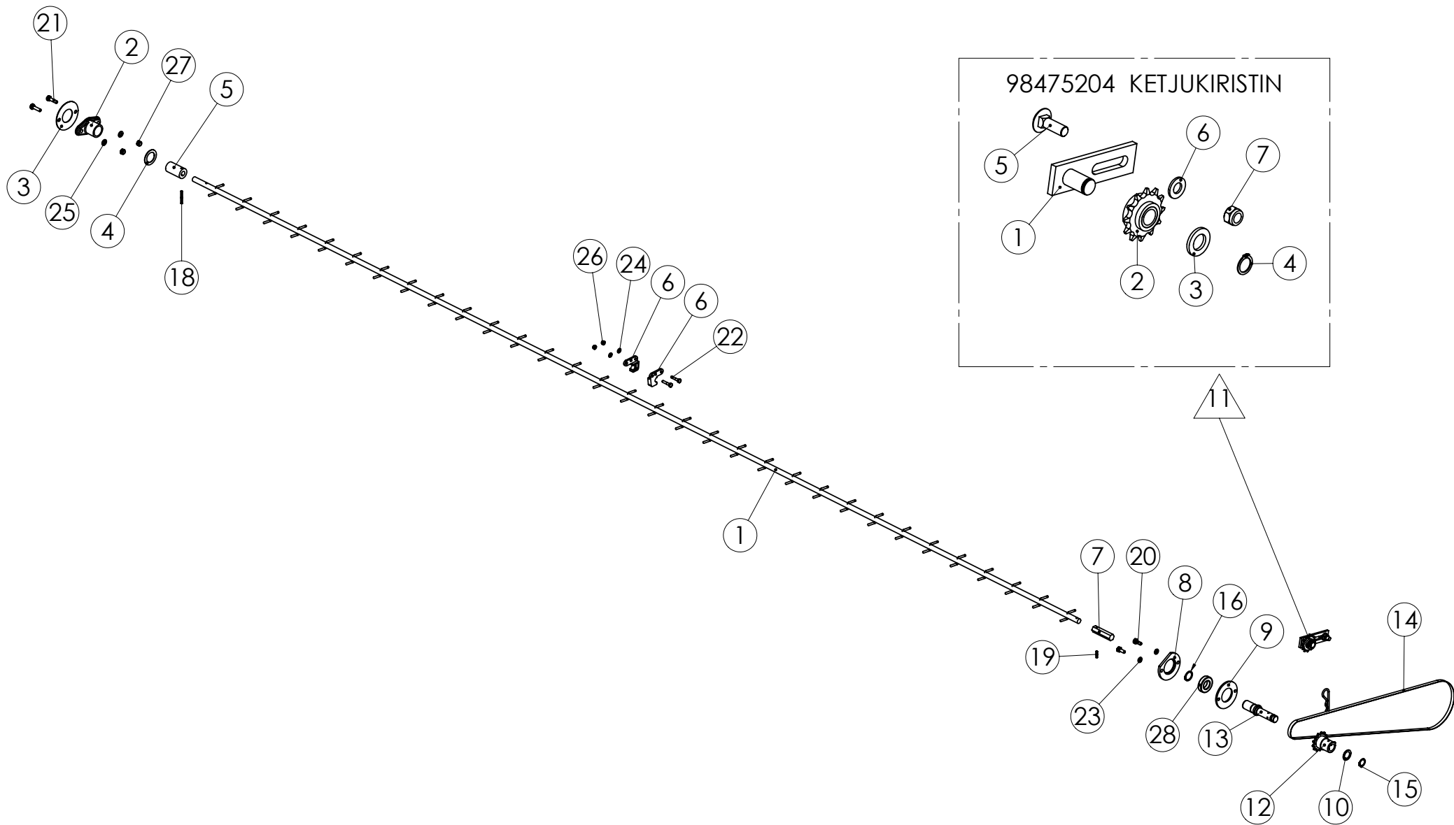
98508401 SIEMENSEKOITUSAKSELI
