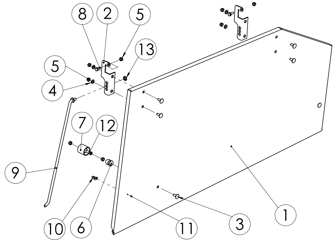
98620603 KANSI OIK.
