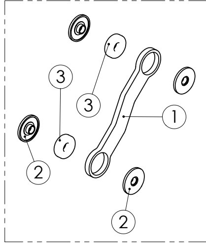
96109904 KIERTOKANKKI
