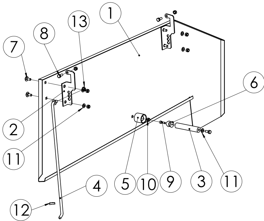
98620503 KANSI VAS.
