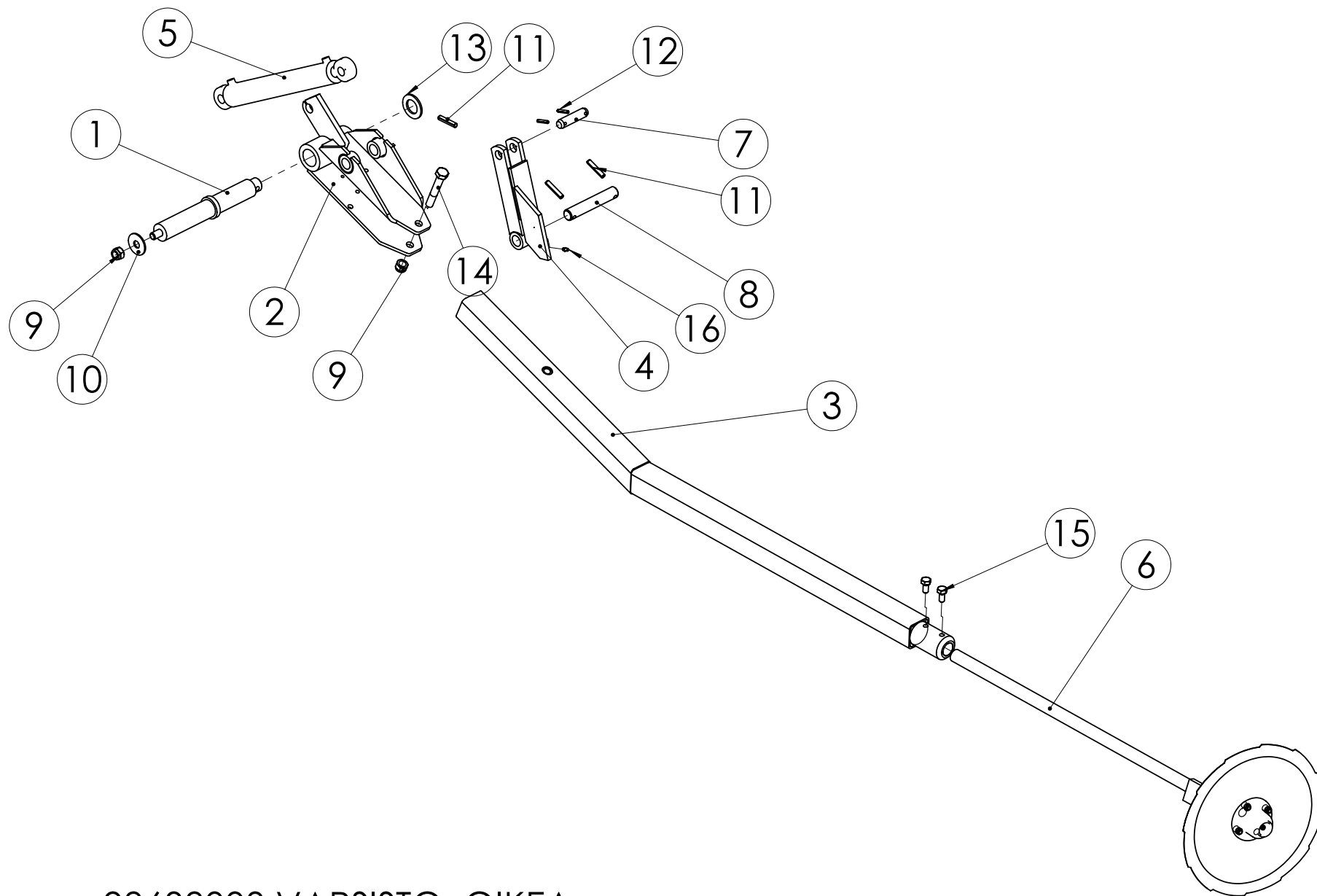
98638003 VARSISTO, OIKEA
