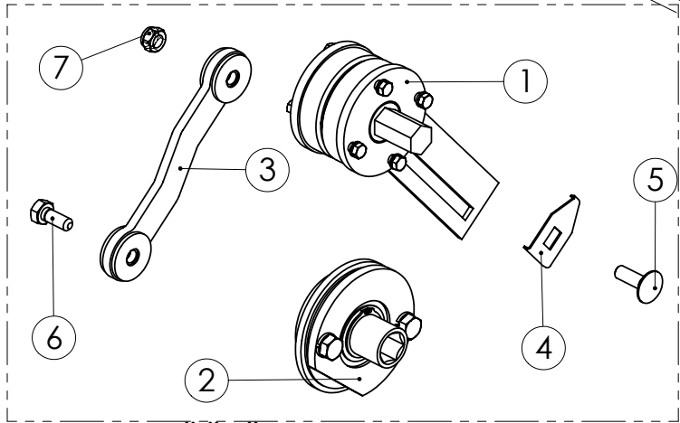
98473004 SÄÄTÖOSAT
