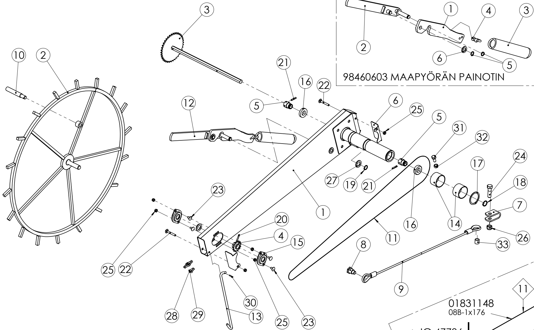
98426301 MAAPYÖRÄ
