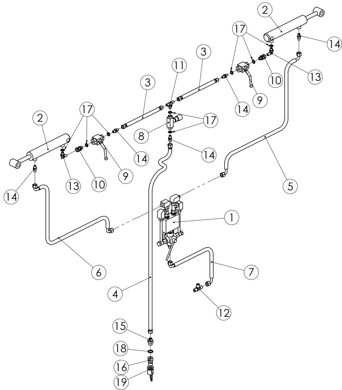
98718902 MERKKARIEN HYDRAULIIKKA VEGA 4000, VAIHTOVENTTIILI
