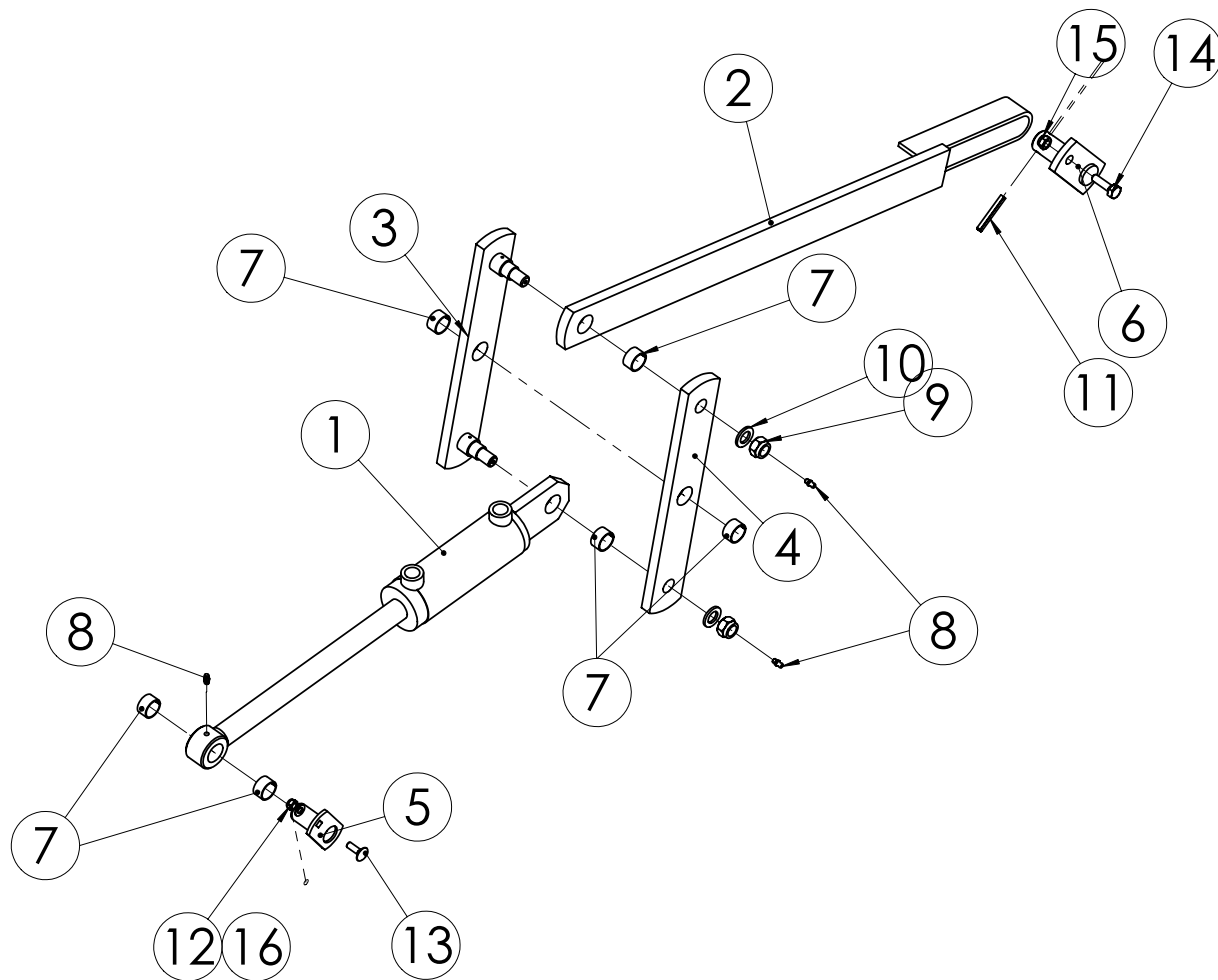
98710604 PAINOTUSVIVUSTO, VEGA 3000-4000
