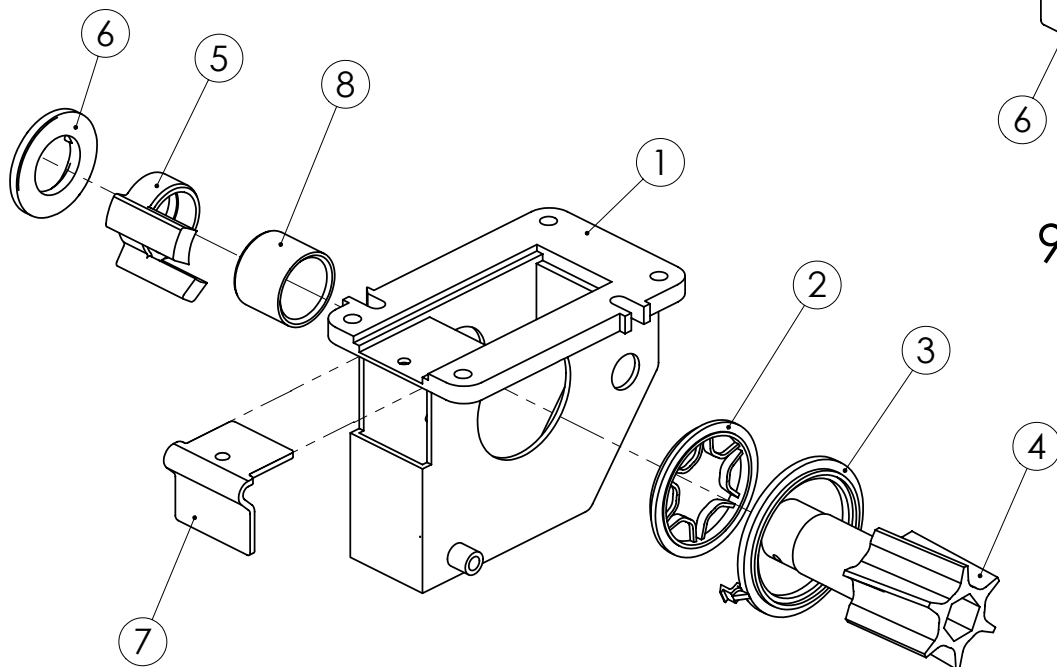
97252703 KYLVÖKAMMIO, LANNOITE
