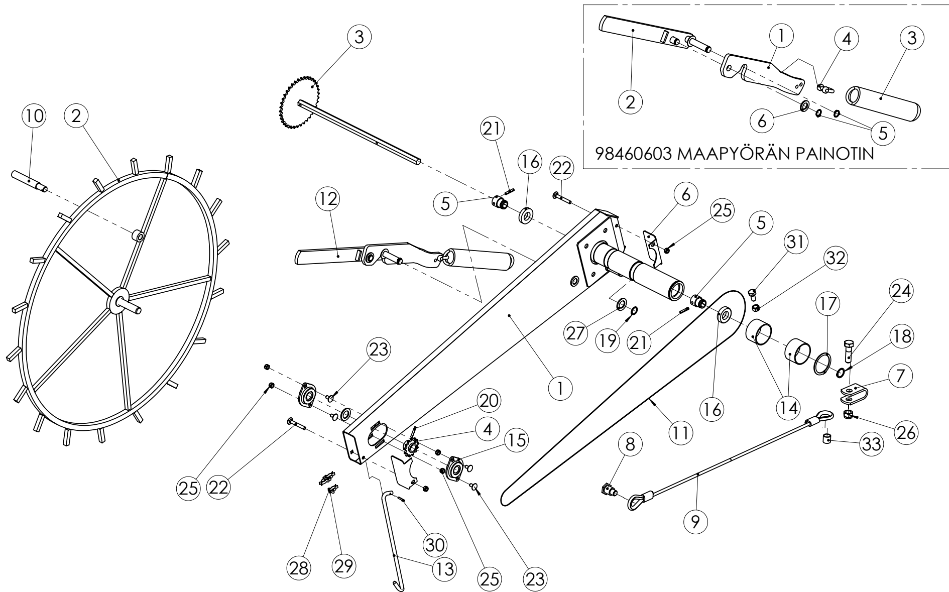
98426301 MAAPYÖRÄ
