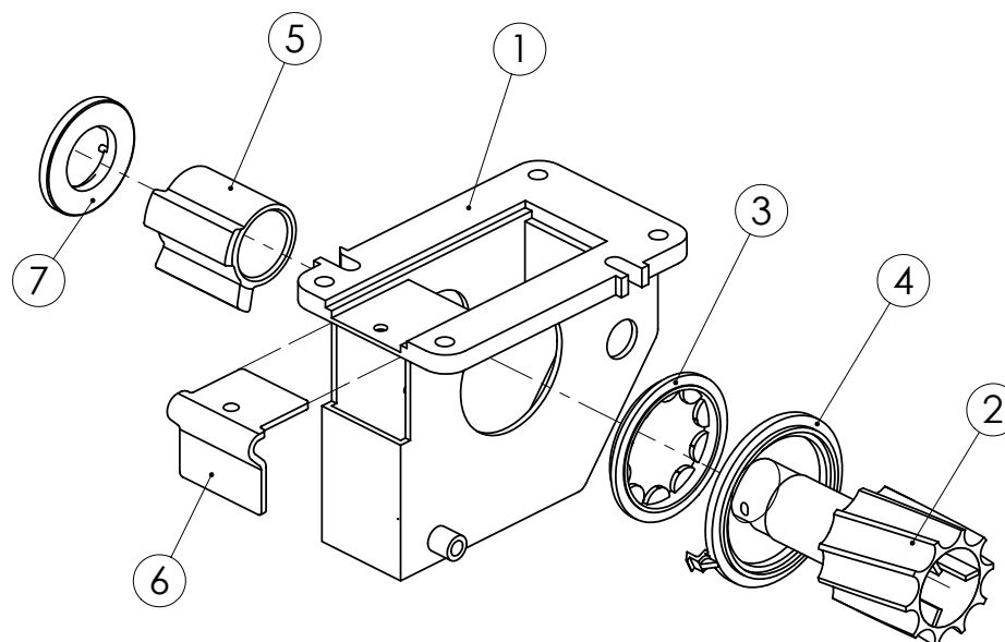
96202503 KYLVÖKAMMIO, SIEMEN
