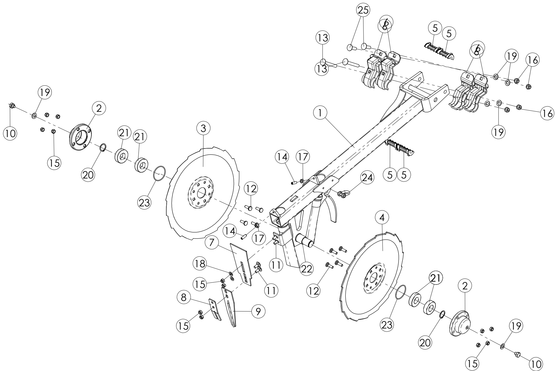
98980602 VANNAS VASEN
