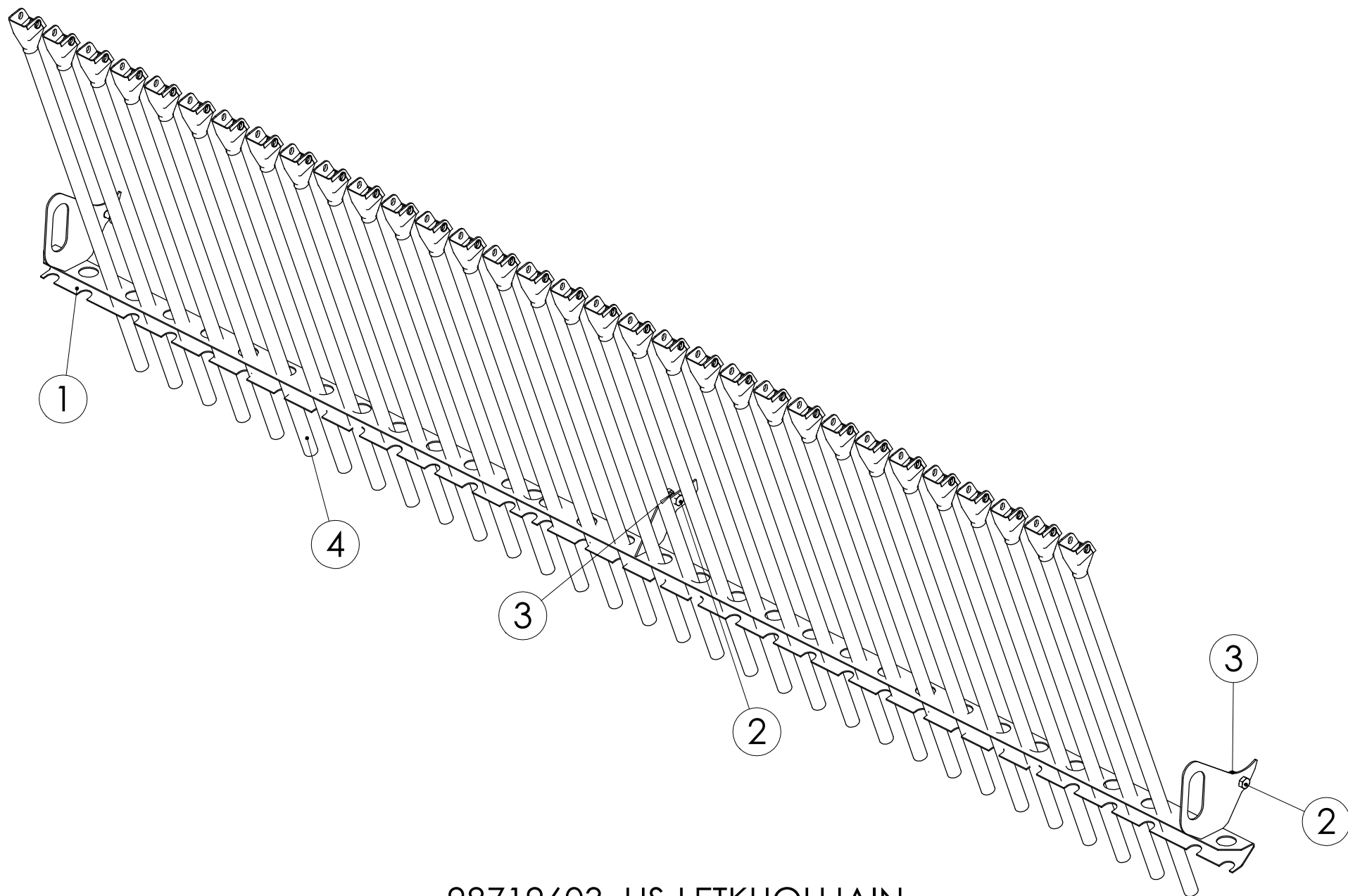
98719603 HS-LETKUOHJAIN
