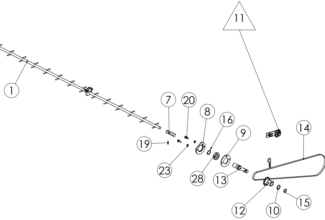
98508401 SIEMEN SEKOITUSAKSELI
