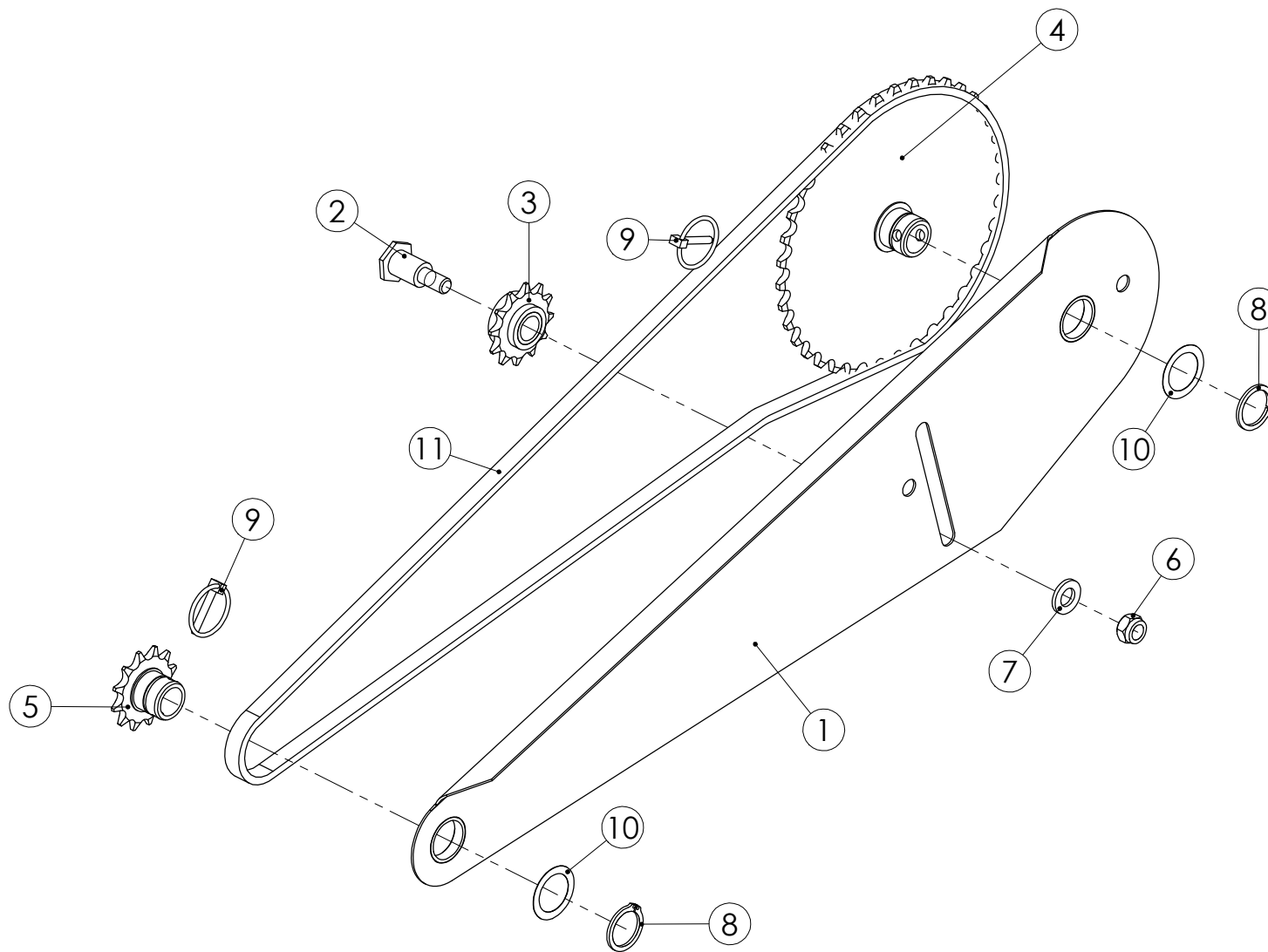
99101403 HYBRIDI-VÄLITYS
