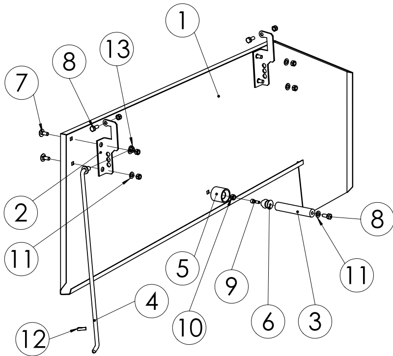
98620503 KANSI VAS.
