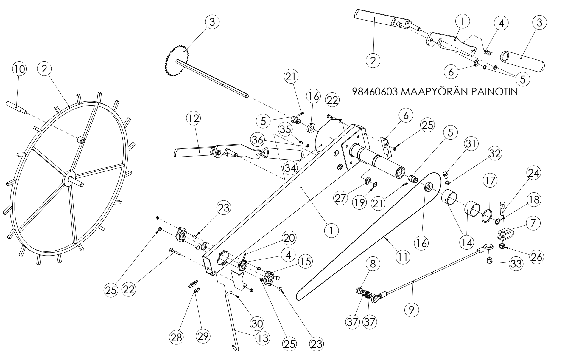
98426301 MAAPYÖRÄ
