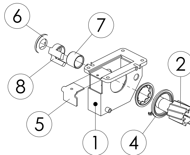
LANNOITE KYLVÖKAMMIO 98314803
