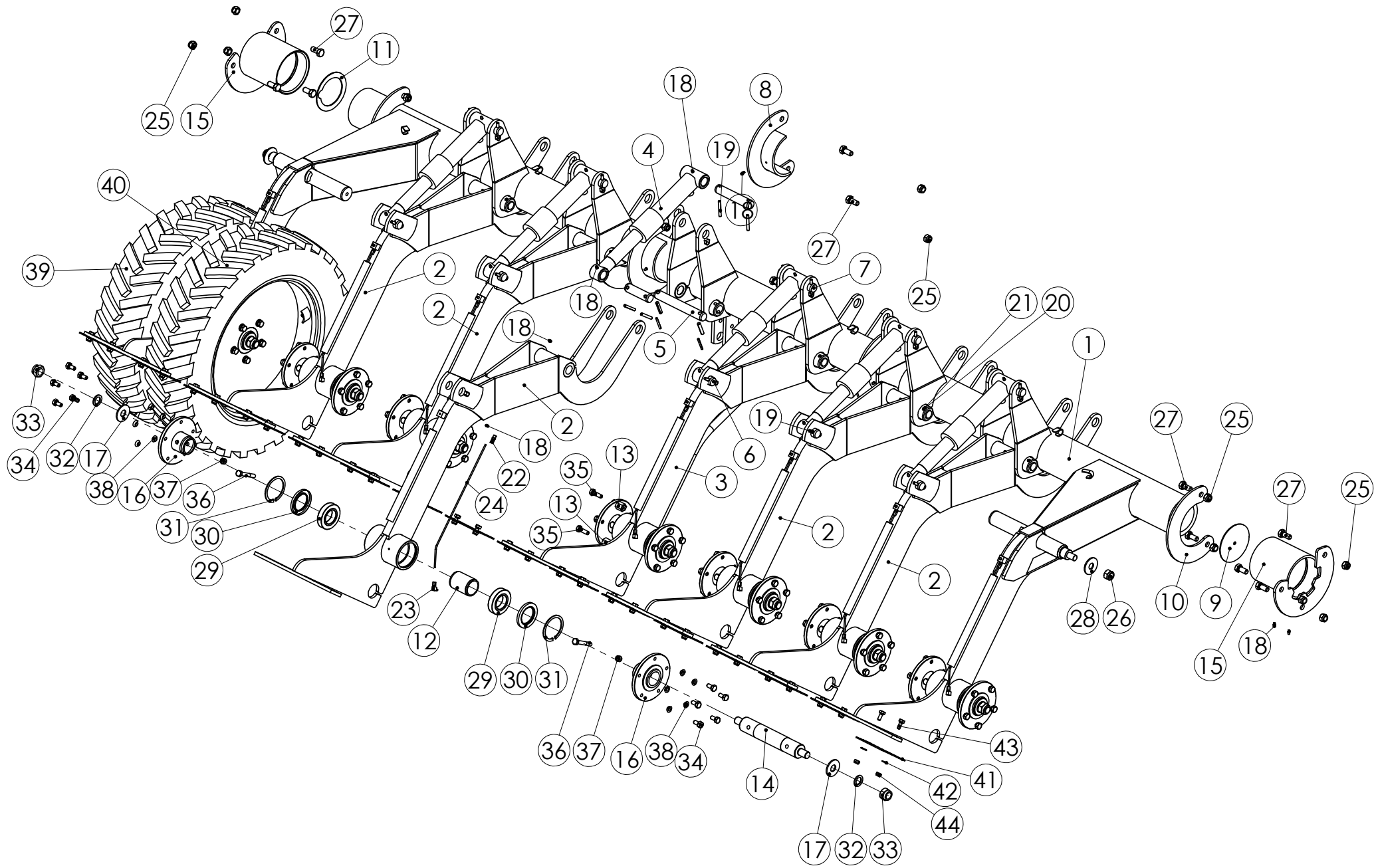
99072002 JYRÄPYÖRÄSTÖ TITAN 4000
