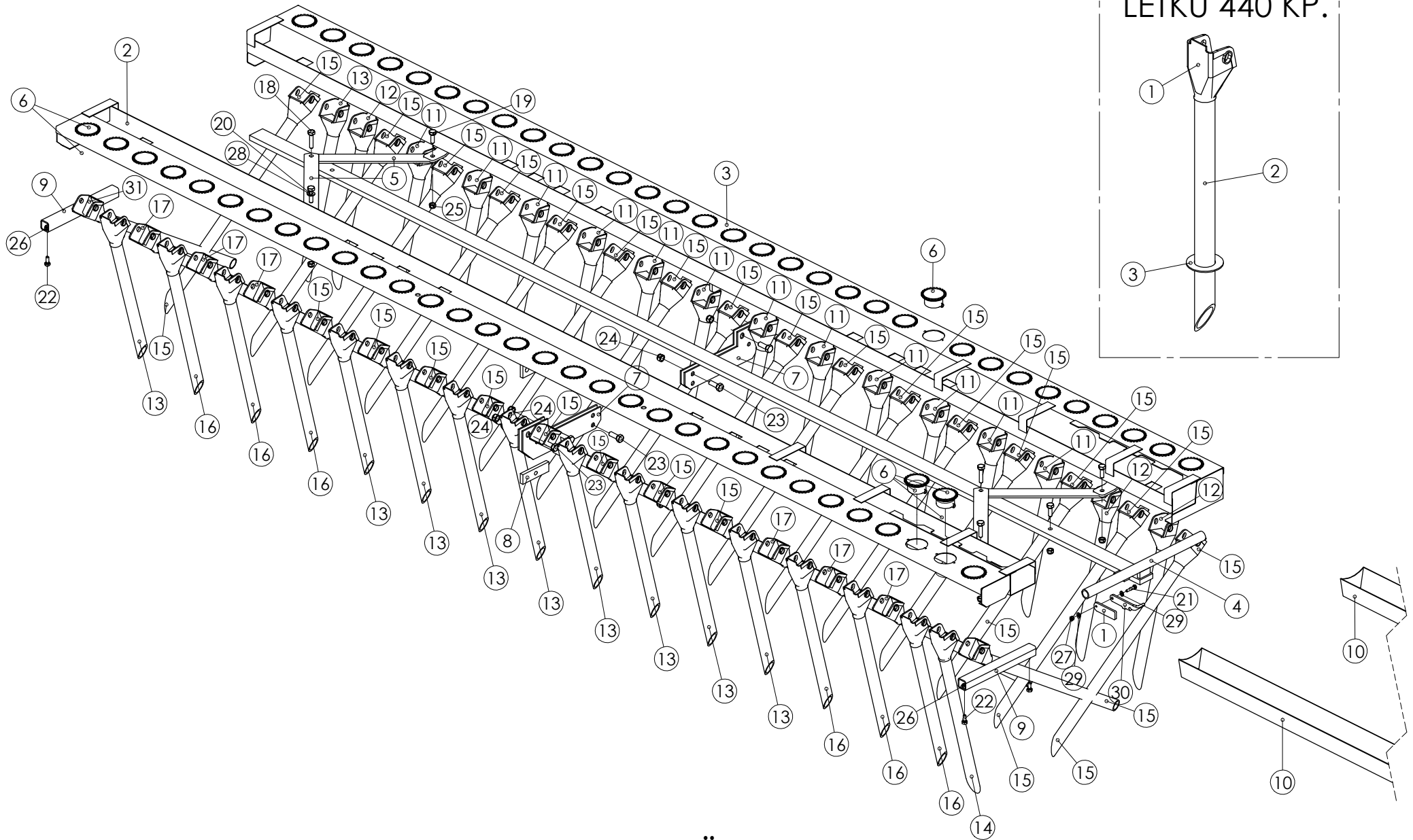
98993502 HYLLEYKÖ 4000
