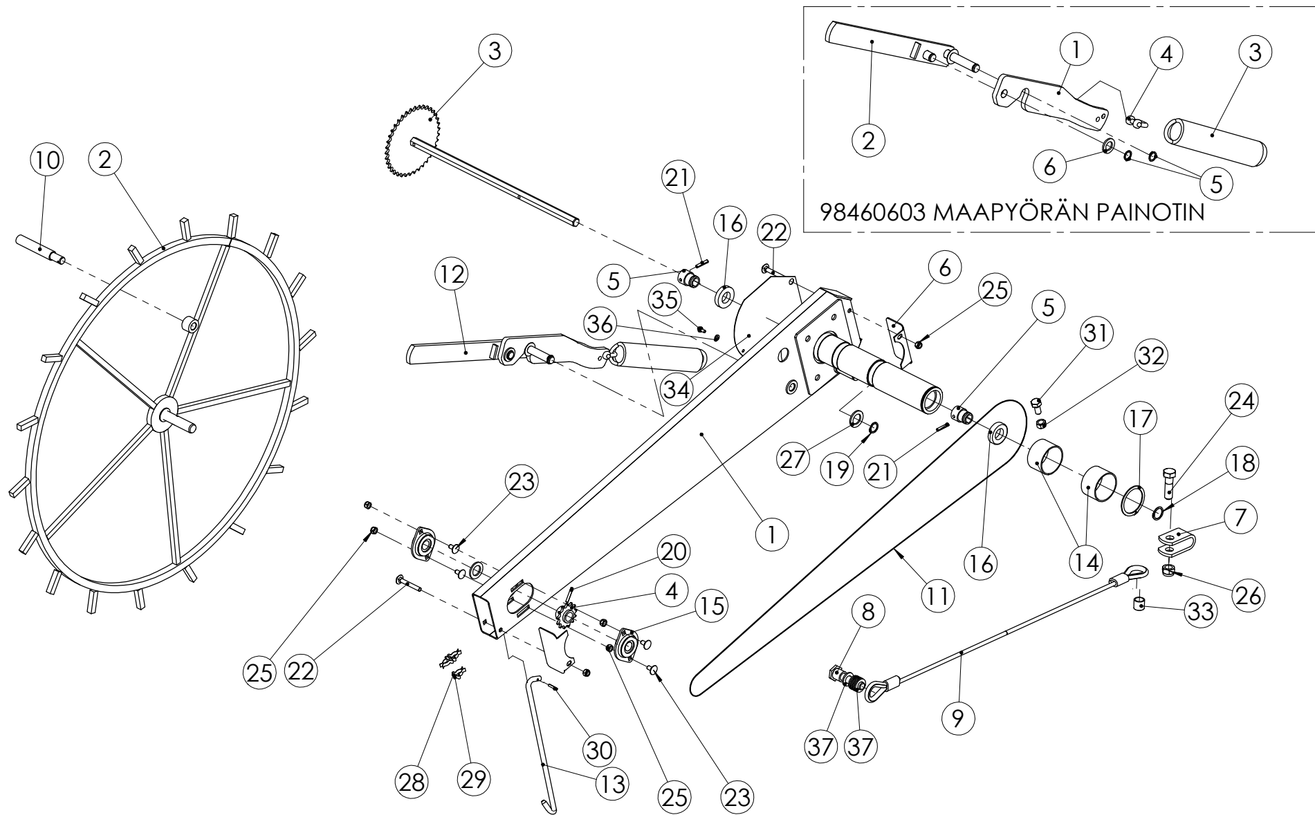
98426301 MAAPYÖRÄ
