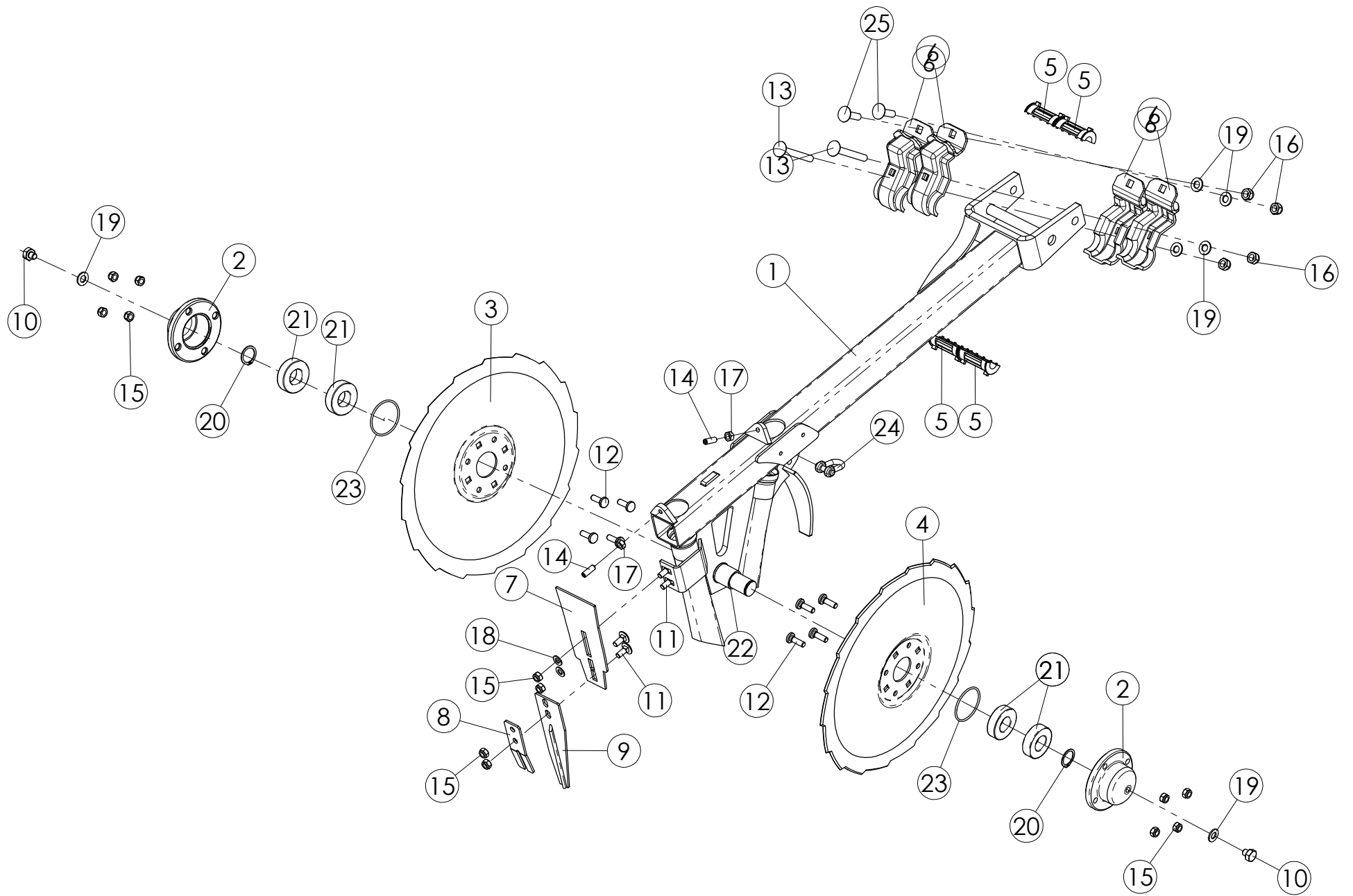
98980602 VANNAS VASEN
