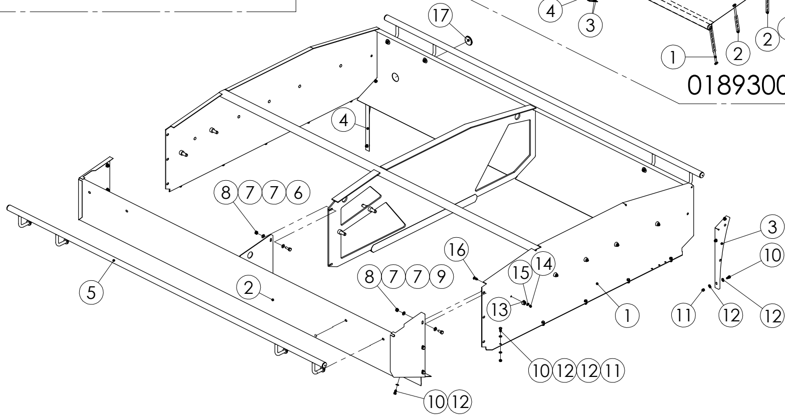
98448302 SÄILIÖ 3000
