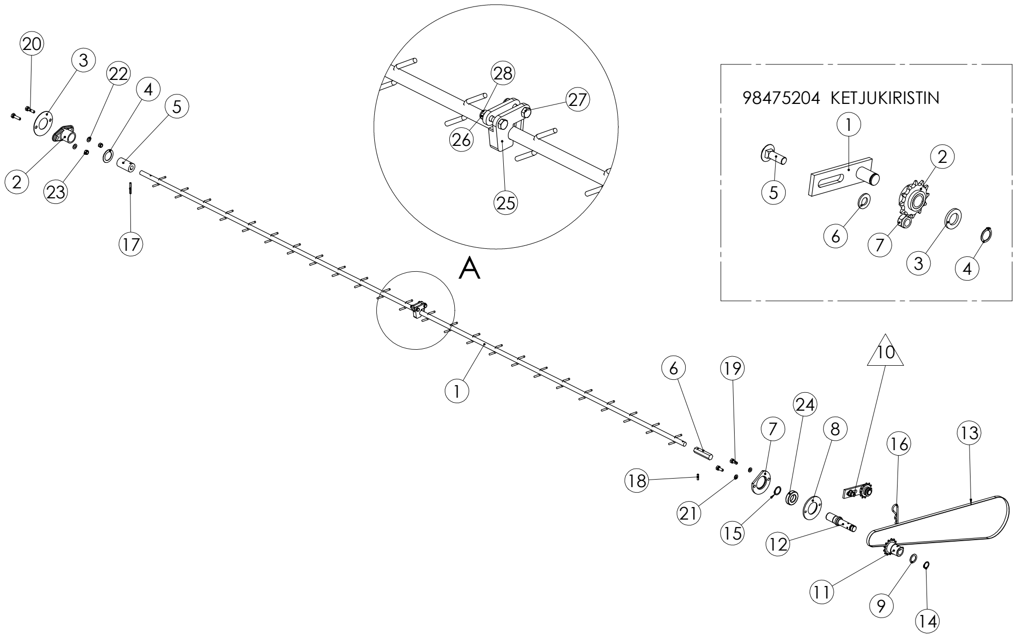
98308002 SIEMEN SEKOITUSAKSELI
