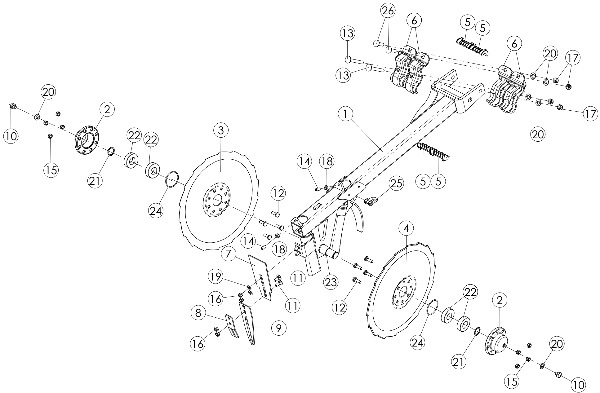
98980602 VANNAS VASEN
