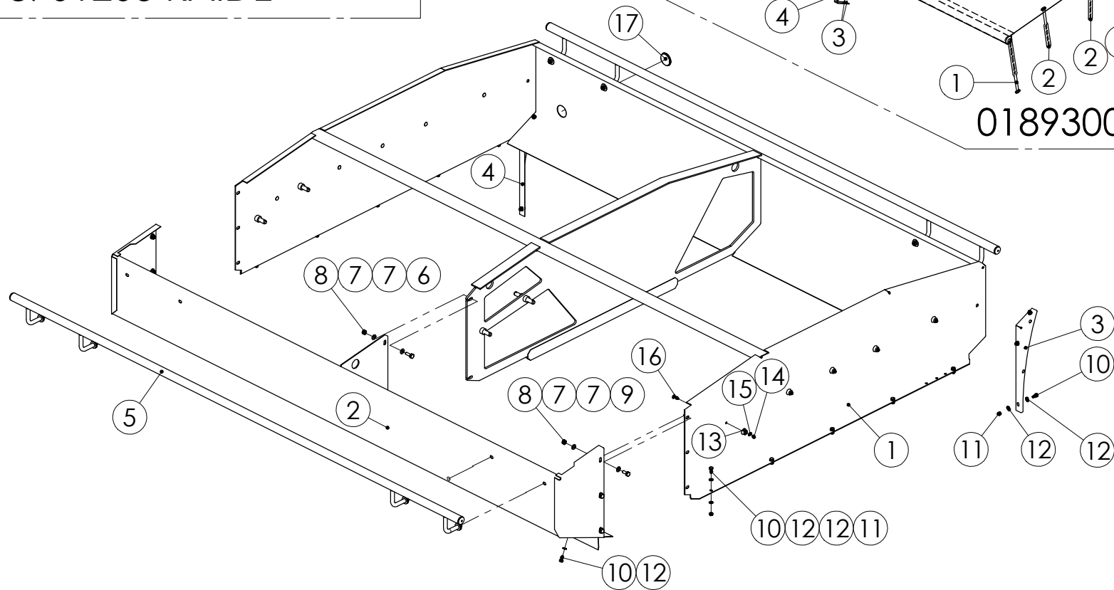
98448302 SÄILIÖ 3000
