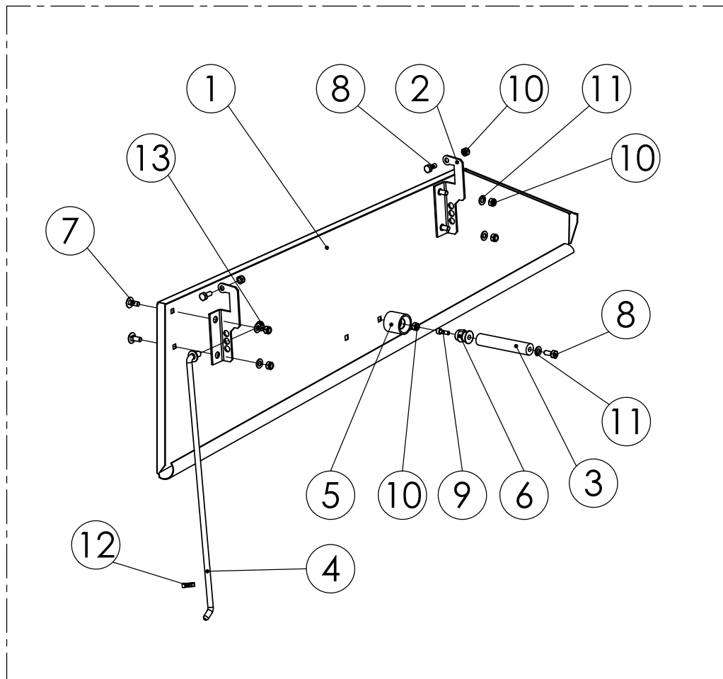
98331803 KANSI VAS. KP.
