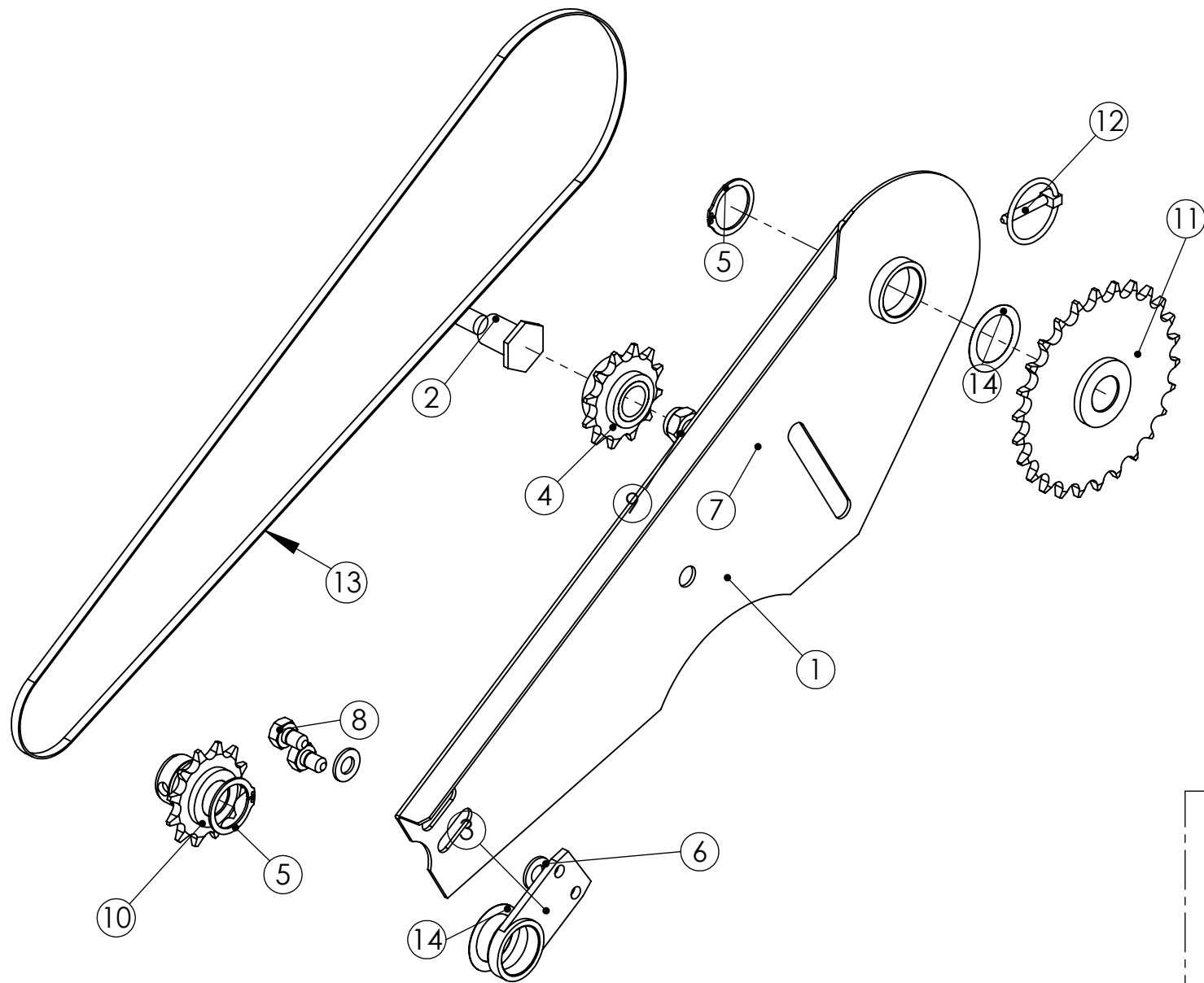
98314404 KETJUNKIRISTIN Z12 L=42
