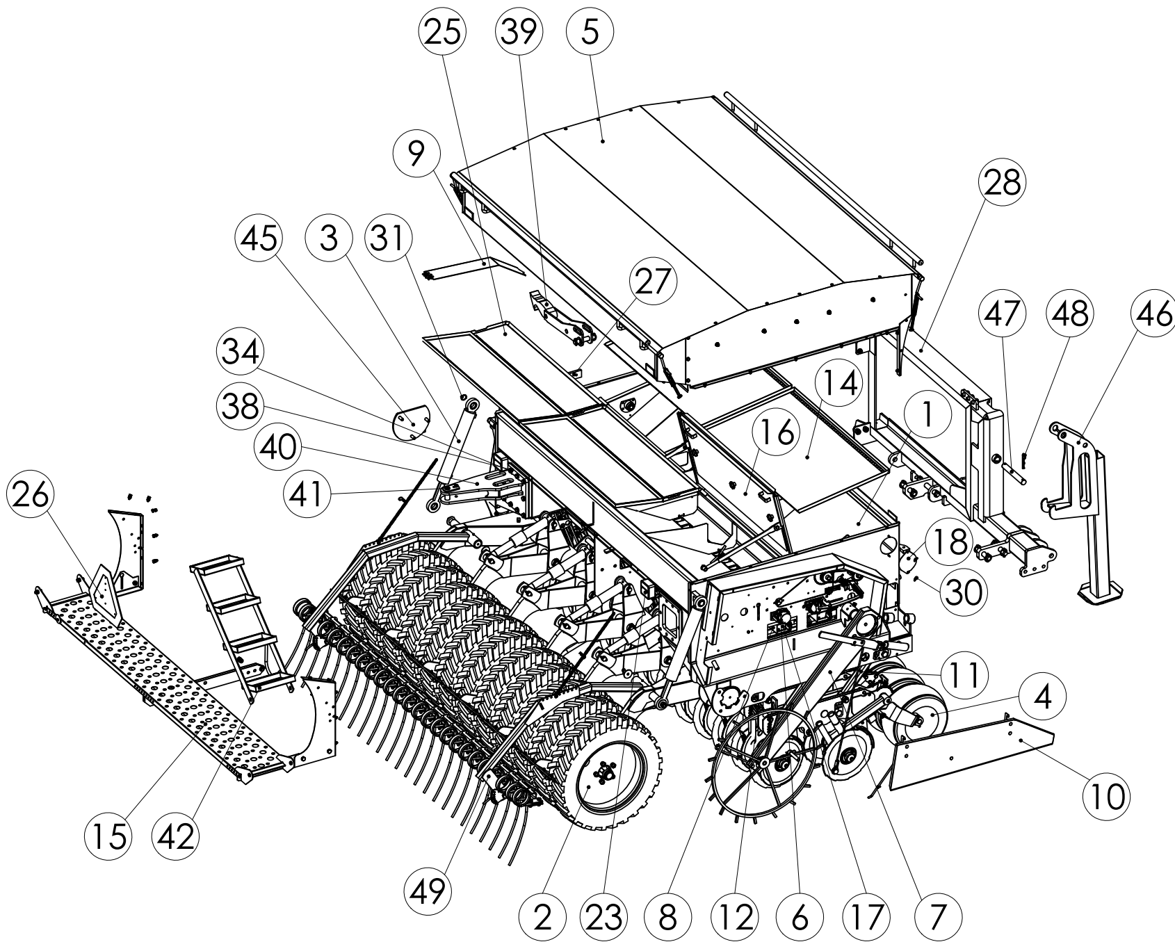
98959402 NOVA COMBI 6000 OIkea
