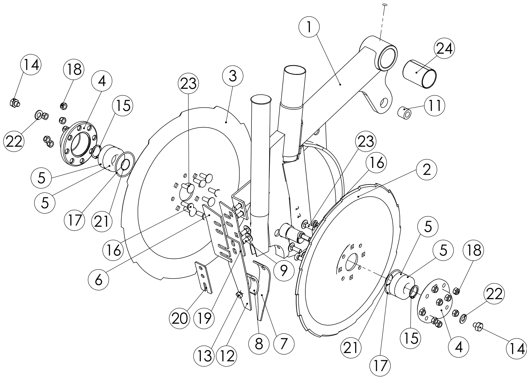
98374802 TAKAVANNAS
