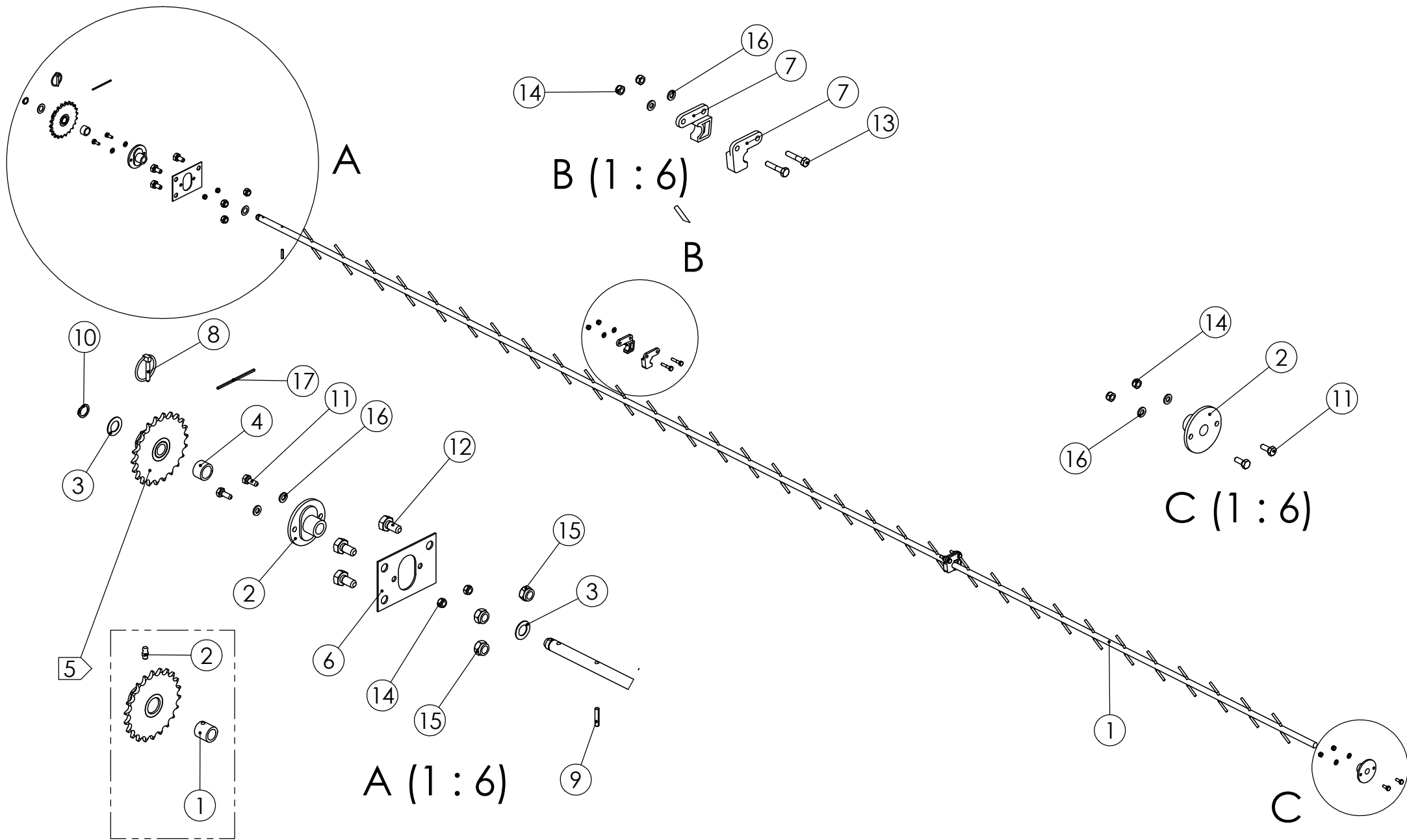
98507801 LANNOITE SEKOITUSAKSELI 4000
