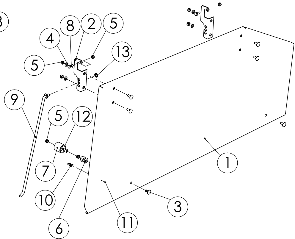
98331303 KANSI OIK.
