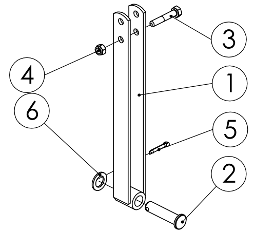
98320704 NOSTOTANKO
