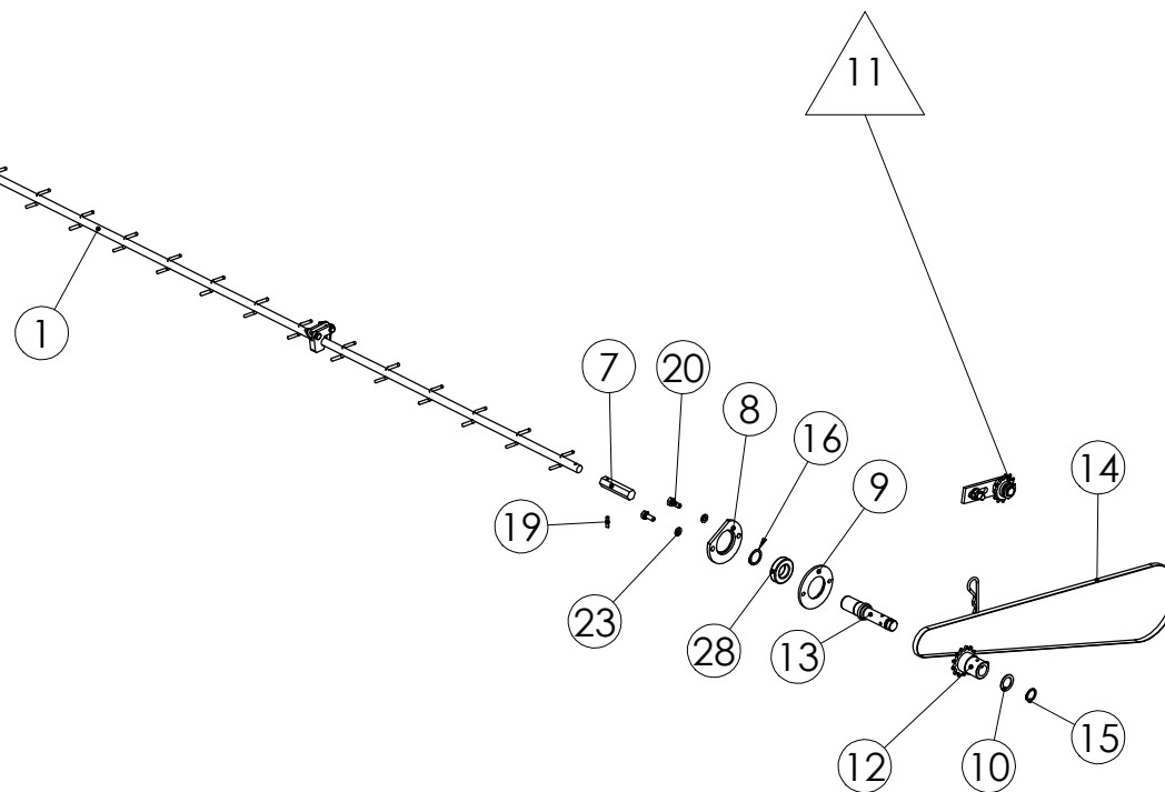
98508401 SIEMEN SEKOITUSAKSELI
