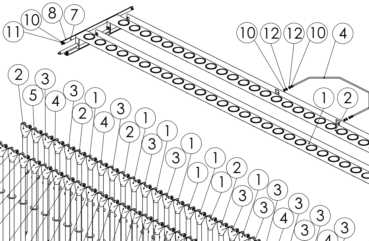
99085403 HYLLYKKÖ 4000
