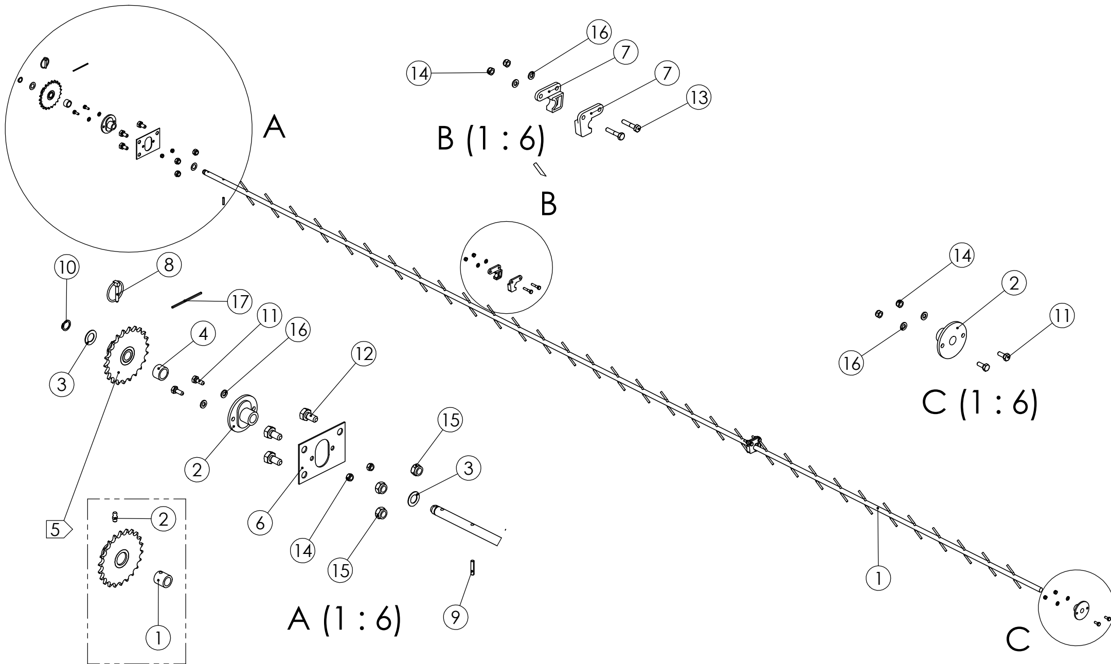
98507801 LANNOITE SEKOITUSAKSELI 4000
