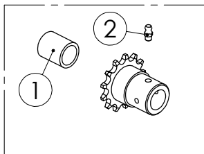
98305844 KETJUPYÖRÄ
