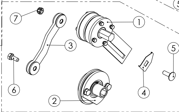
98473004 SÄÄTÖOSAT
