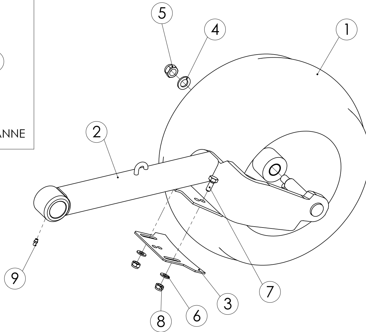
98350003 KANNATUSPYÖRÄ
