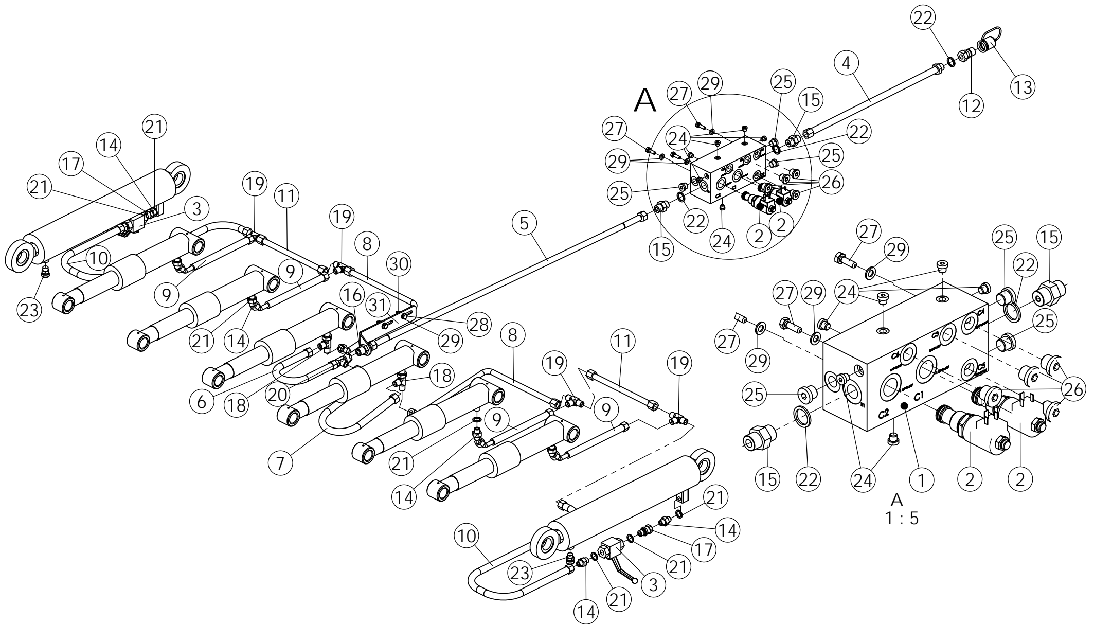
98940702 HYDRAULIIKKA 4000
