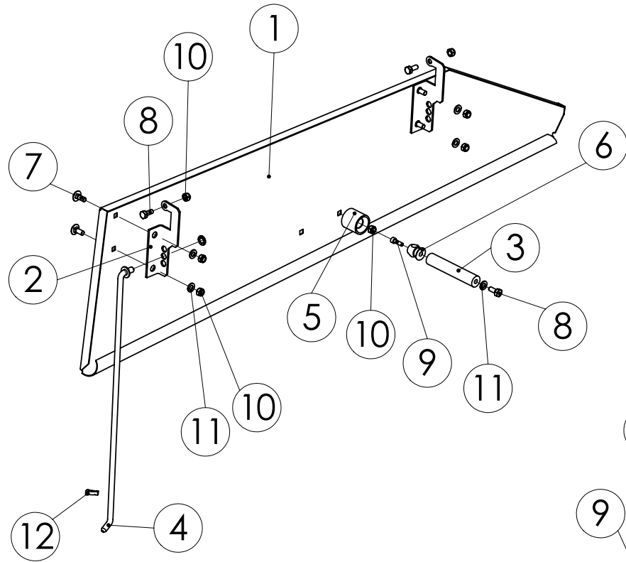
98331373 KANSI VAS.
