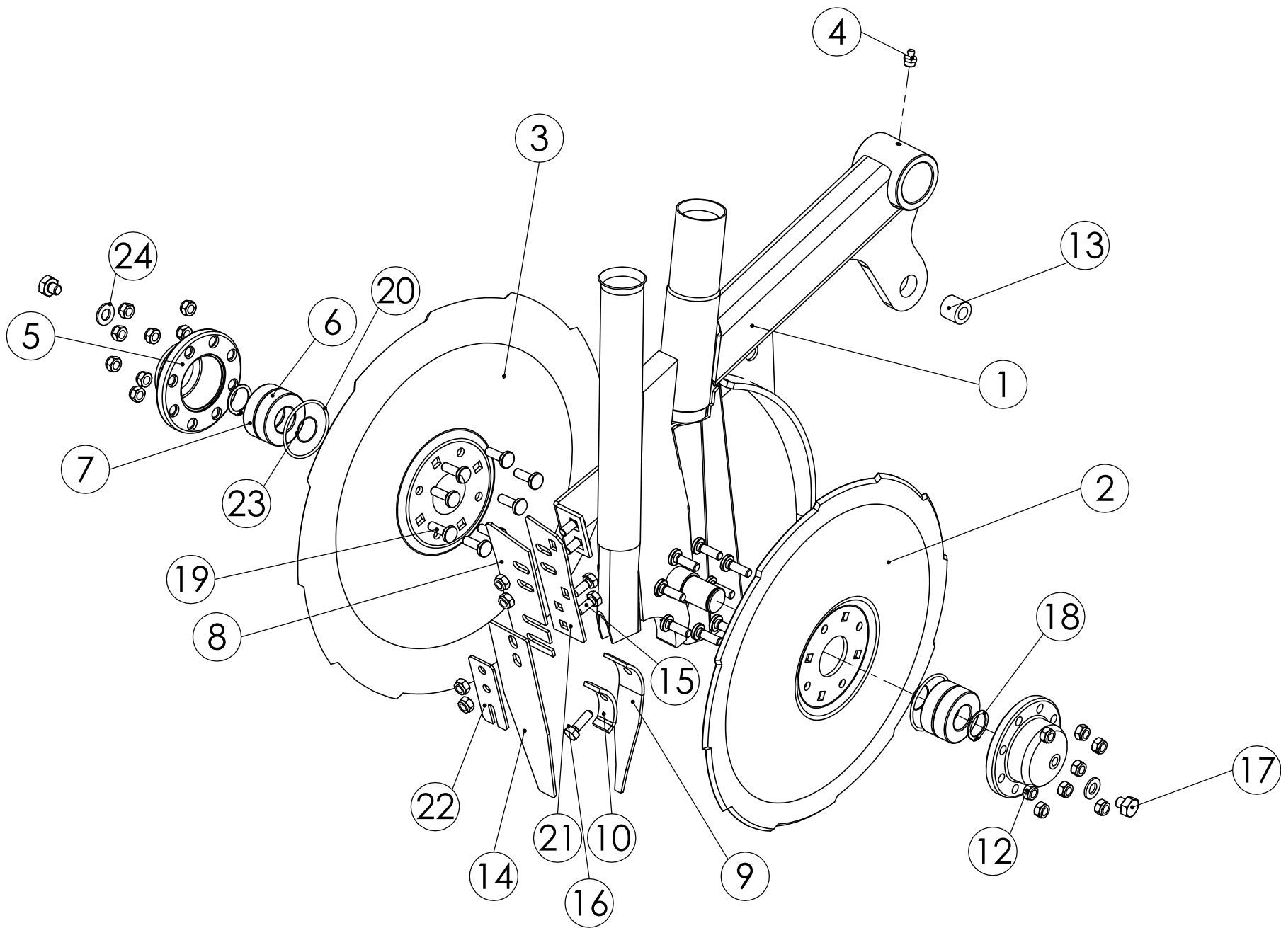
98374802 TAKAVANNAS
