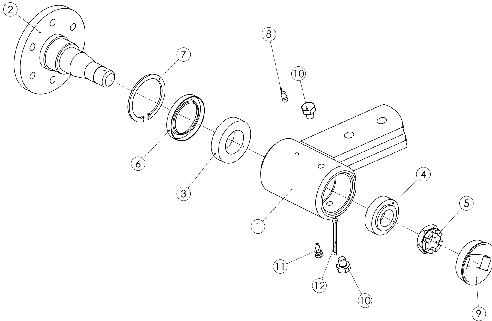
98473604 LAAKEROINTI
