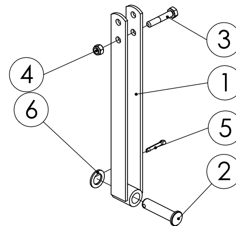
98320704 NOSTOTANKO
