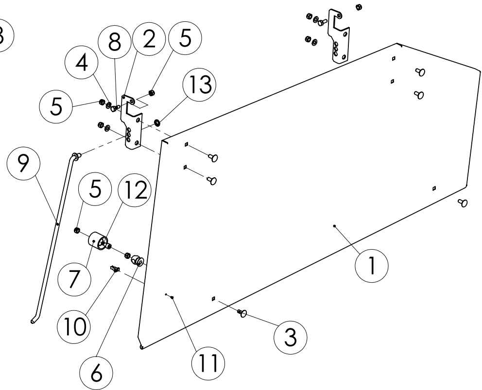
98331873 KANSI OIK.
