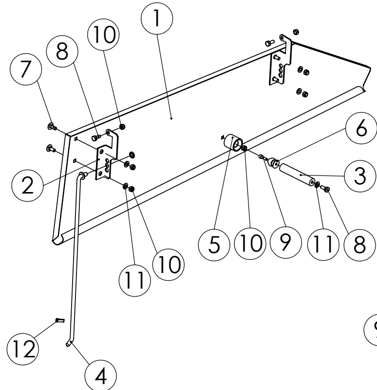
98331373 KANSI VAS.
