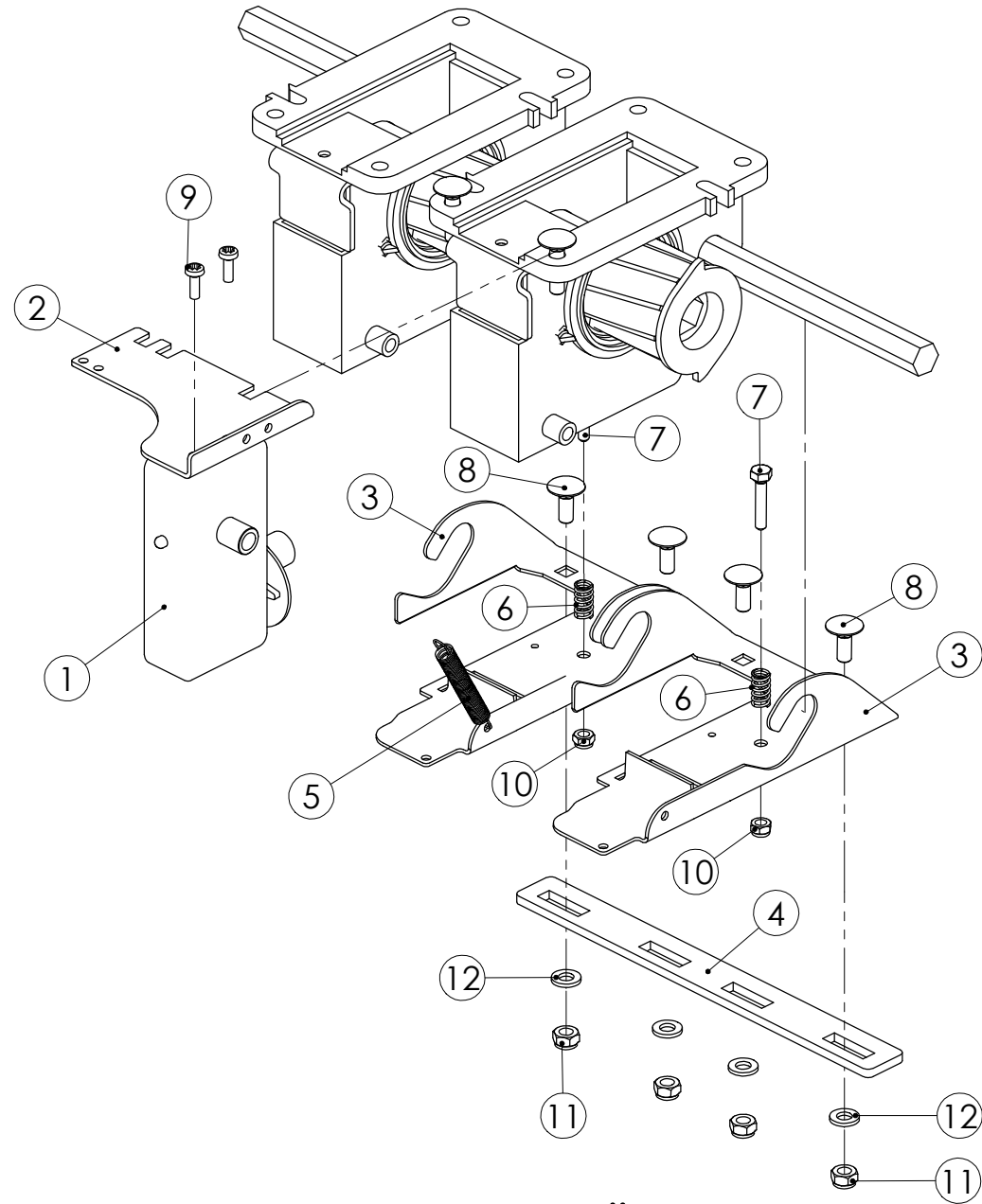
99012603 AJOURAPYSÄYTIN
