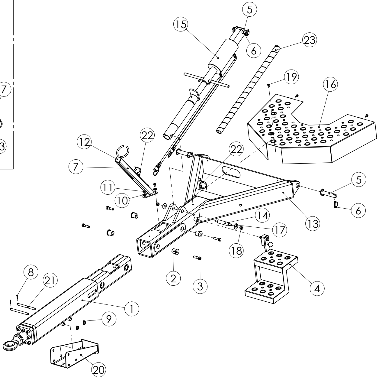
99079703 VETOLAITE 3000
