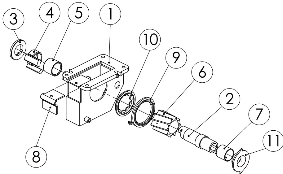
98453703 AJOURAKAMMIOKAMMIO LANNOITE
