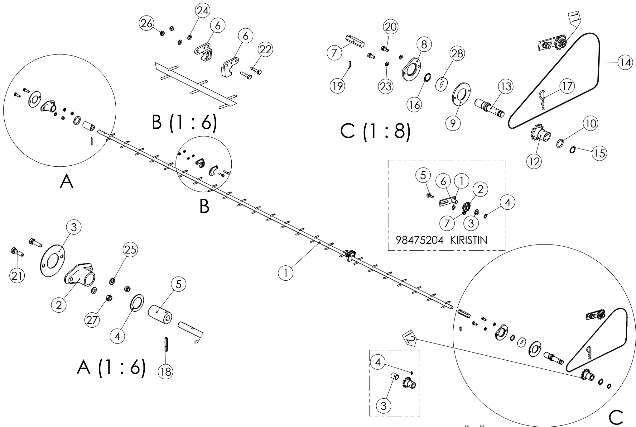
98446601 SIEMEN SEKOITUSAKSELI 3000
