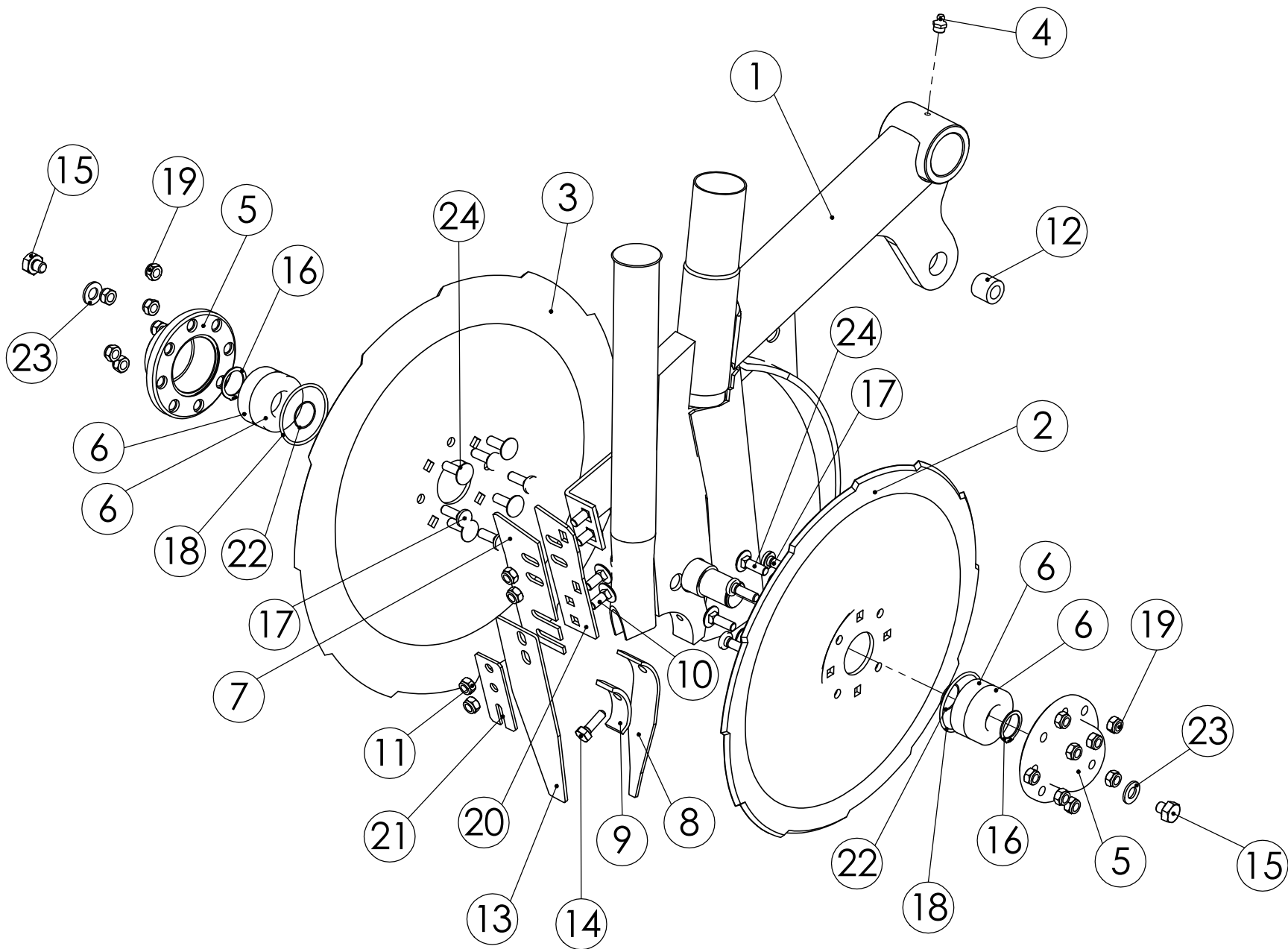
98374802 TAKAVANNAS
