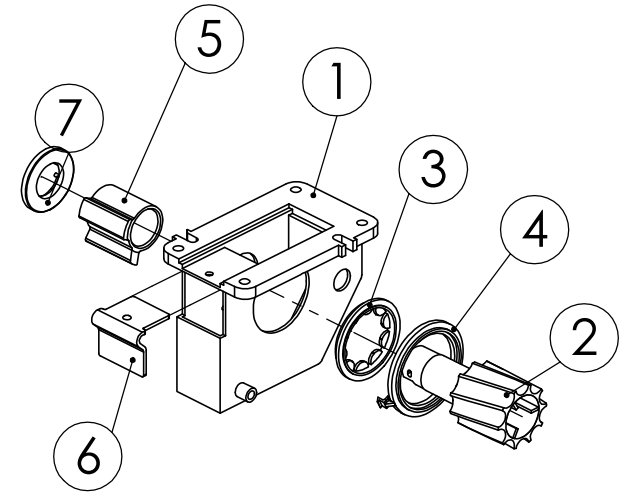
96202503 KYLVÖKAMMIO KP.
