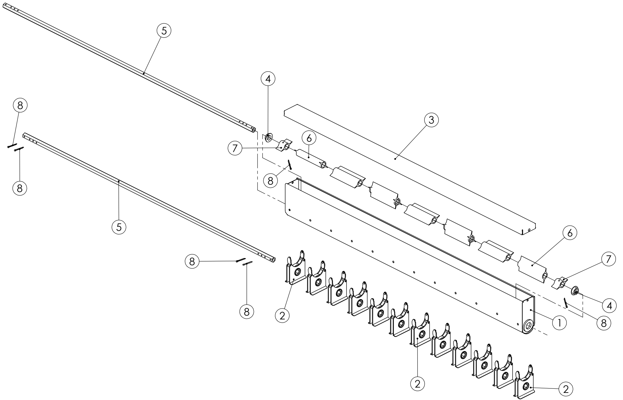
98385001 SYÖTTÖKAUKALO 3000
