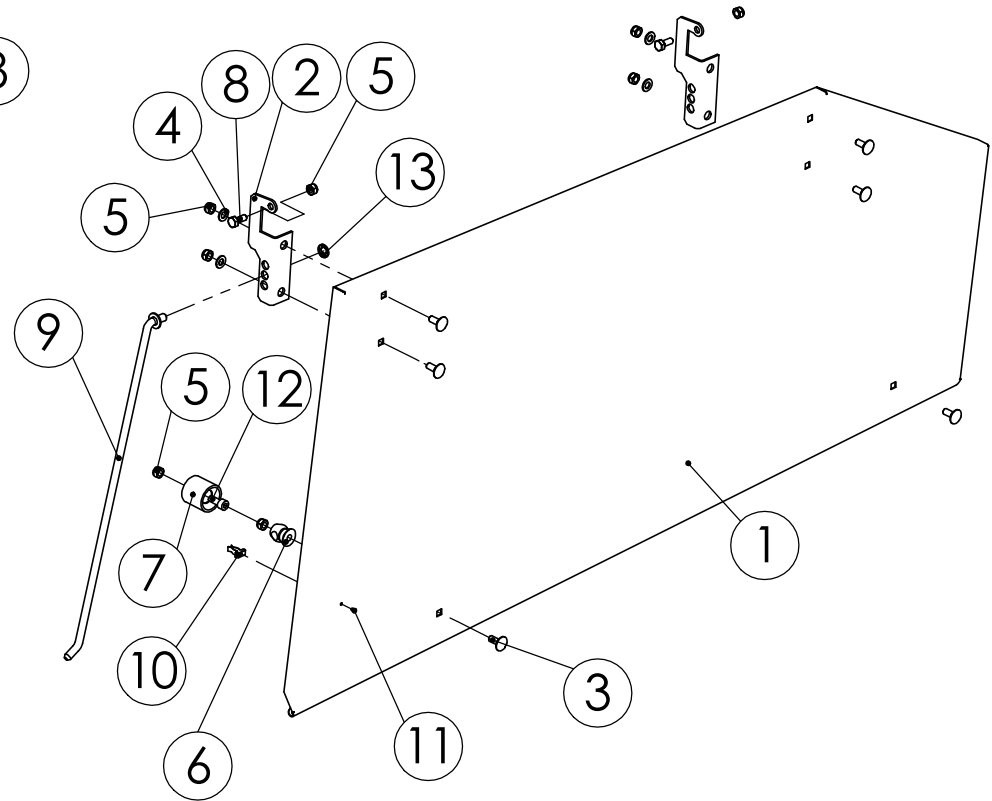
98331303 KANSI OIK.
