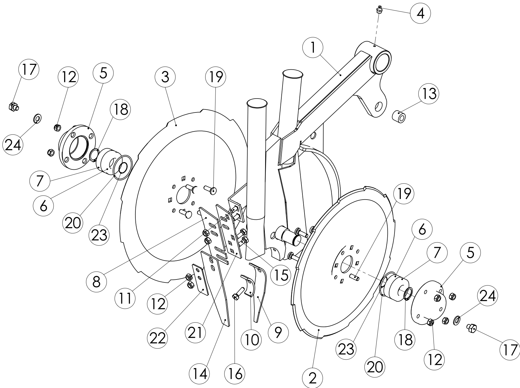
98374802 TAKAVANNAS
