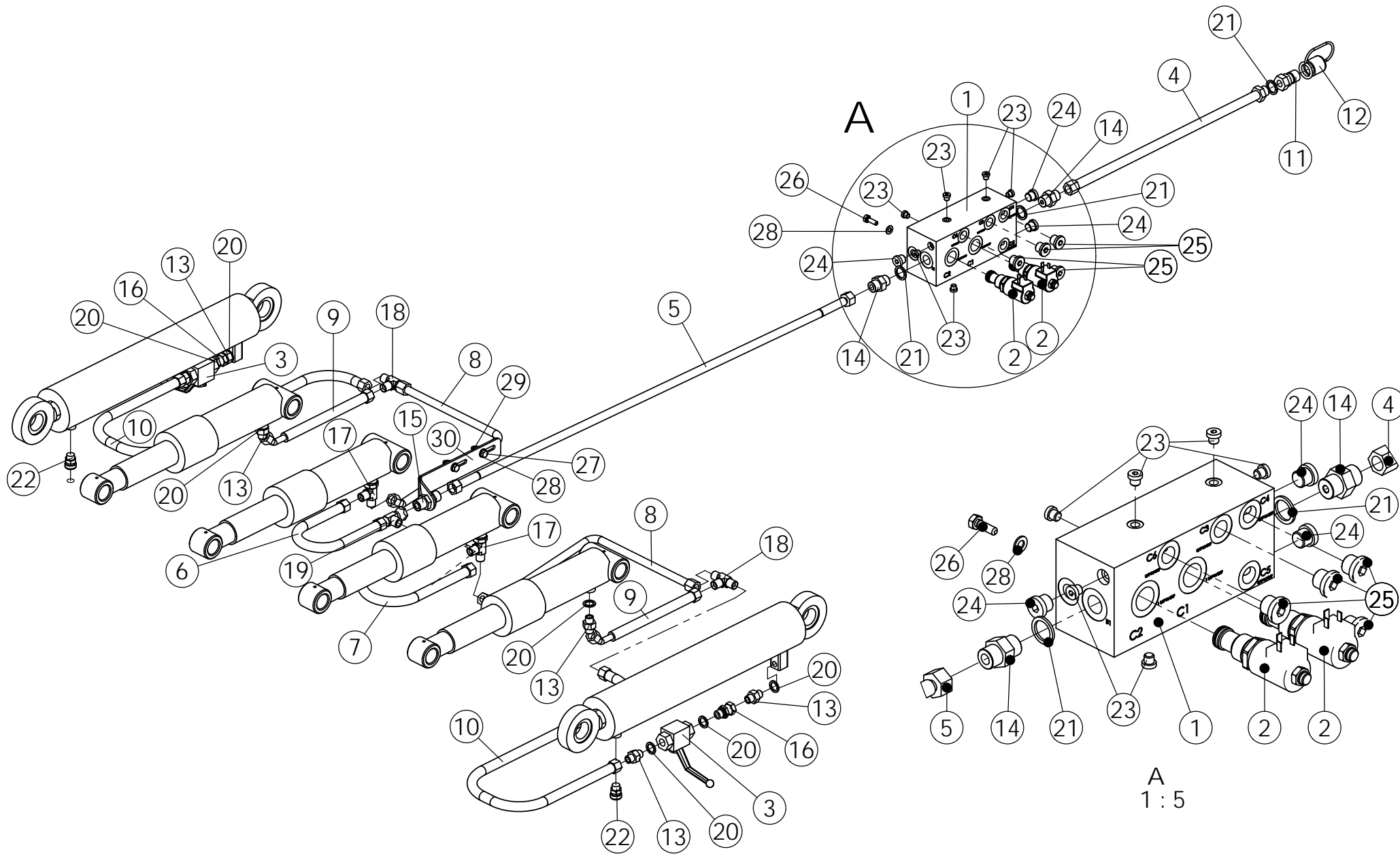
98940602 HYDRAULIIKKA 3000
