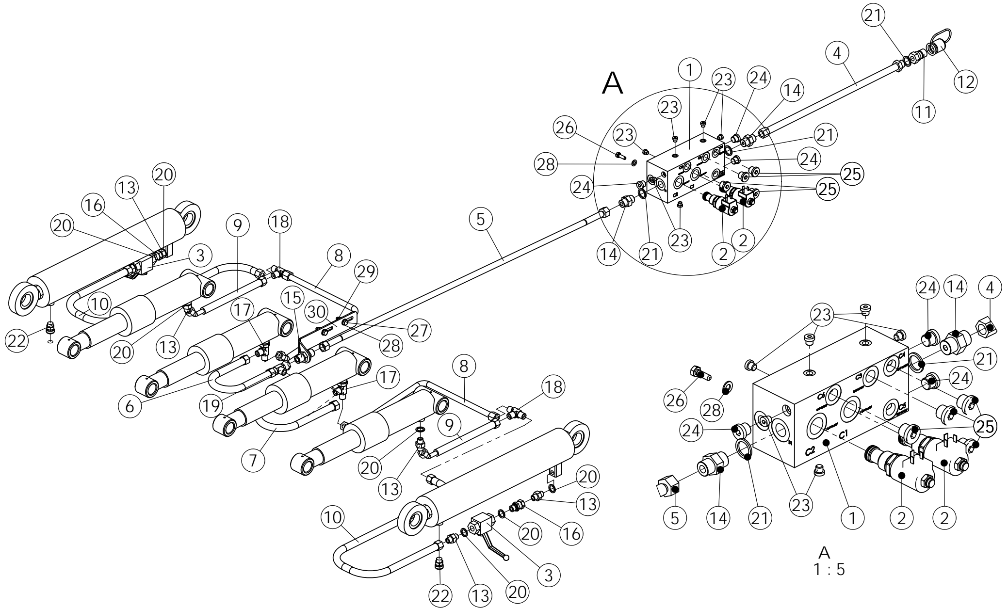
98940602 HYDRAULIIKKA 3000
