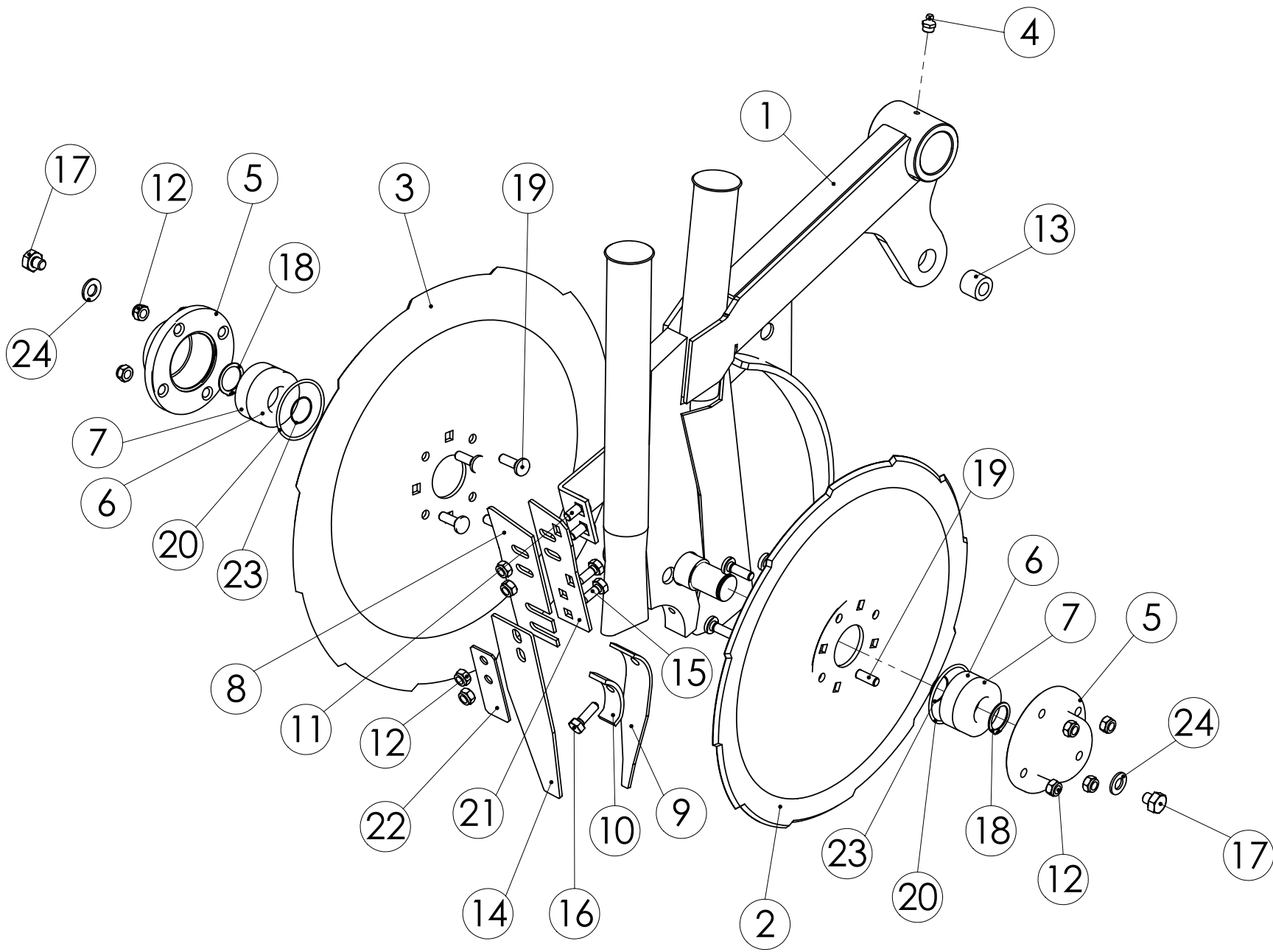
98374802 TAKAVANNAS
