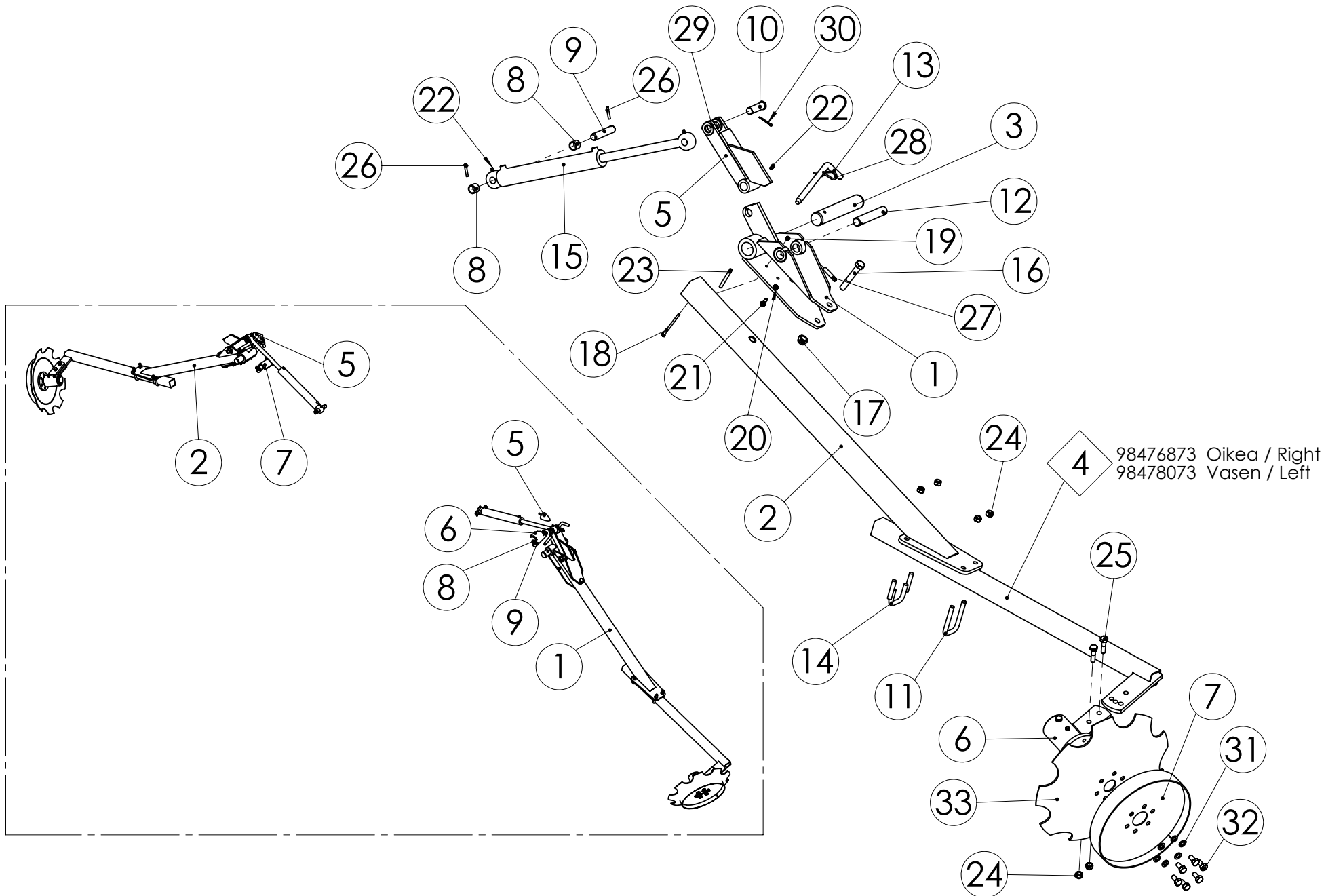
98478203 MERKITSIMET NC 3000
