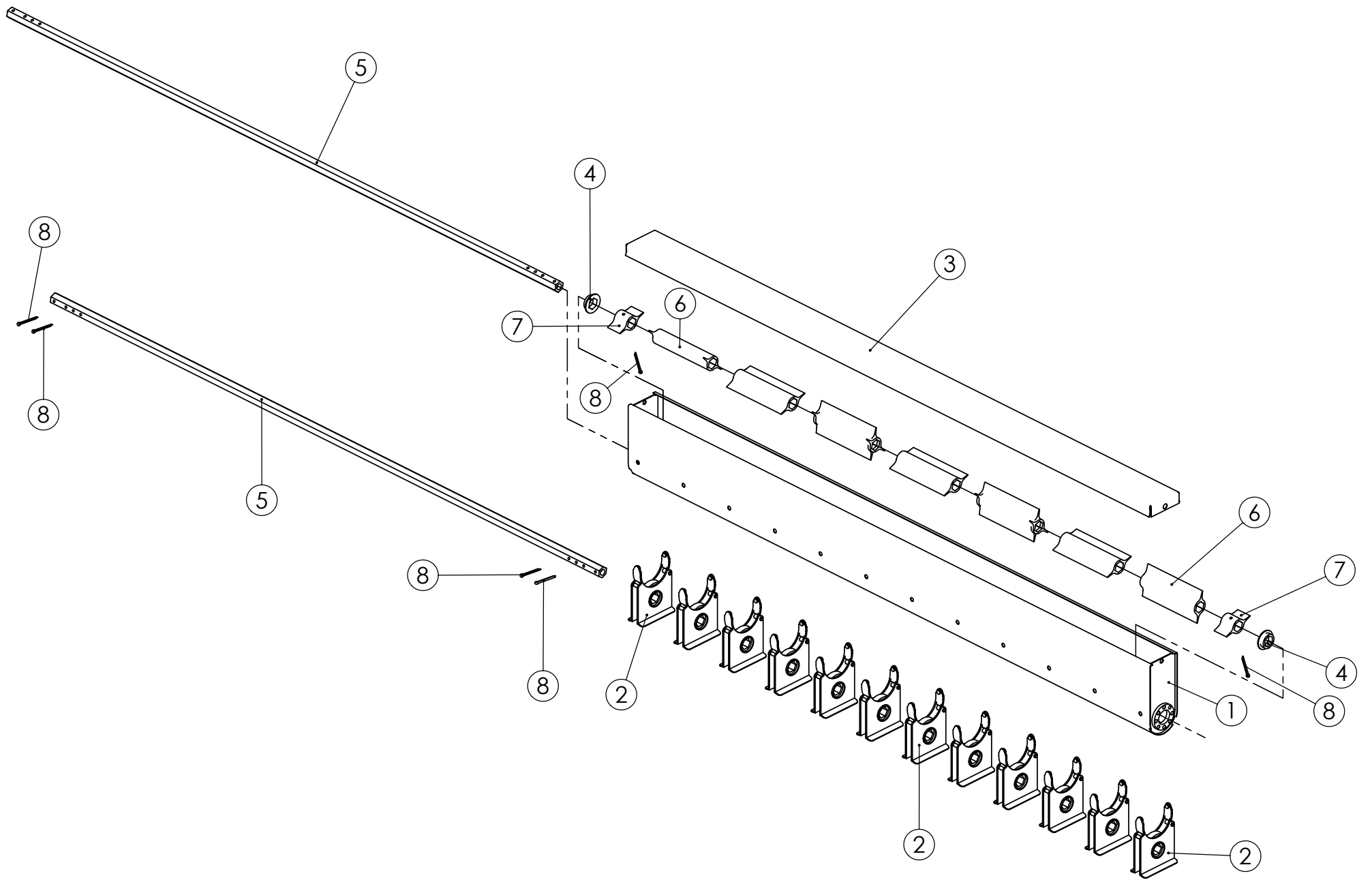
98385001 SYÖTTÖKAUKALO 3000
