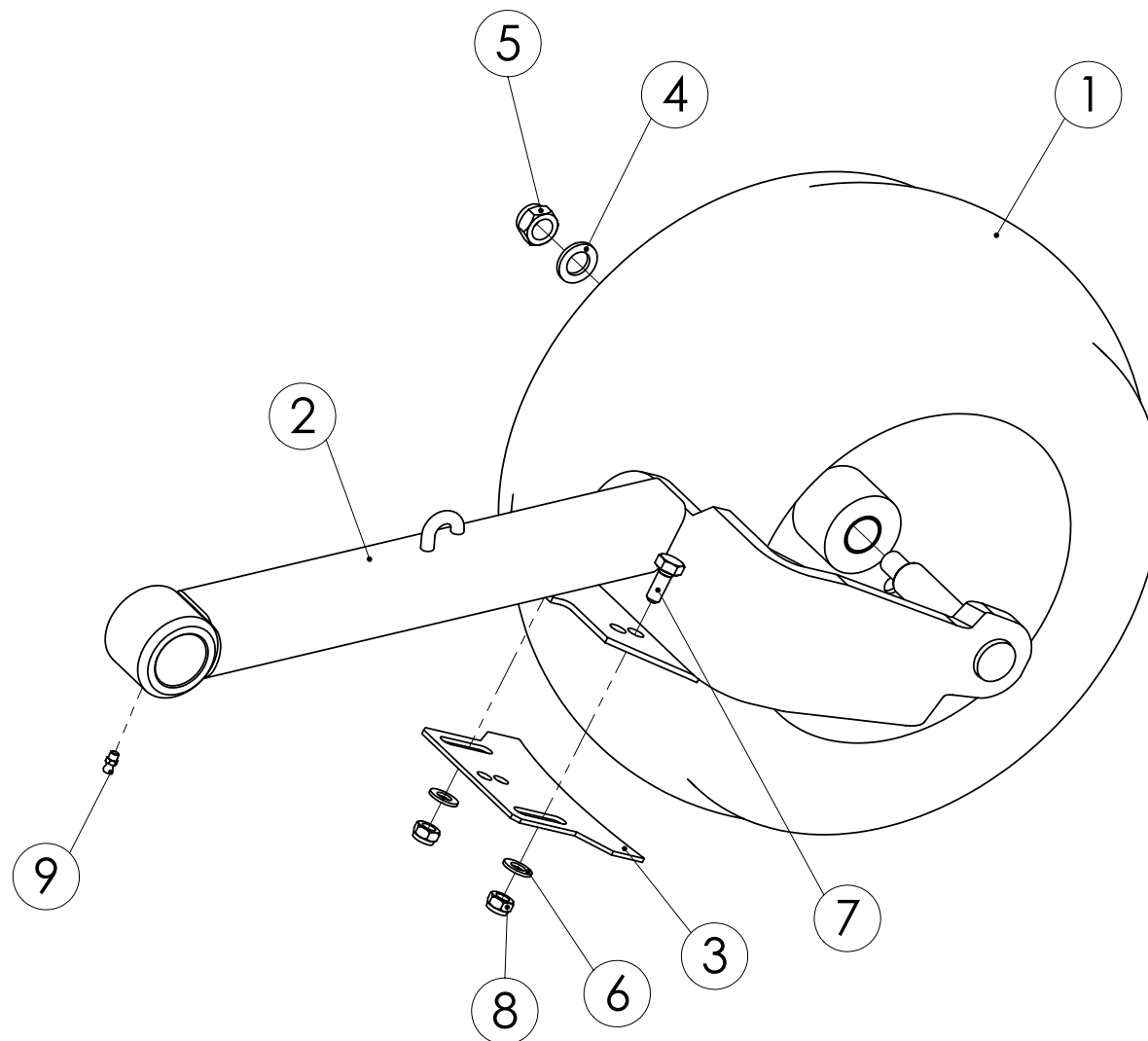
98350003 KANNATUSPYÖRÄ
