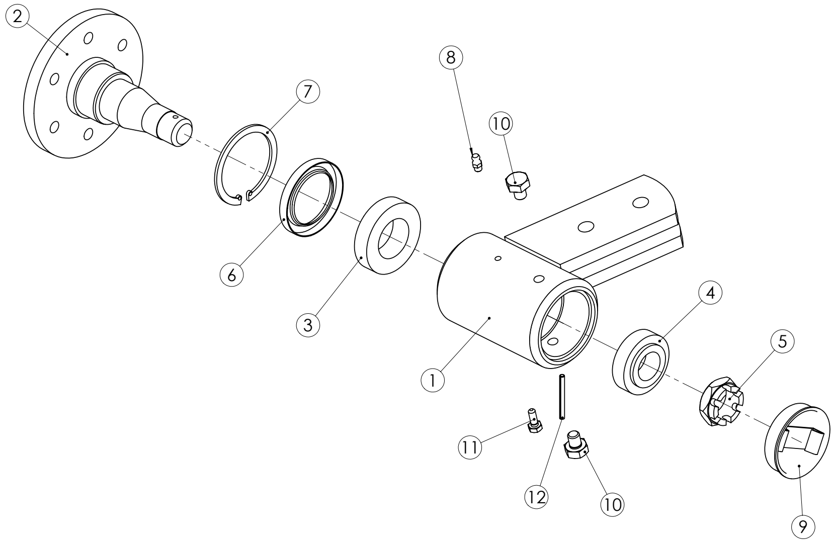
98473604 LAAKEROINTI
