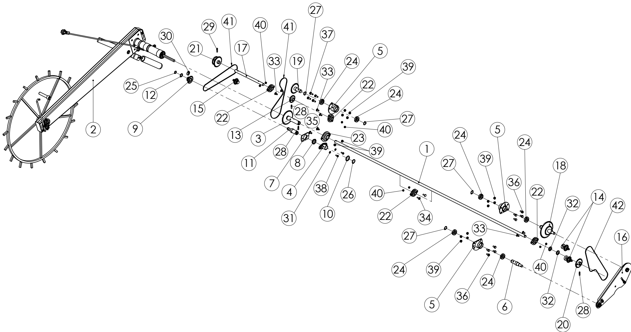
98423801 VOIMANSIIRTO 3000
