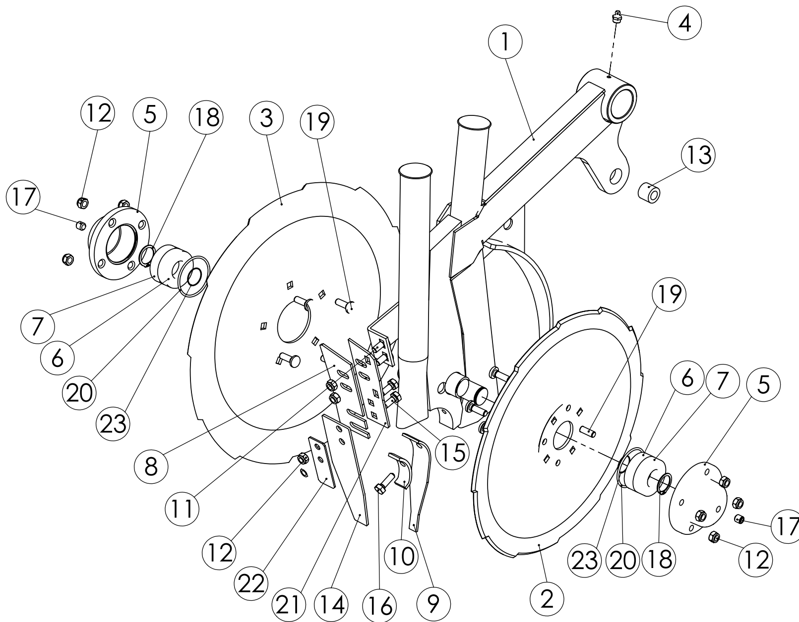
98374802 TAKAVANNAS
