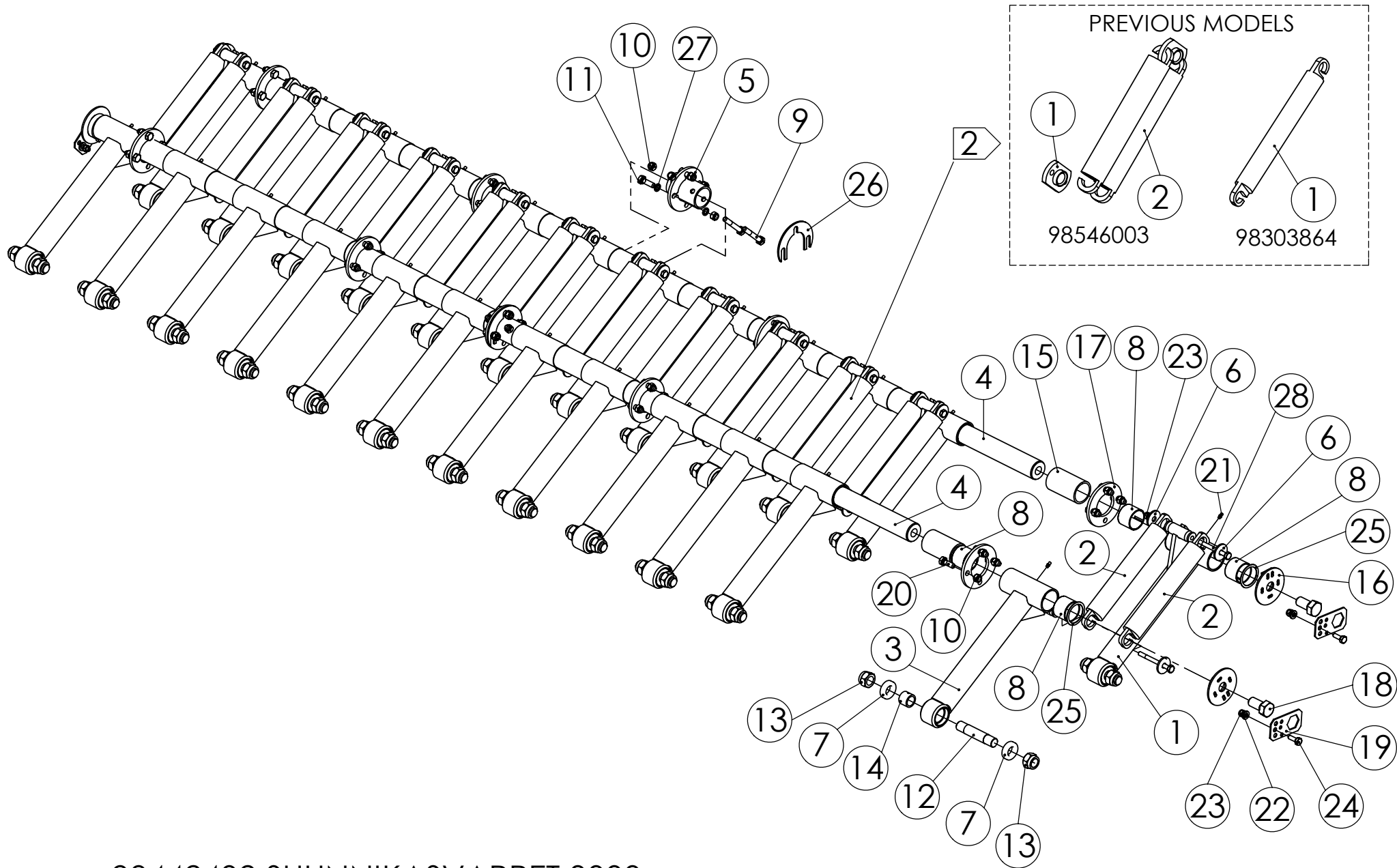
98442402 SUUNNIKASVARRET 3000
