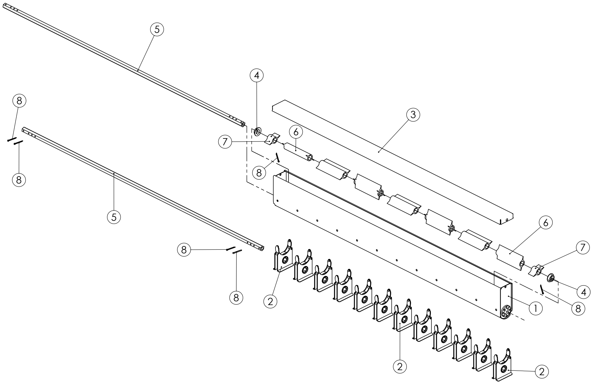
98385001 SYÖTTÖKAUKALO 3000
