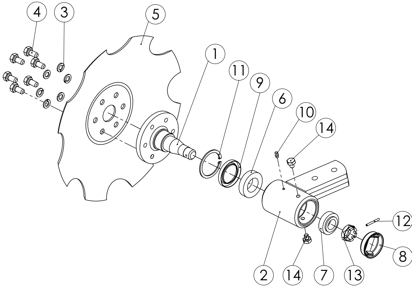
98476203 KIEKKO KP.
