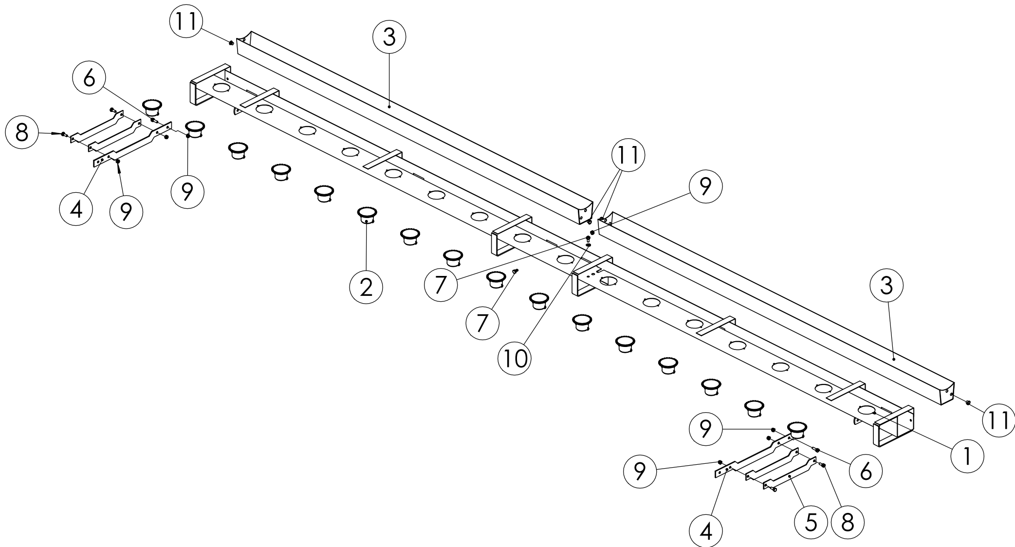
99100502 LANNOITEHYLLY JC 4000 STAR
