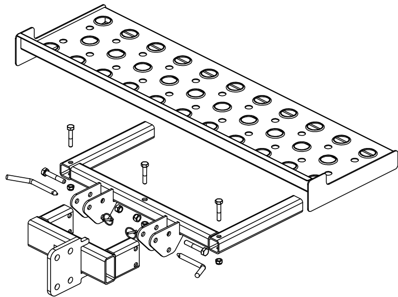
99010503 ETUASTINTASO VAS. KP.
