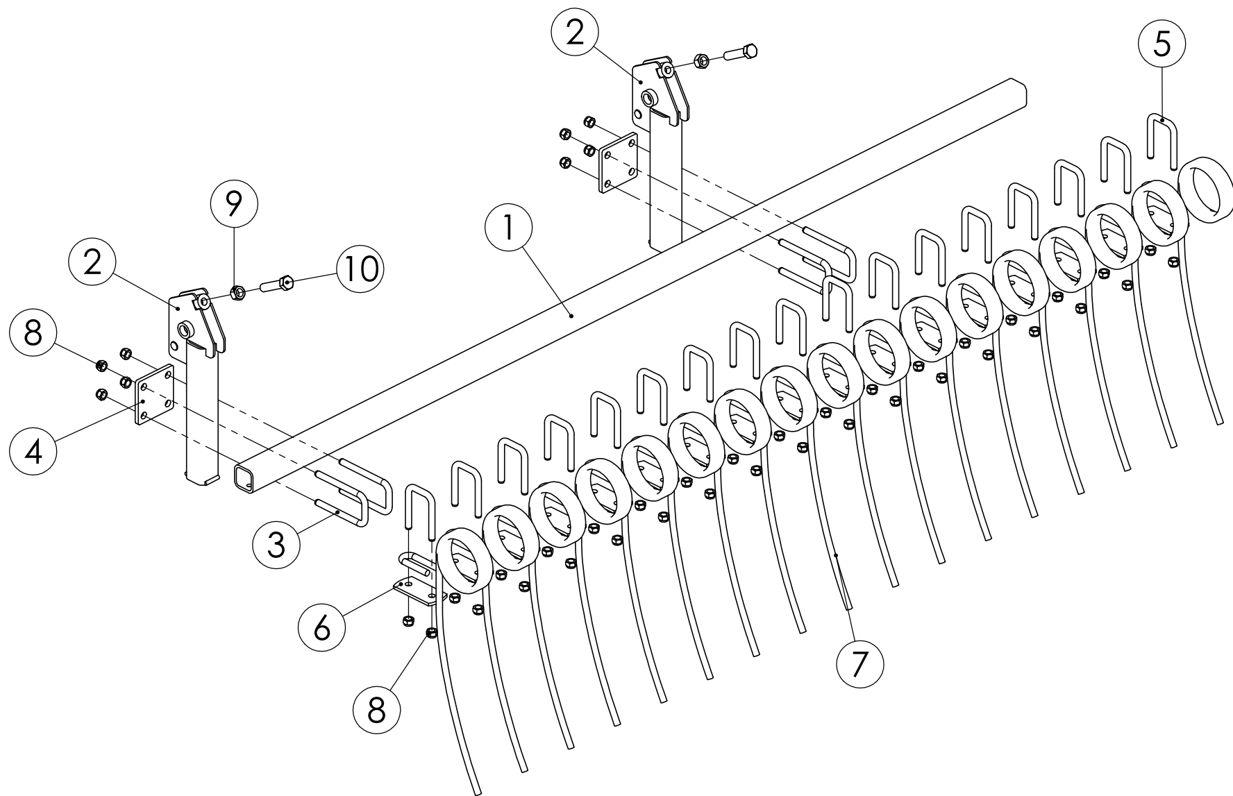
98637802 PIIKKIRUNKO, VASEN JC 4000
