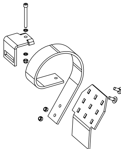
98950104 JOUSIPIIKKI KP. OIK
