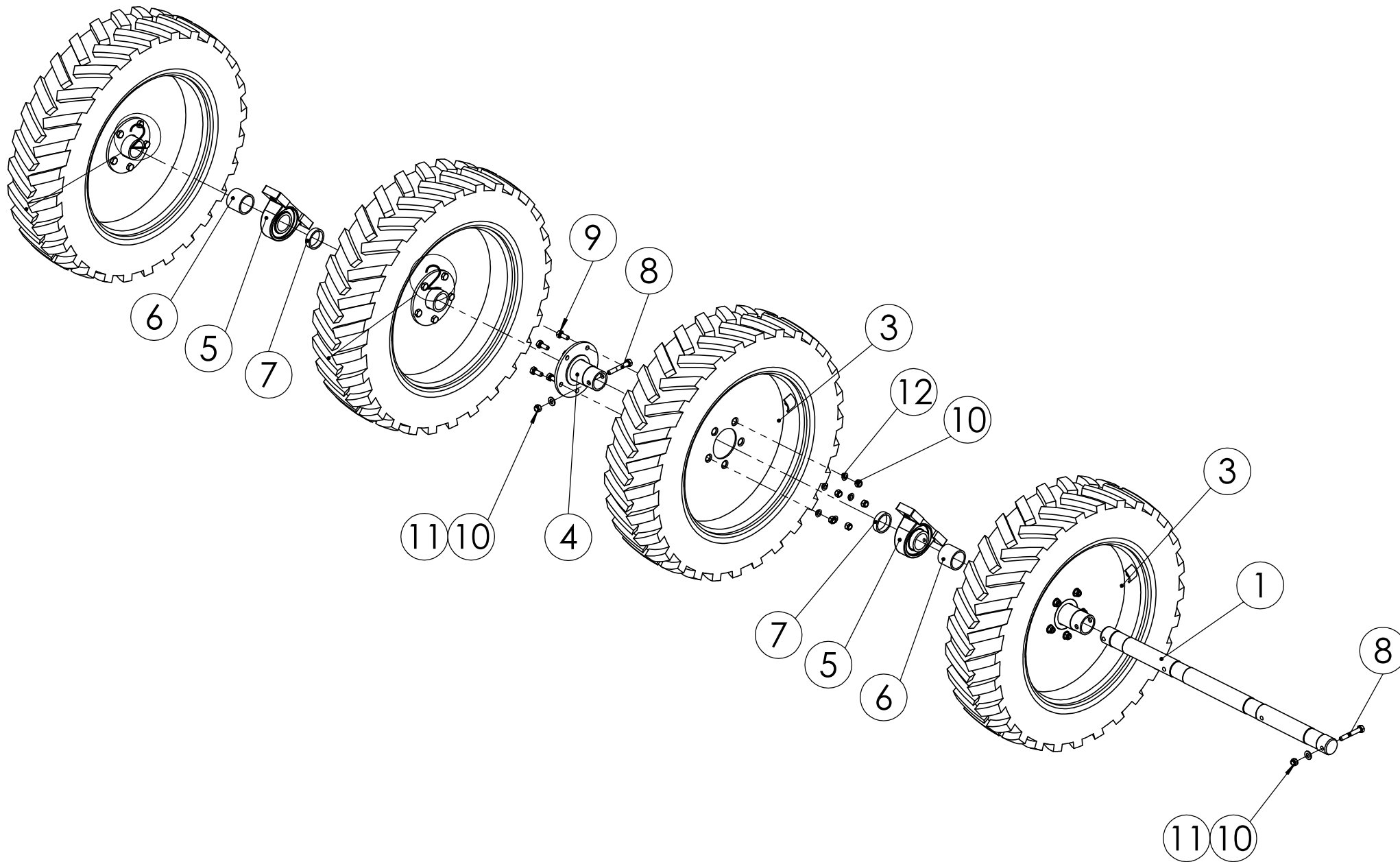
98794004 PYÖRÄPAKETTI, KESKIOSA, JC 4000
