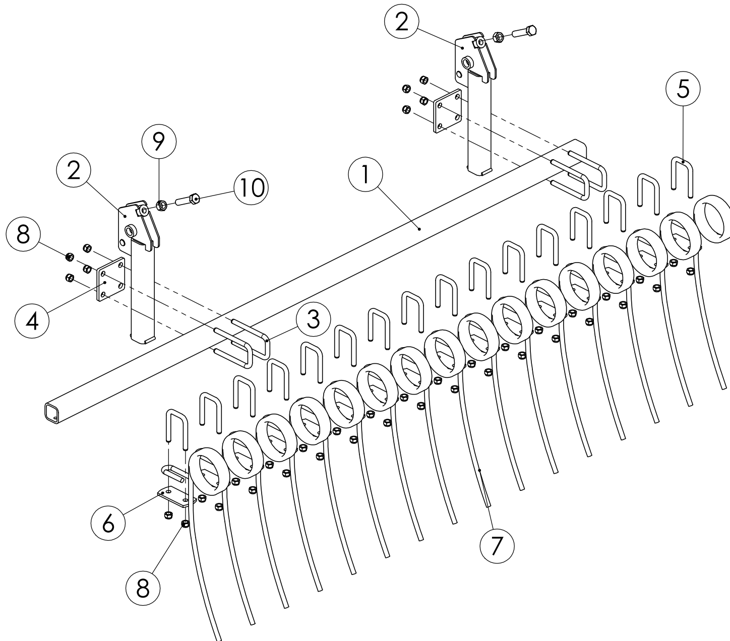
98637902 PIIKKIRUNKO OIKEA JC 4000
