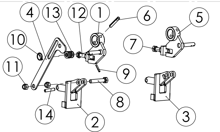
98903402 MUUTOSOSAT HYDRAULINEN JÄLKIÄES KP. JC 3000-4000 STAR
