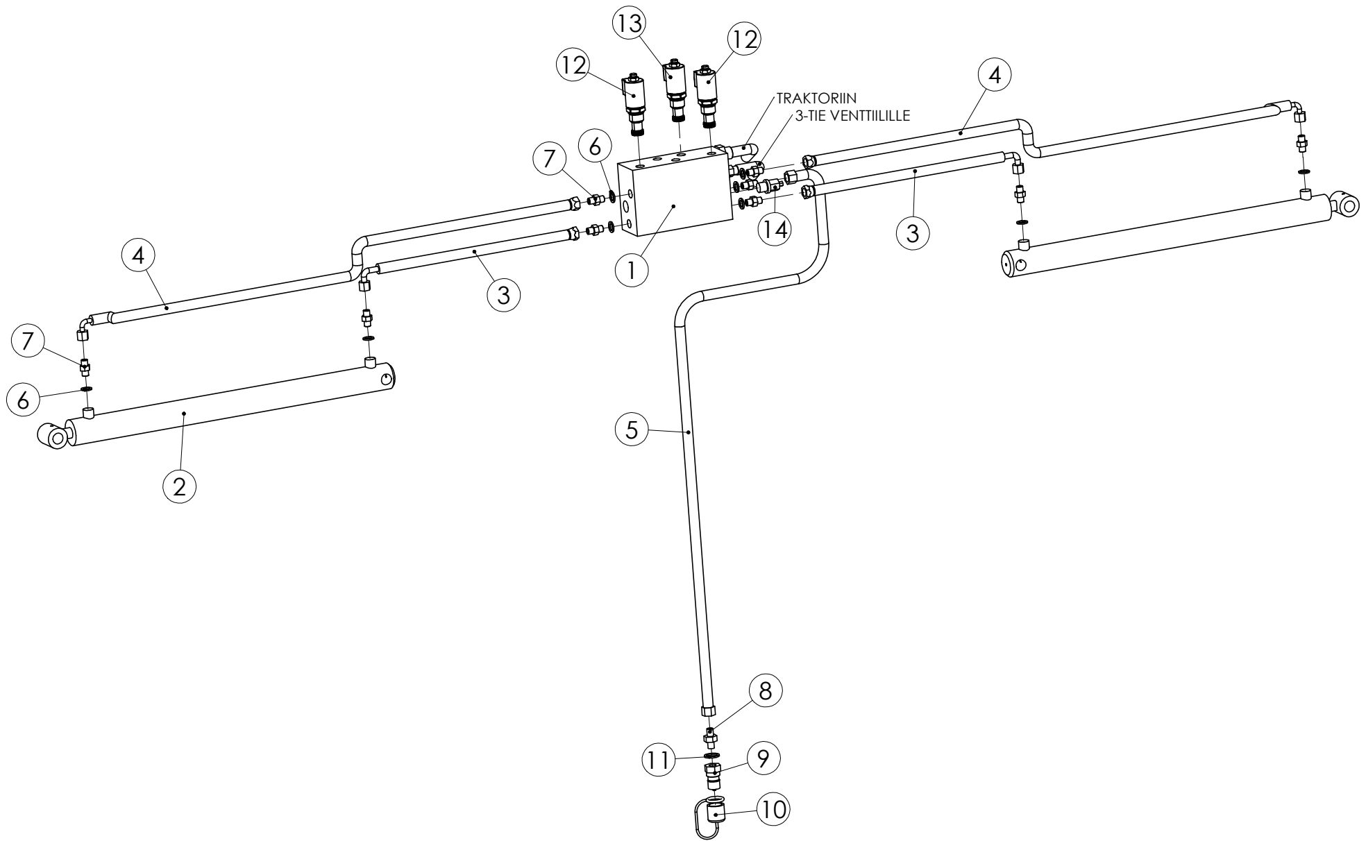
99158703 MERKKARIEN HYDR.KP JC 3000 BLOKI-VENTTIILI
