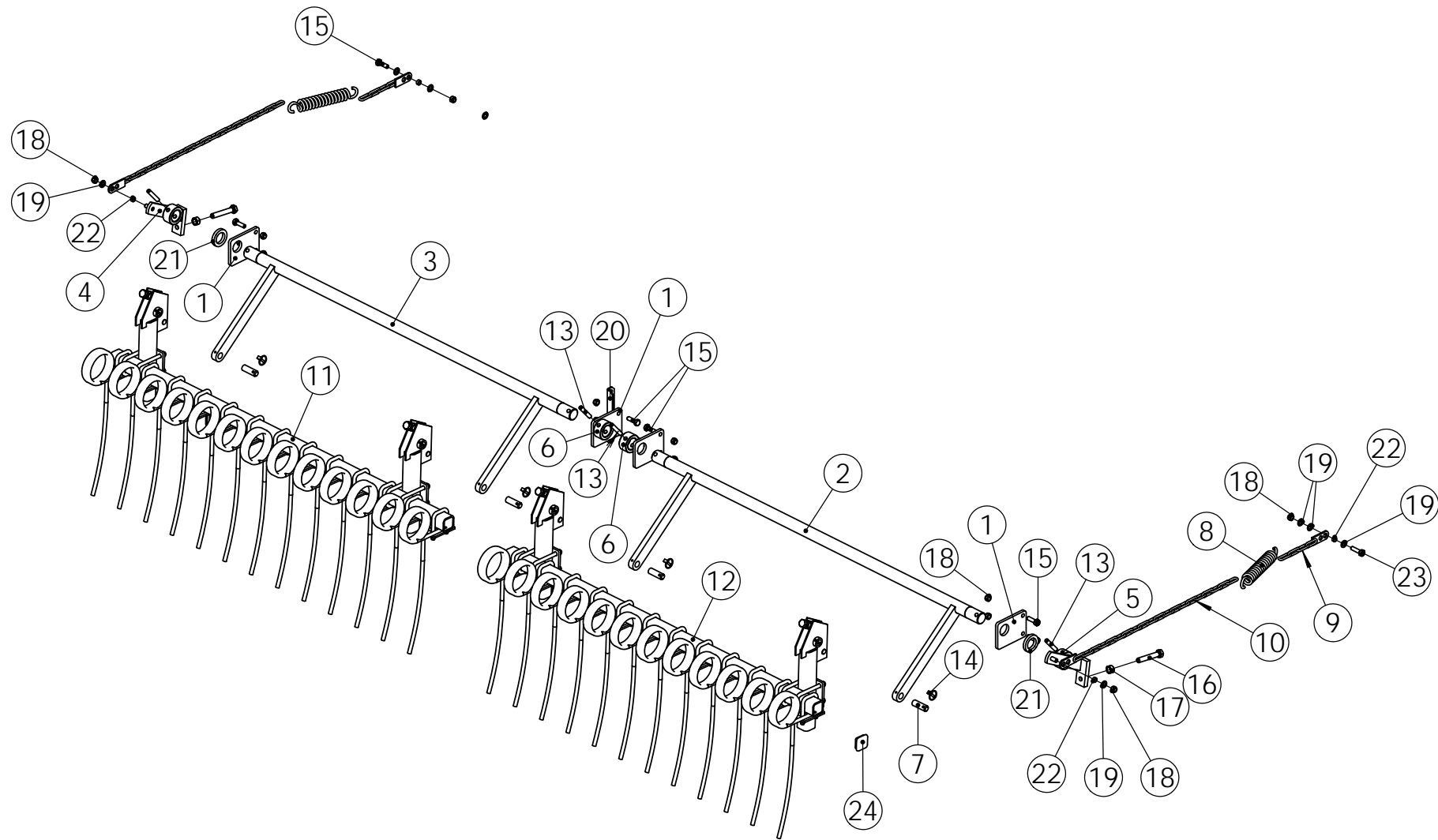
98637402 JÄLKIÄES
