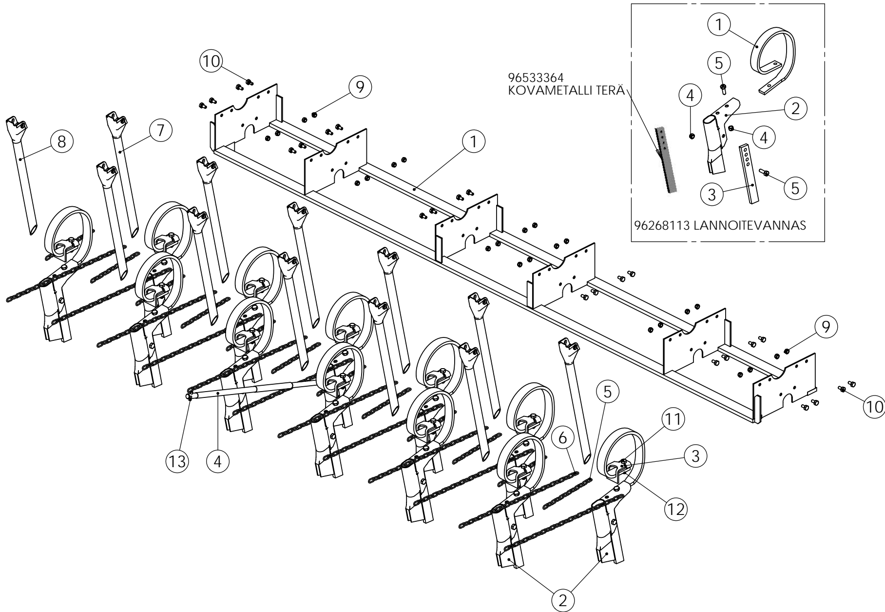
98835502 S-PIIKKIRUNKO
