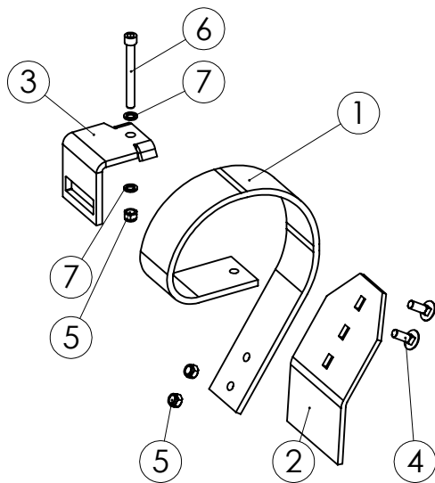
98849104 JOUSIPIIKKI KP.
