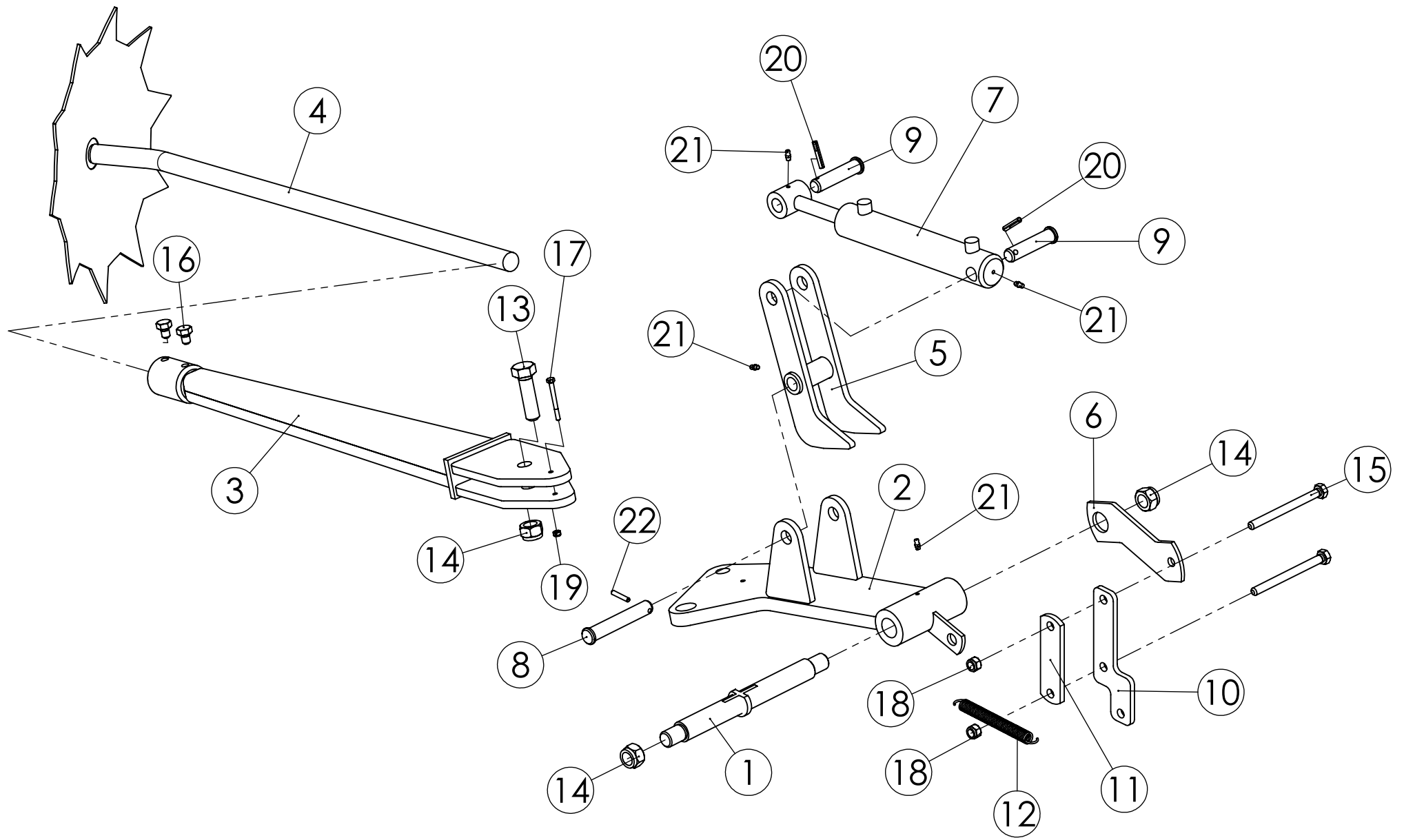
98836203 VARSISTO, VASEN
