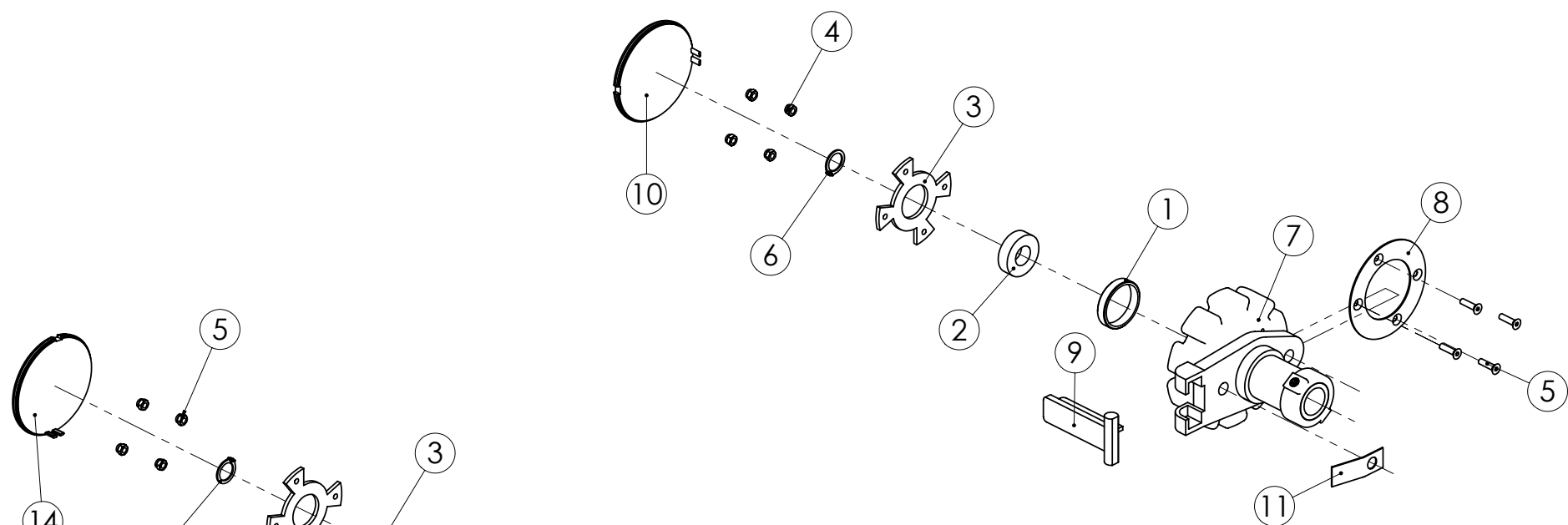
98837403 LANNOITE KÄSIPYÖRÄ
