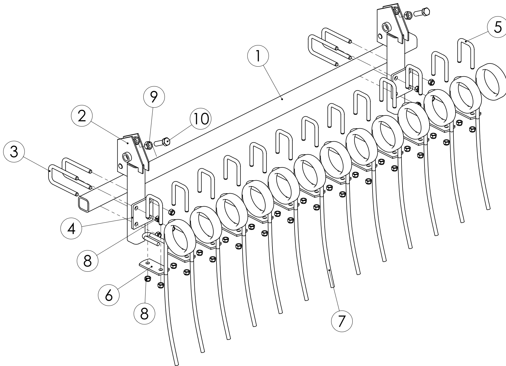
98637602 PIIKKIRUNKO, VASEN
