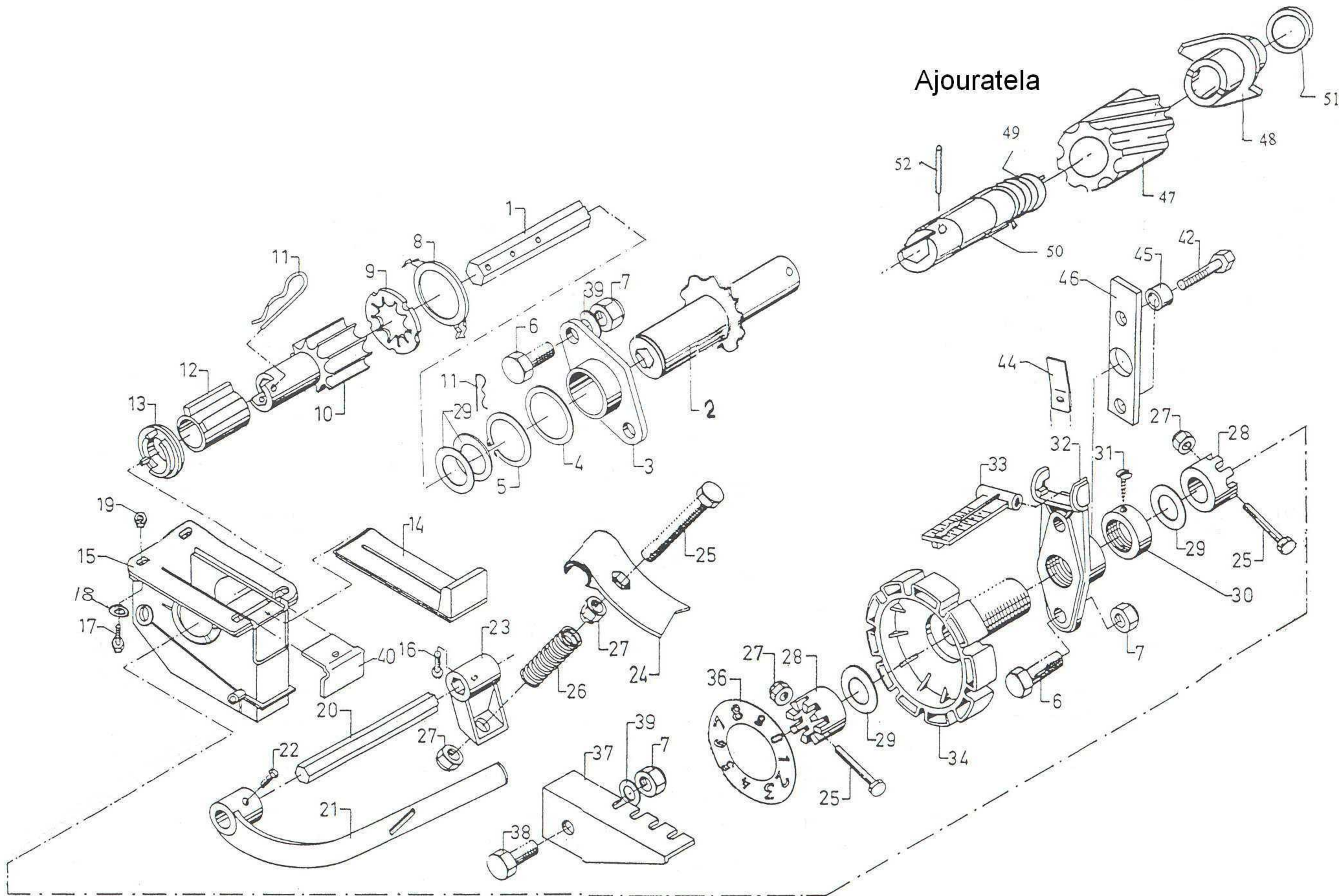
Syöttölaitteisto, siemen HKL 3000 / 4000 JC Pro
