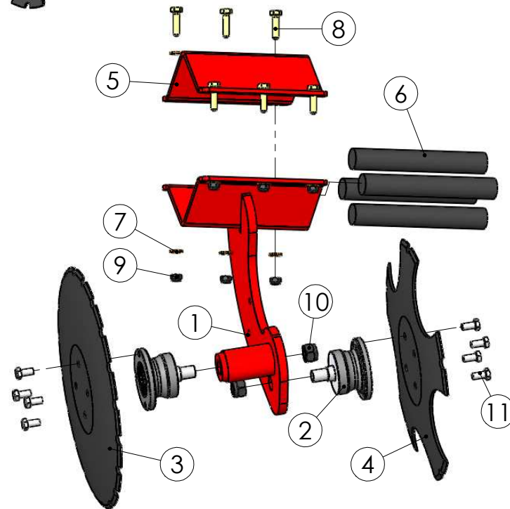
99170803 Arms left
