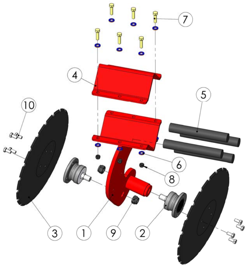
99119603 Arms left
