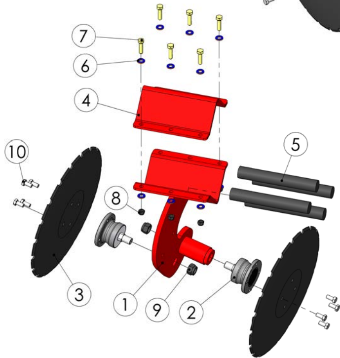
99119603 Arms left
