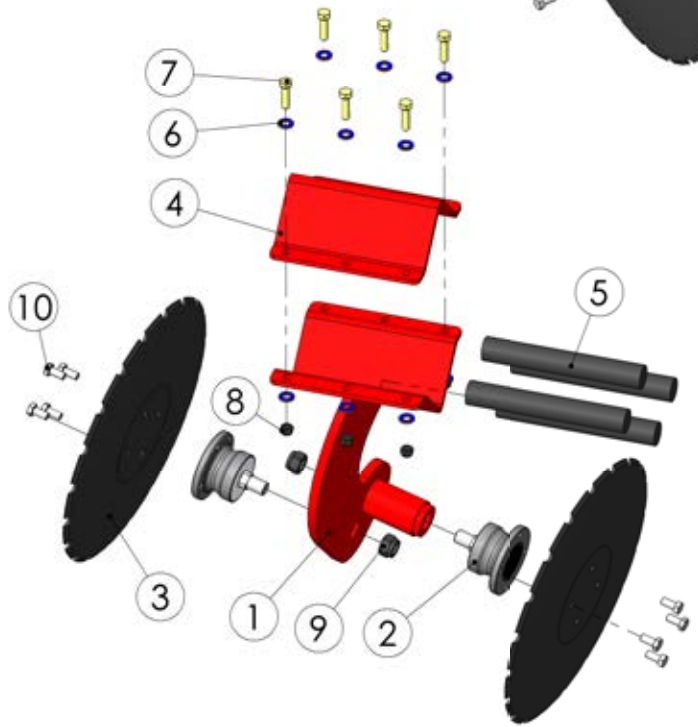
99119603 Arms left
