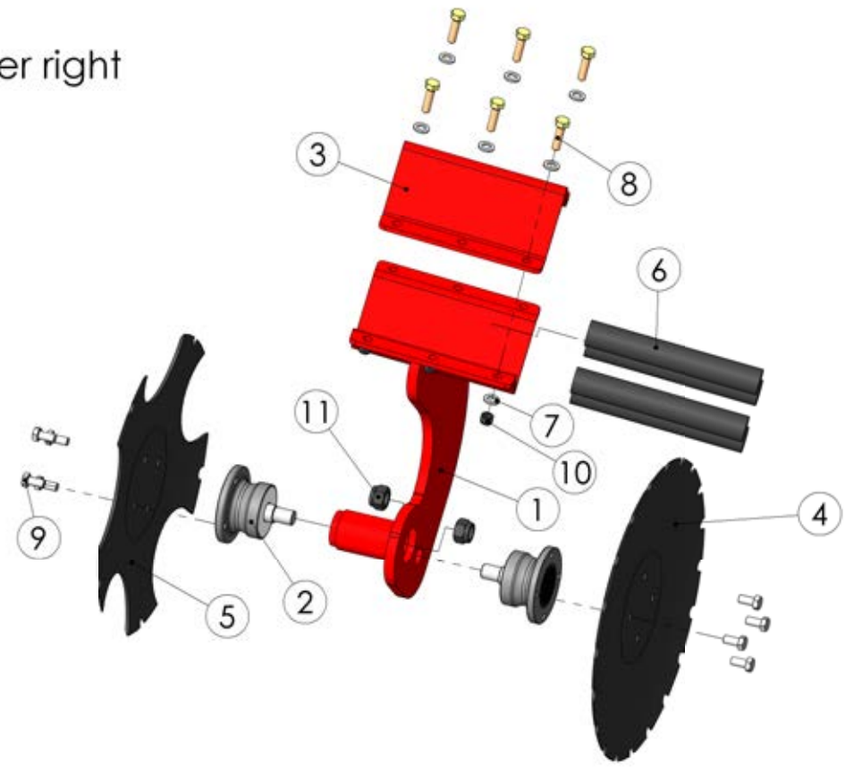
99171103 Arms left
