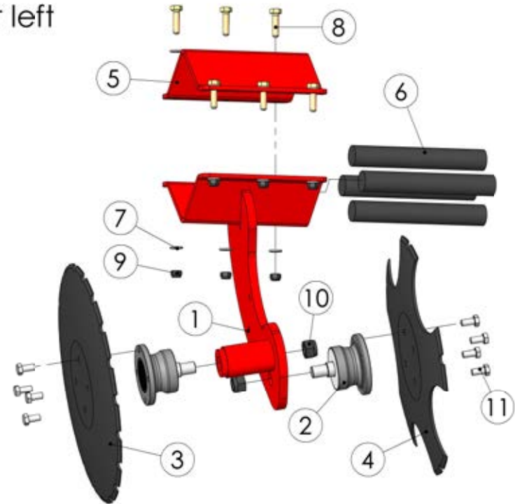
99170803 Arms left
