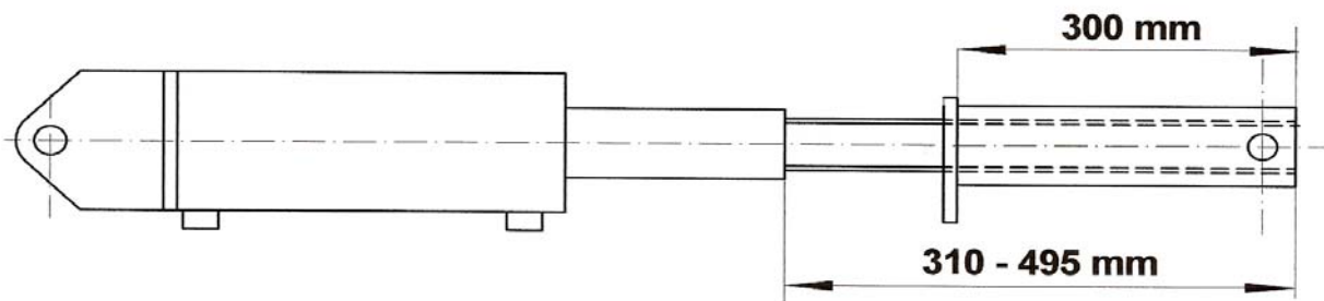
KUVA 12. Lyhyellä säätöholkilla varustetun hydraulisen työntötangon pituussäätöalue
