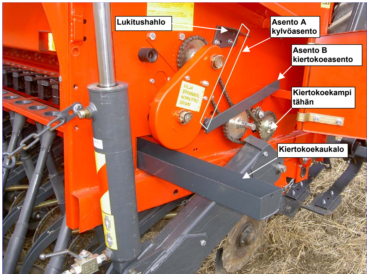
KUVA 27. Siemenpuolen kiertokoejärjestelmän käyttö
