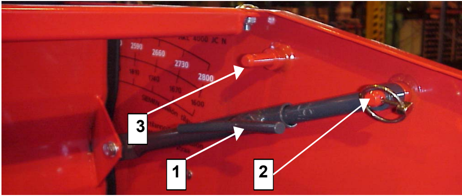
KUVA 17. Väliseinän säätötanko ja säiliöiden tilavuusasteikko
