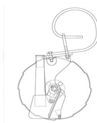
KUVA 35. Laser-lannoitevannas
