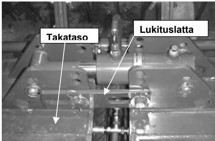
KUVA 1. Mukautumisnivelen rajoitus- ja lukituslatta
