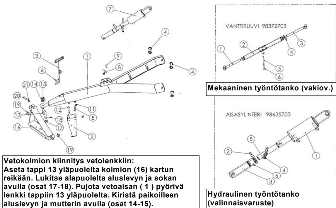
KUVA 2. Vetolaitteen kokoonpano
