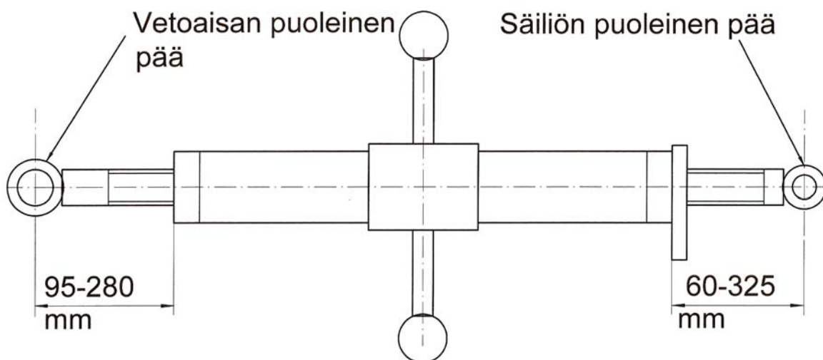
KUVA 10. Mekaanisen työntötangon pituussäätöalueet
