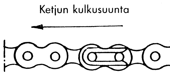
KUVA 43. Ketjulukon asennus
