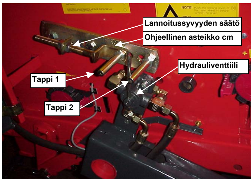
KUVA 30. Lannoitteen sijoitusyvyyden säätöventtiili
