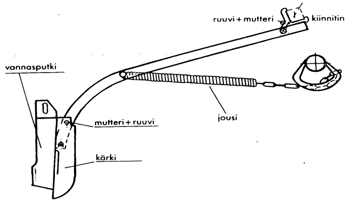
KUVA 41. Kylvövannas varsineen
