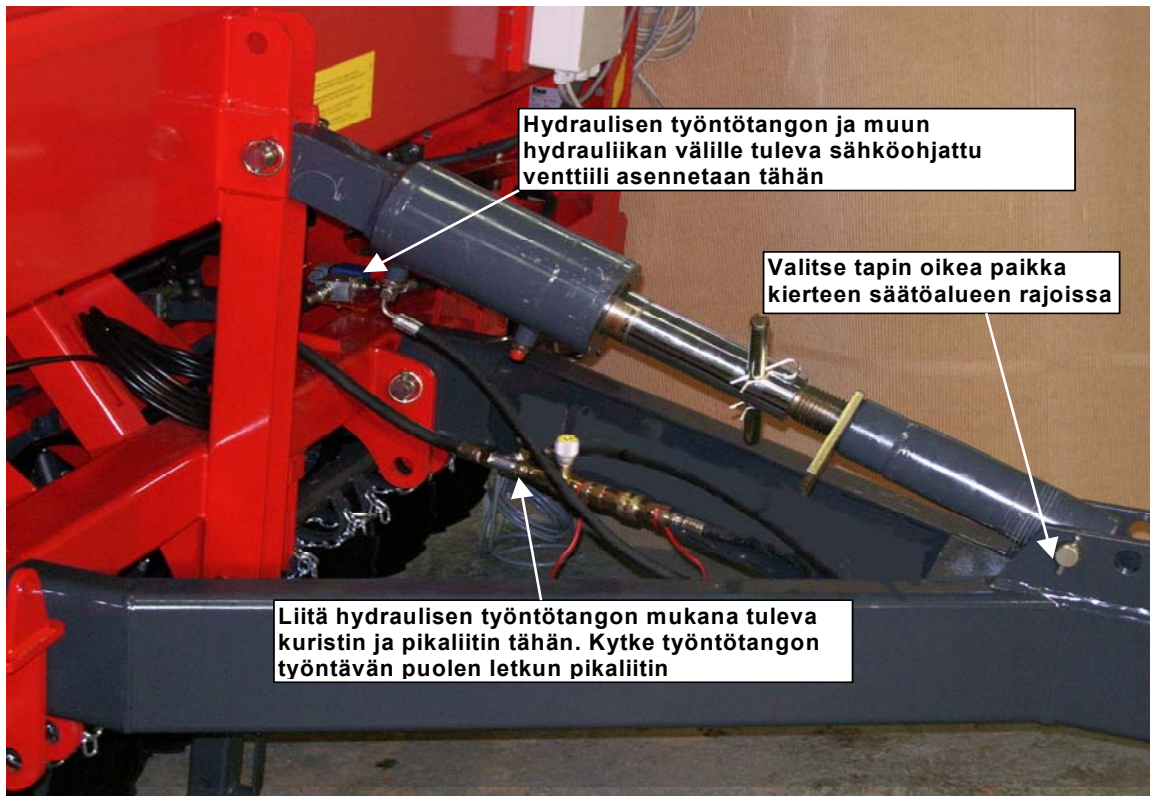
KUVA 4. Vetoaisahydrauliikan asennus
