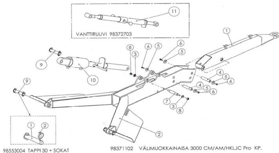
KUVA 5. Monitoimivetoaisan kokoonpano
