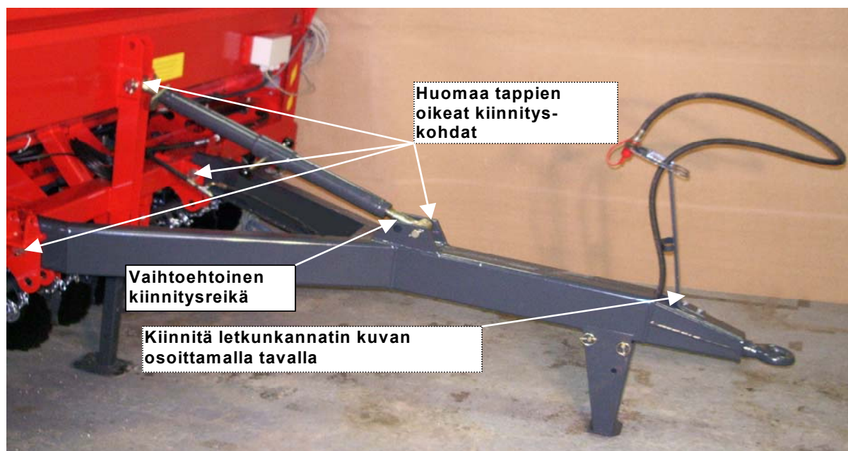
KUVA 3. Vakiovetoaisan asennus
