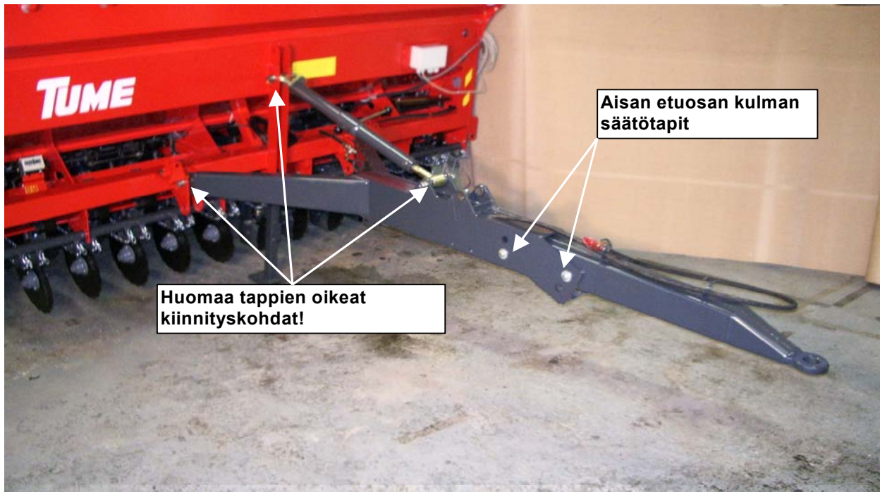
KUVA 6. Monitoimivetoaisa alavetoaisana mekaanisella työntötangolla.
