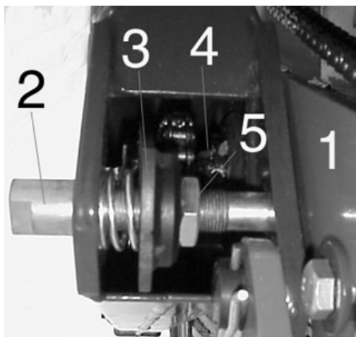
KUVA 40. Voimansiirron kytkin
