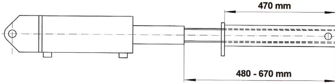
KUVA 11. Pitkällä säätöholkilla varustetun hydraulisen työntötangon pituussäätöalue
