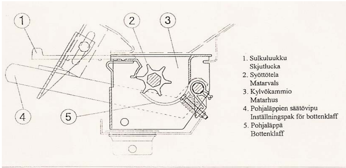
KUVA 18. Siemenen syöttölaitteen rakenne
