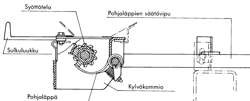
KUVA 25. Lannoitteen syöttölaite
