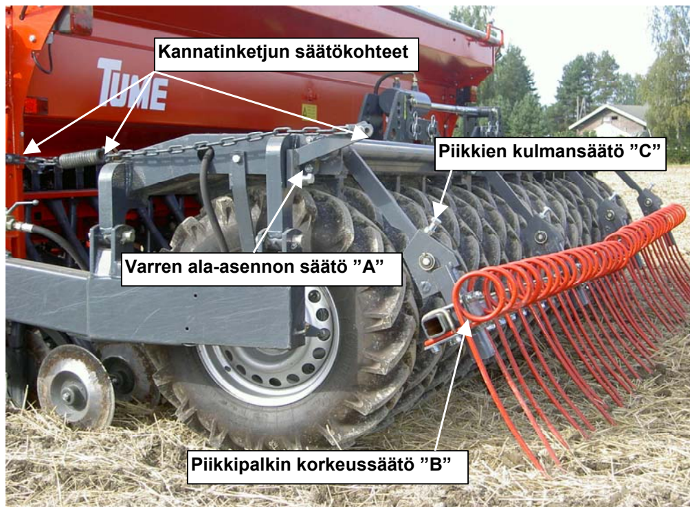
KUVA 33. Jälkiäes.
