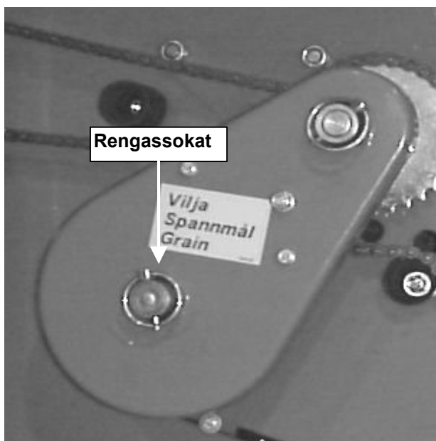
KUVA 20. Voimansiirtokasetti. I = Vilja, II = Piensiemien
