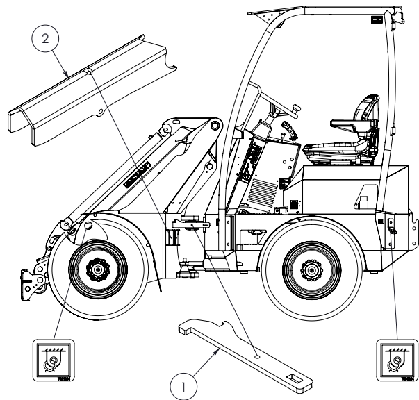
Kuva 5, kiinnityskohtat
