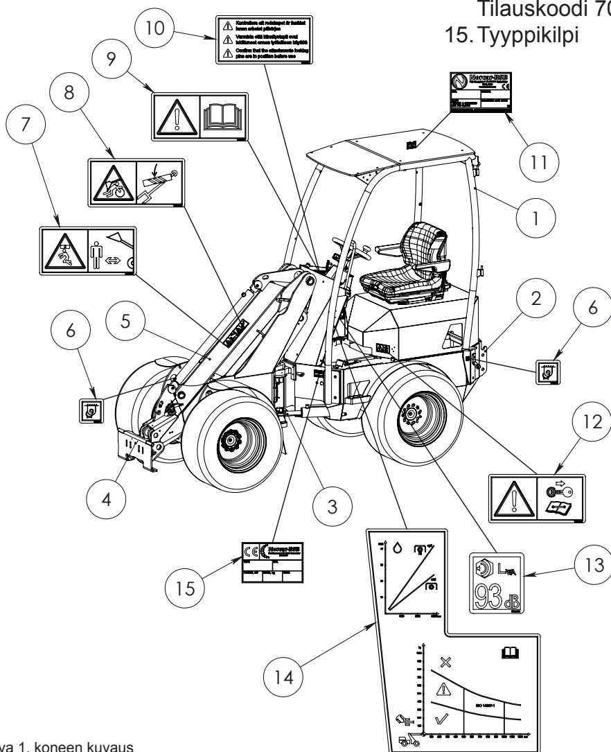
Kuva 1, koneen kuvaus
