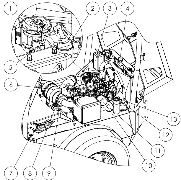
Kuva 7, huoltokohtat
