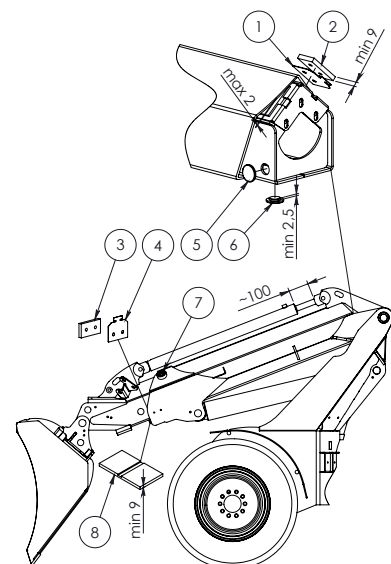
Kuva 8, nostopuomin tarkastus.
