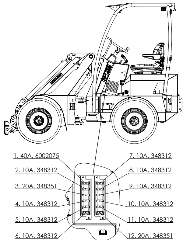
Kuva 9, sulakkeet
