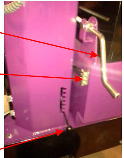
Valssivällyksen säätökampiu
