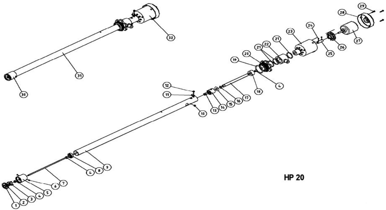
Varaosakuva nro 11 Partspicture No 11 Pumppu Pump
