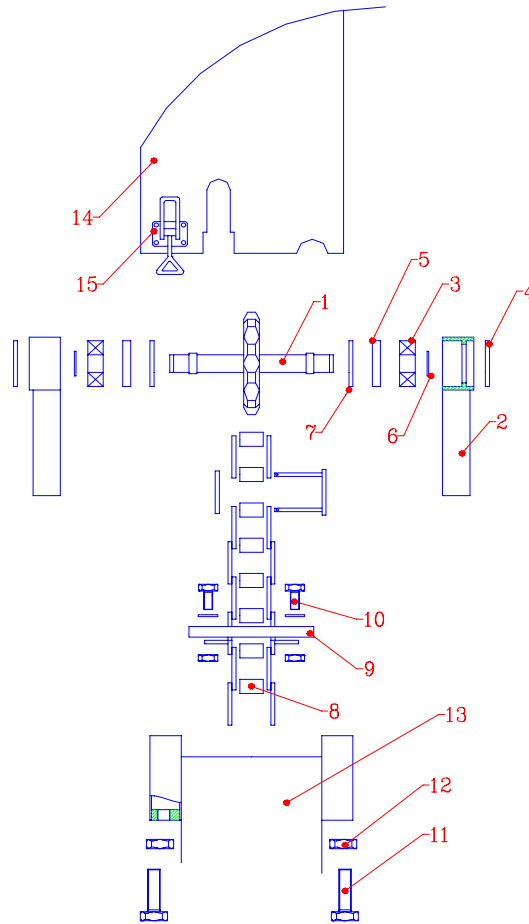
Varaosakuva nro 2 Kirstystyspyörä
