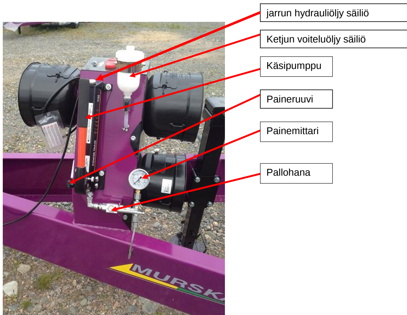
Kuva. Baggerin jarrut
