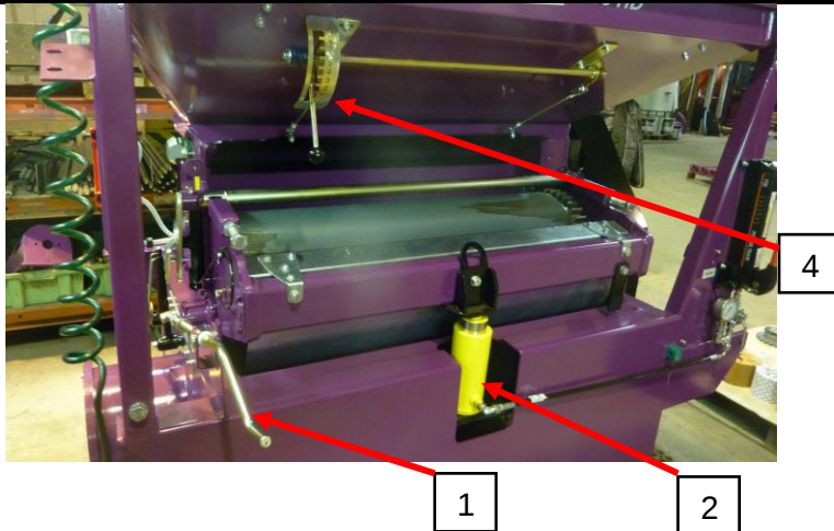
Kuva. Valssien säätäminen Osaluettelo:
