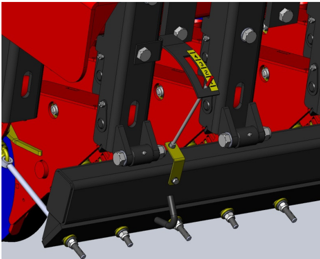
Kuva 3.2.3 Vantaan jousivoiman säätö ja viisari.
