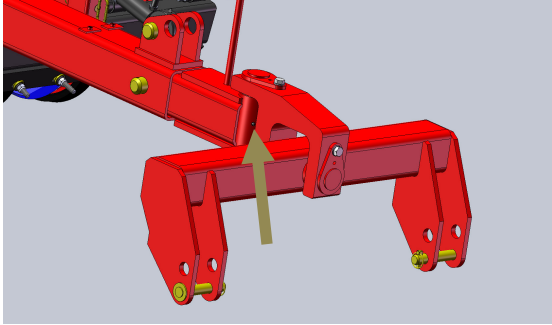
Kuva 5.8 Vetolaitteen nivel.
