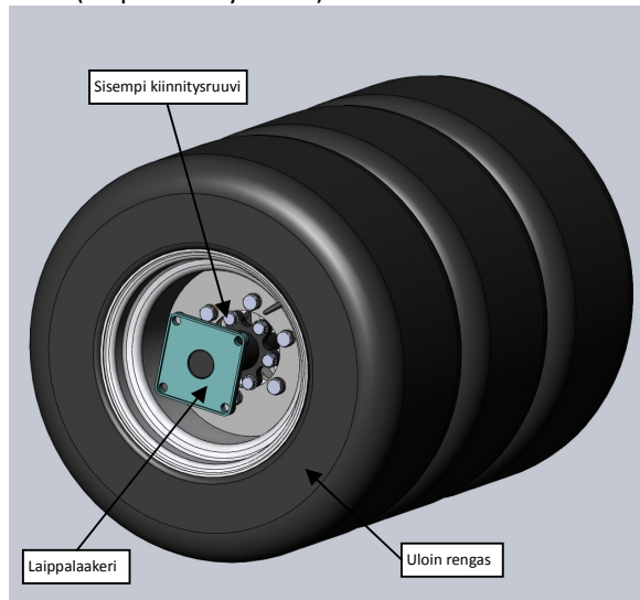
Kuva 5.14 Keskipaketin purku.
