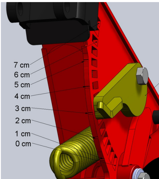
Kuva 3.2.2 Syvyydensäädön lovet.
