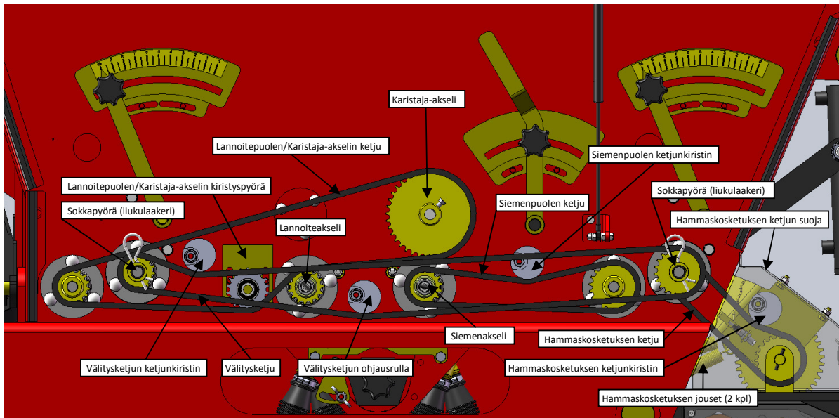
Kuva 5.2 Voimansiirron ketjut.
