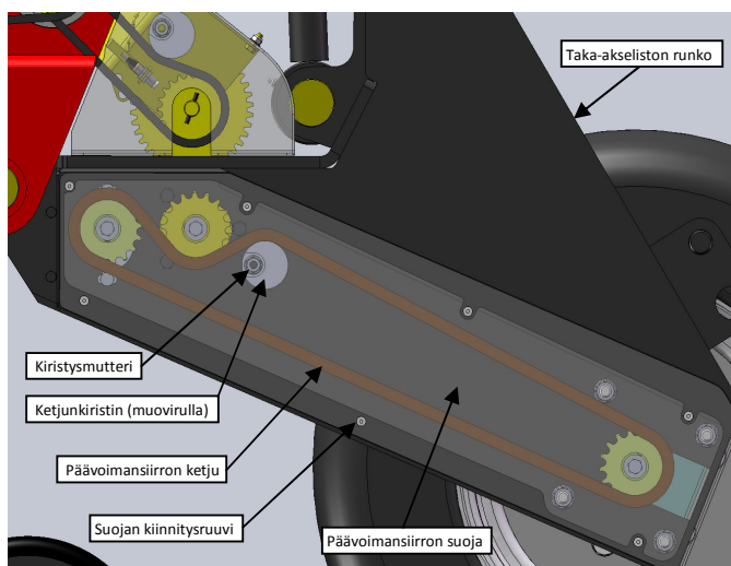
Kuva 5.1 Päävoimansiirron ketju.
