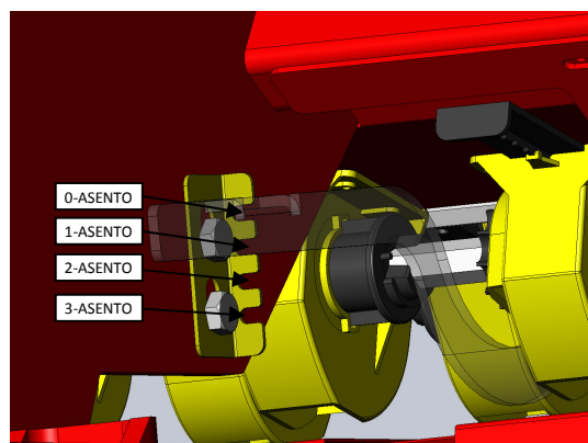
Kuva 3.4.2 Säätövivun loviasteikko.
