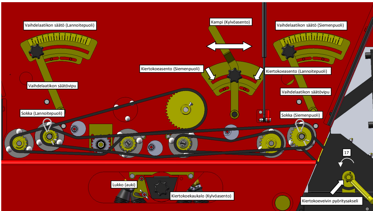
Kuva 3.3.3 Kiertokokeen tekeminen.
