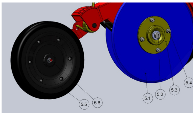
Kuva 5.11 Kiekkovannas ja peittopyörä.
