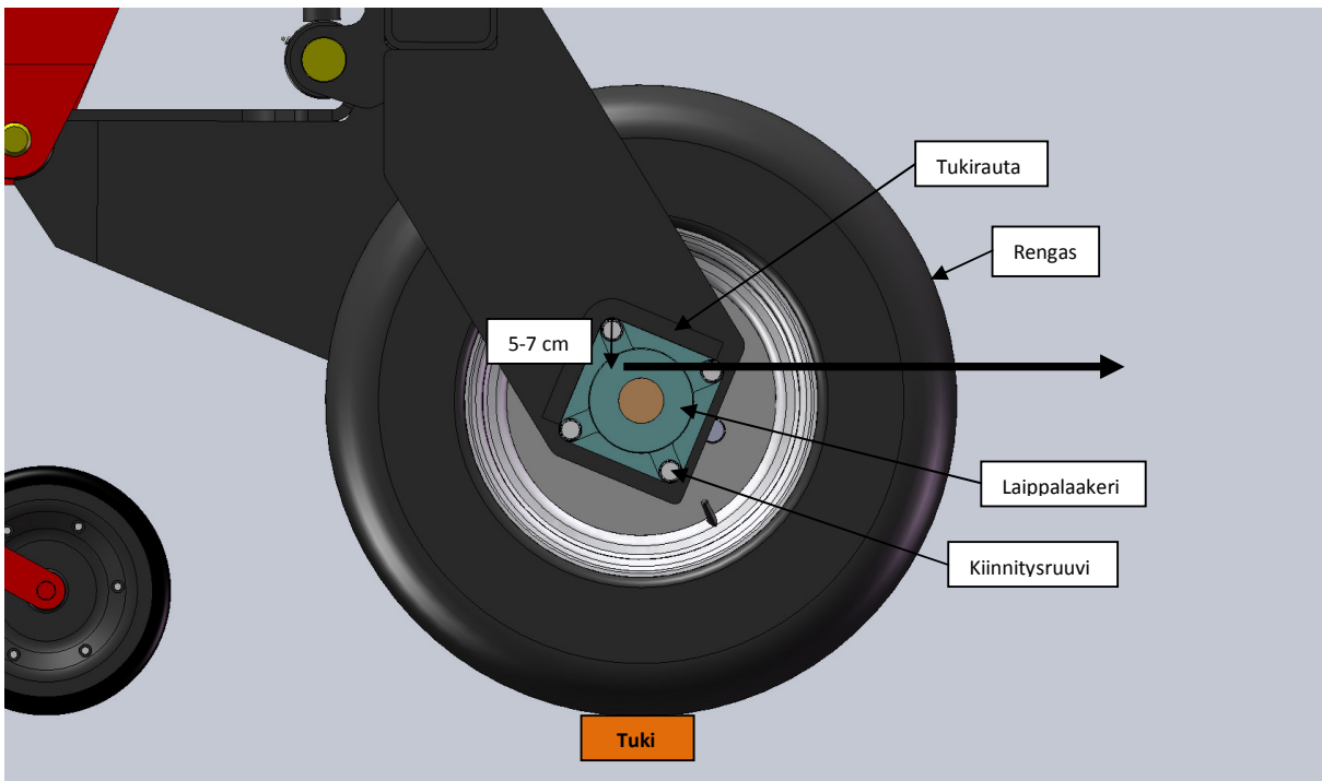
Kuva 5.12 Rengaspaketin irrotus.
