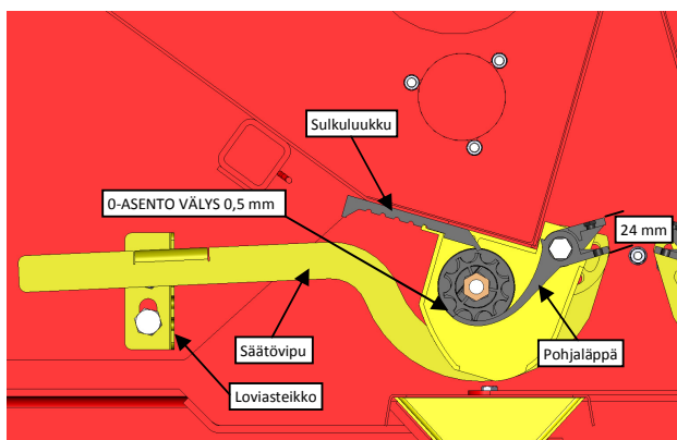
Kuva 3.4.1 Pohjaläpän säätö.
