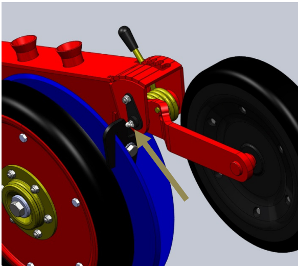
Kuva 5.5 Peittopyörän nivelholkki.
