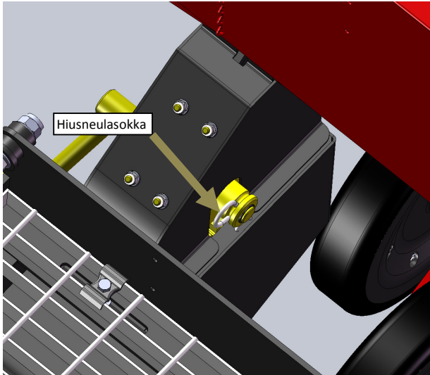
Kuva 3.3.1 Voimansiirron vapautus.
