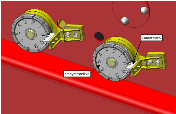
Kuva 3.3.4 Ruuvityyppiset säätöpyörät.
