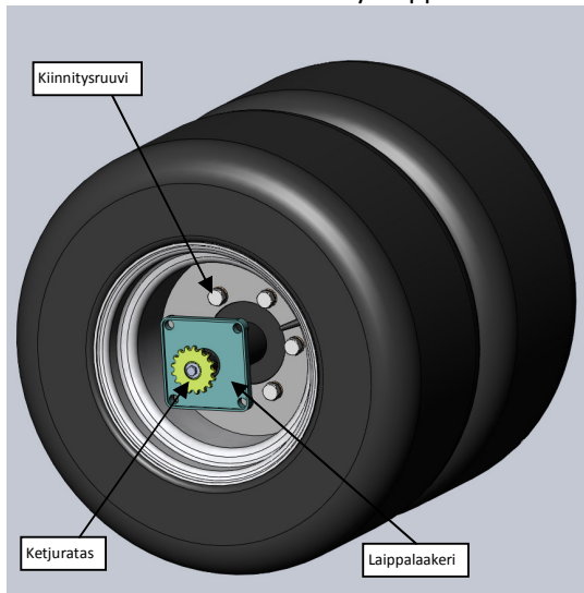
Kuva 5.13 Rengaspaketin (vasen) purku.
