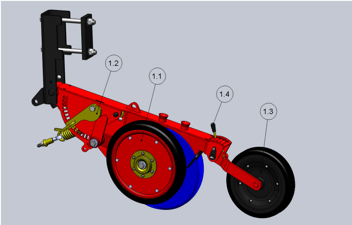
Kuva 3.2.1 Tarkkuusvannas.
