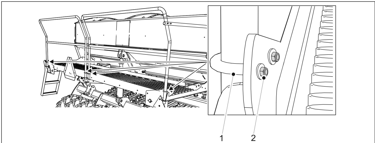
Kuva. 7.1.2.5. - 178. Hoitotason U-pultit
