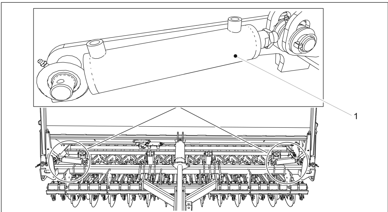
Kuva. 7.2.8. - 204. Keskimerkkarisylinterit
