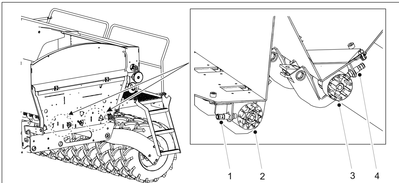
Kuva. 4.2.1.4. - 17. Pyörintävahdit
