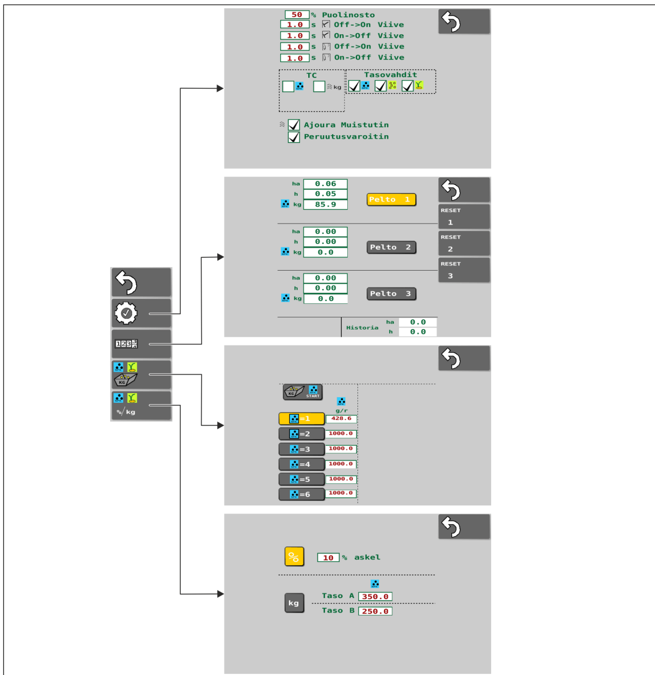
Kuva. 4.2.3. - 36. Kylvöasetukset
