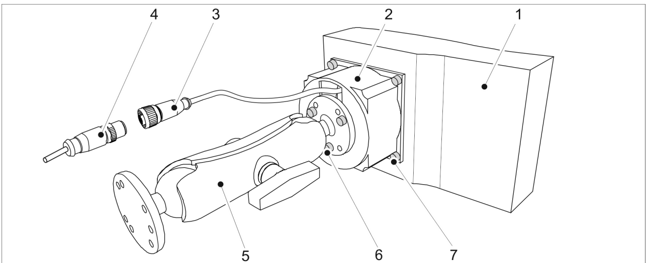
Kuva. 5.2.2. - 74. SeedPilot-ohjauspaneelin asentaminen
