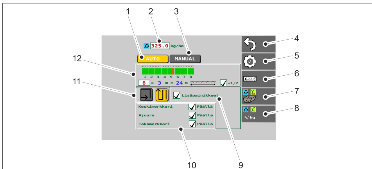
Kuva. 4.2.4.1. - 45. Kylväasetukset-sivun painikkeet
