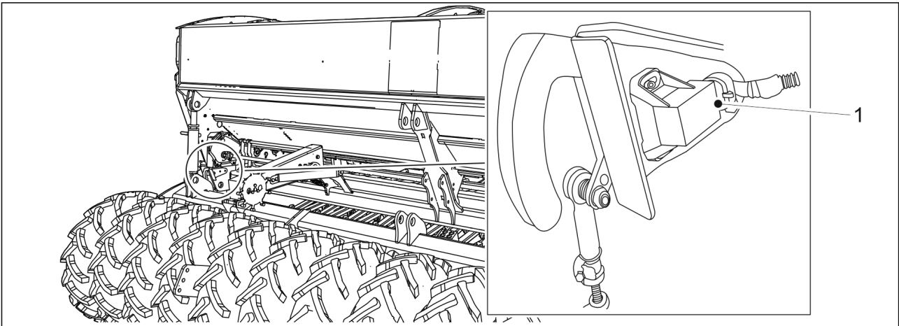
Kuva. 4.2.1.2. - 15. Kylvöasentoanturi
