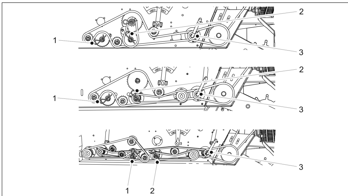
Kuva. 6.8.7. - 159. Piensiemensäiliön kiertokoe. Ylhäällä kone, jossa ei ole vaihdelaatikkoa, keskellä kone, jossa on vaihdelaatikko siemenpuolelle ja alhaalla kone, jossa on tuplavaihteisto.
