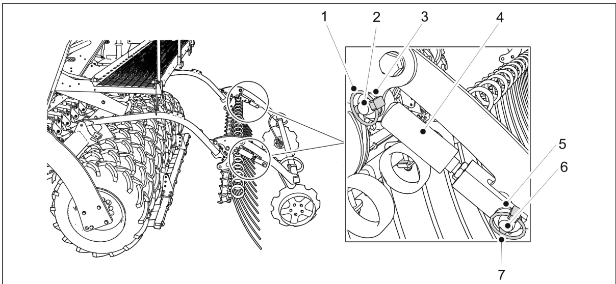
Kuva. 7.4.1. - 220. Takamerkkarisylinterien irrotus
