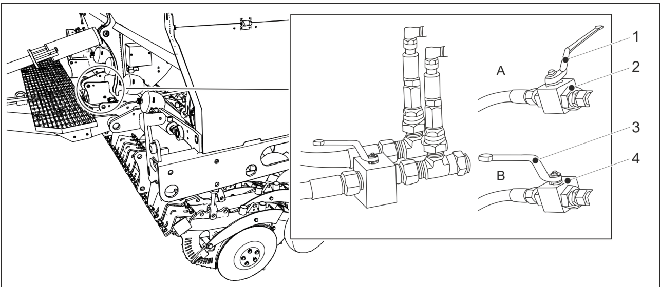
Kuva. 5.3.5. - 89. Nostopiirin sulkuhanat
