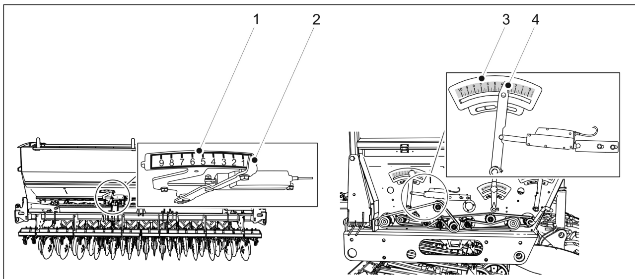
Kuva. 7.1.14. - 192. Lannoitteen kaukosäädön toiminnan tarkastus. Vasemmalla kone, jossa ei ole vaihdelaatikkoa tai on vaihdelaatikko siemenpuolelle (telamalli). Oikealla kone, jossa on tuplavaihteisto (vaihdelaatikkomalli).
