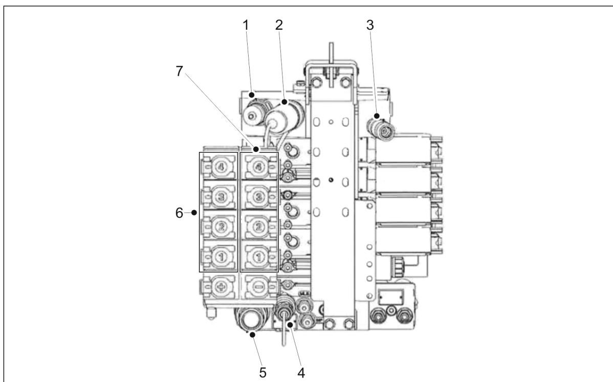
Kuva. 5.3. - 79. Kytkeämallina Valtran T-sarjan hydrauliliitännät
