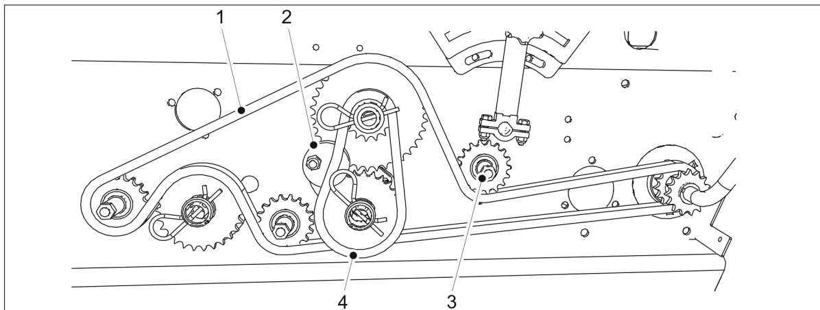
Kuva. 7.5.1. - 232. Ketjujen kiristys koneessa, jossa ei ole vaihdelaatikkaa
