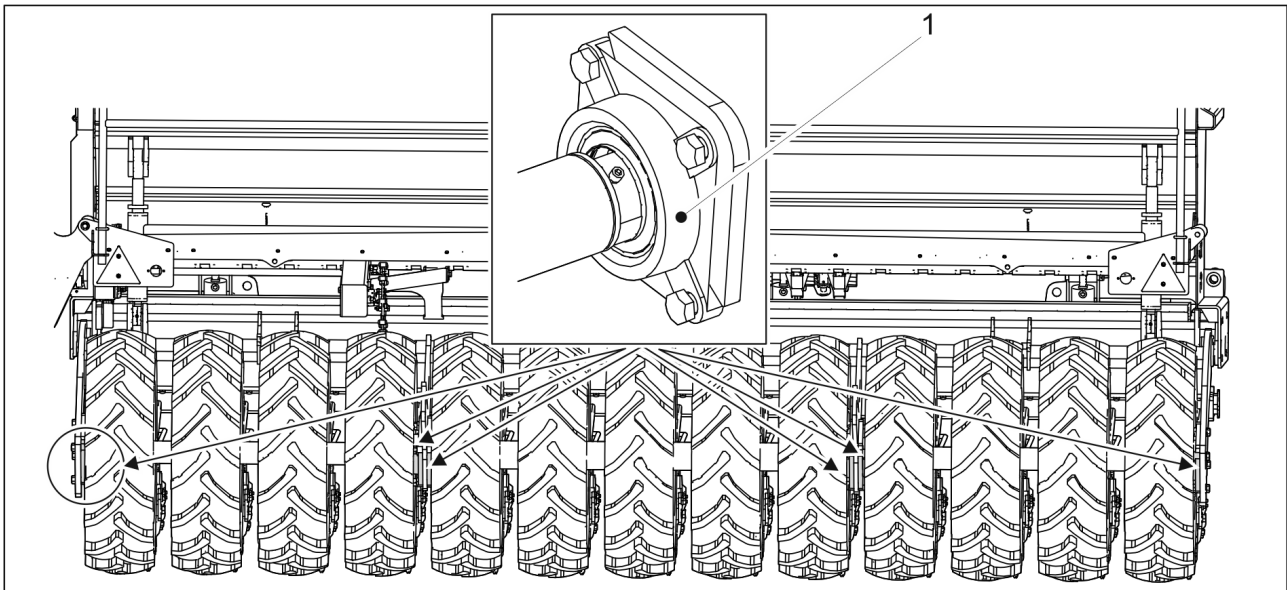
Kuva. 7.2.5. - 201. Pyöräakselien laakerit
