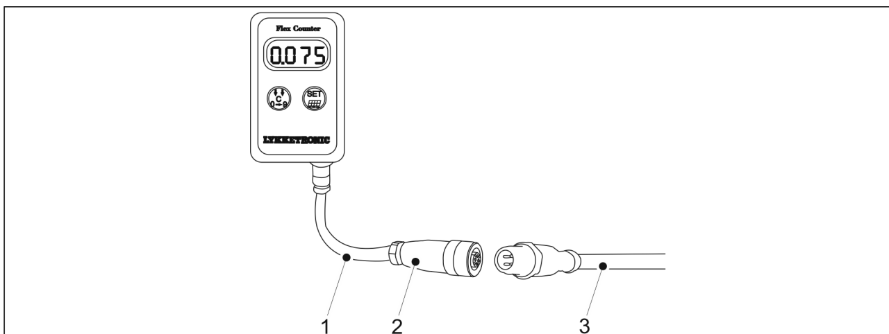
Kuva. 5.2.1. - 72. Pinta-alamittarin asentaminen
