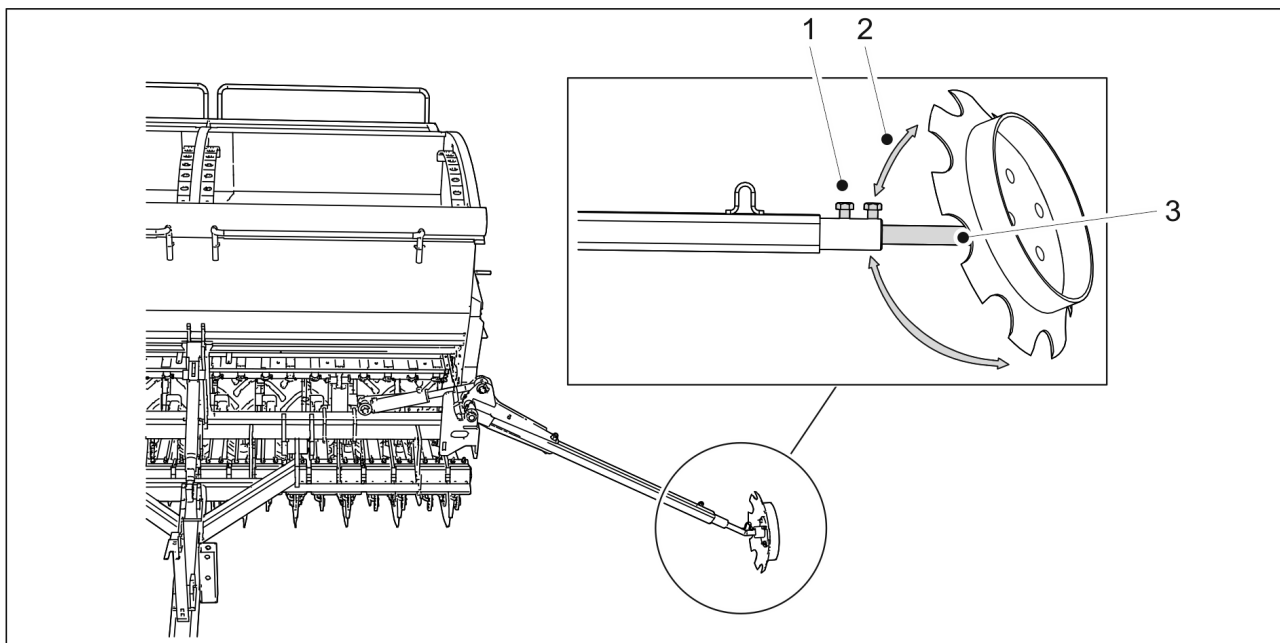
Kuva. 5.3.7. - 90. Keskimerkkarien säätäminen
