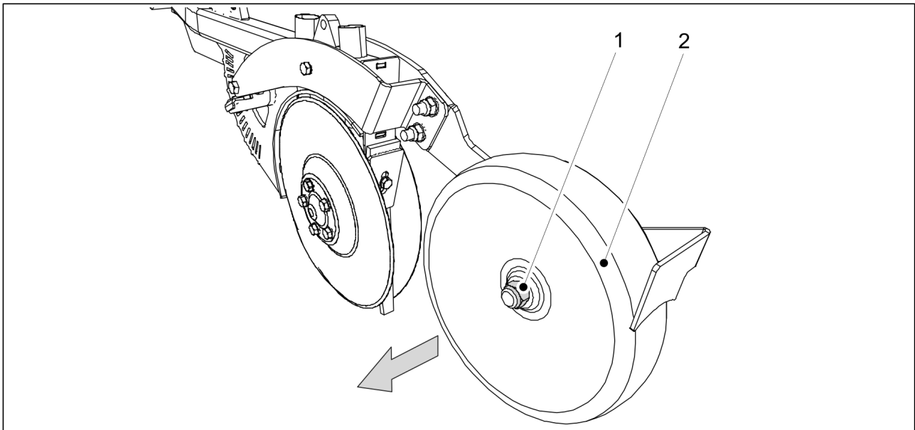
Kuva. 7.9.4.1. - 258. Peittopyörän irrotus
