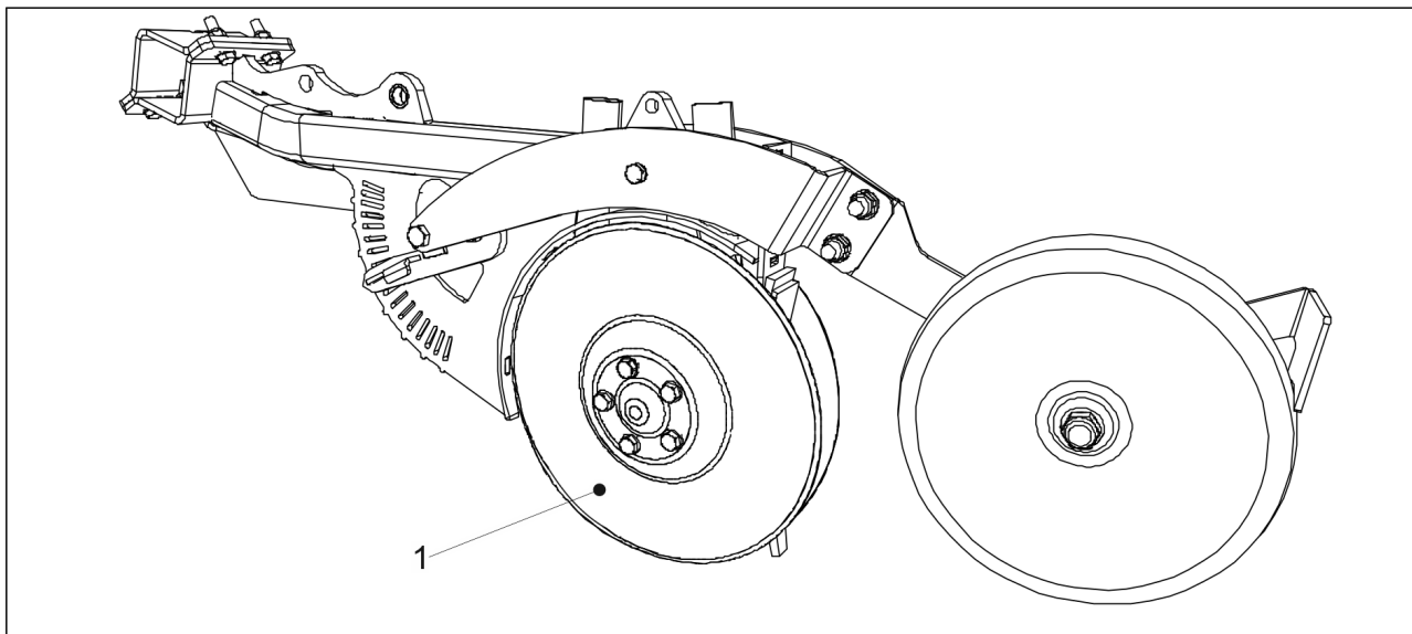
Kuva. 7.1.13. - 191. Vantaan kiekot
