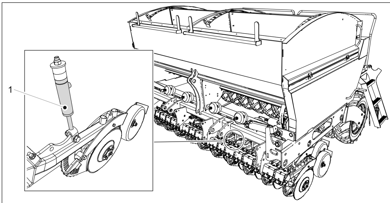
Kuva. 6.10. - 162. Vannaspainatuksen säätäminen
