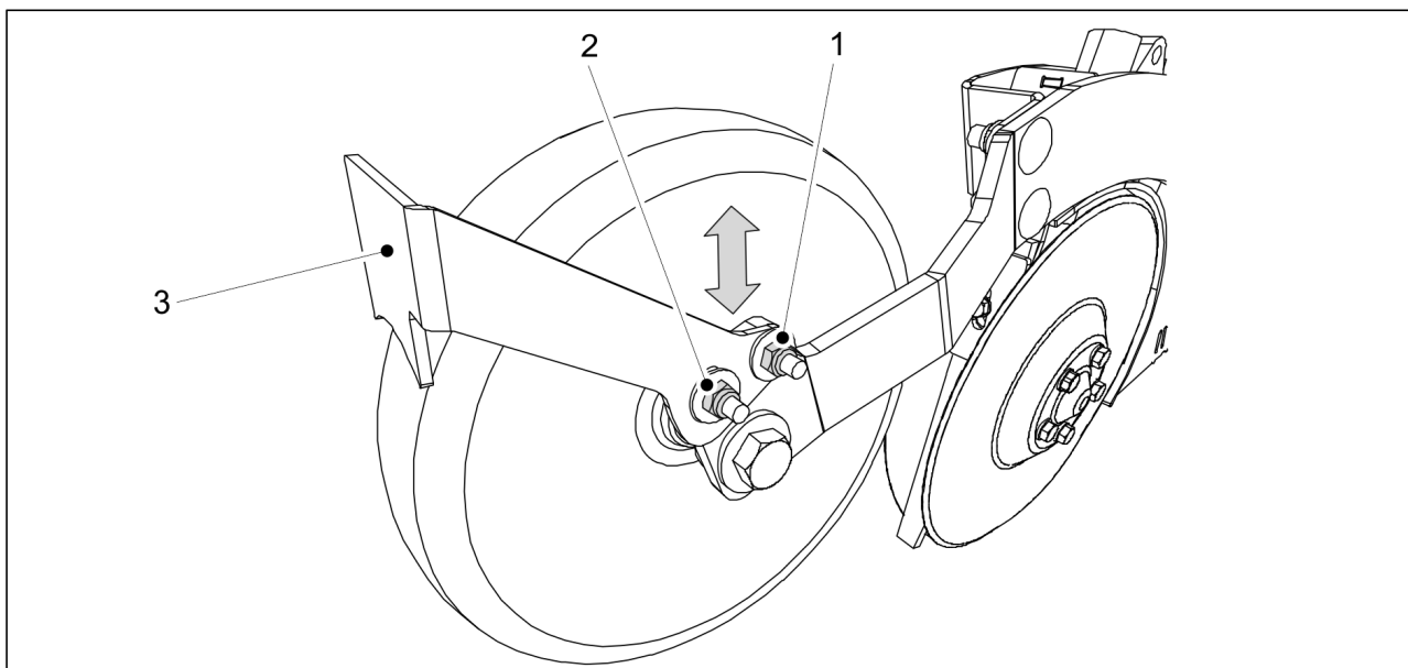
Kuva. 7.9.5.2. - 261. Peittopyörän raappalevy
