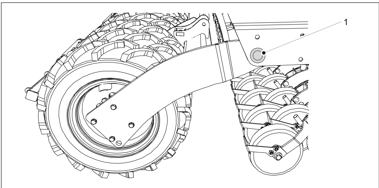
Kuva. 7.2.4. - 200. Taka-akselin kiinnitys
