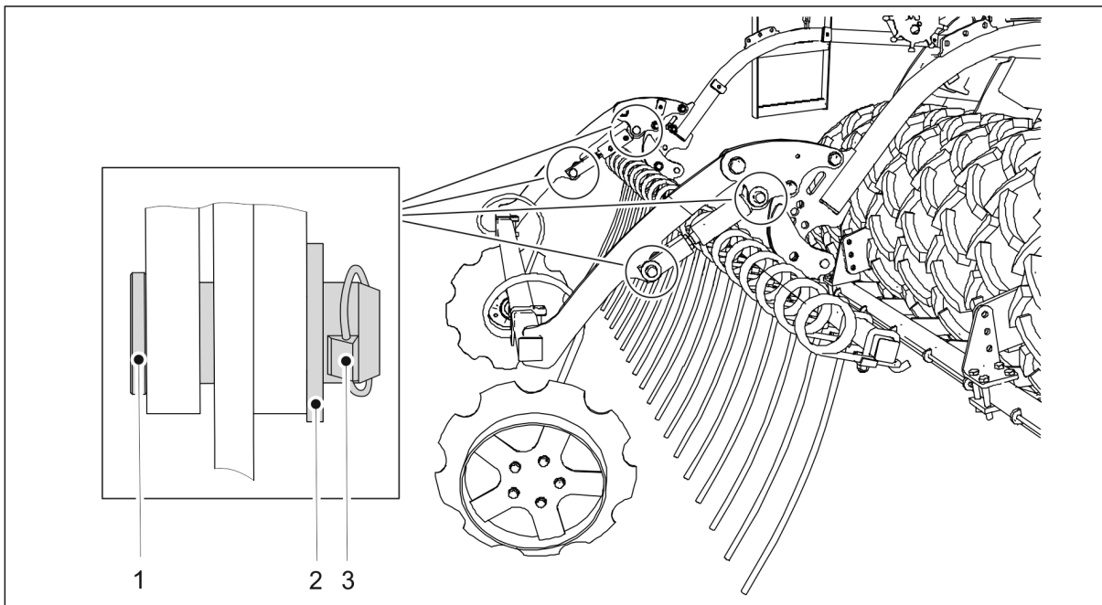
Kuva. 5.1.9. - 69. Takamerkkarisylinterien kiinnittäminen
