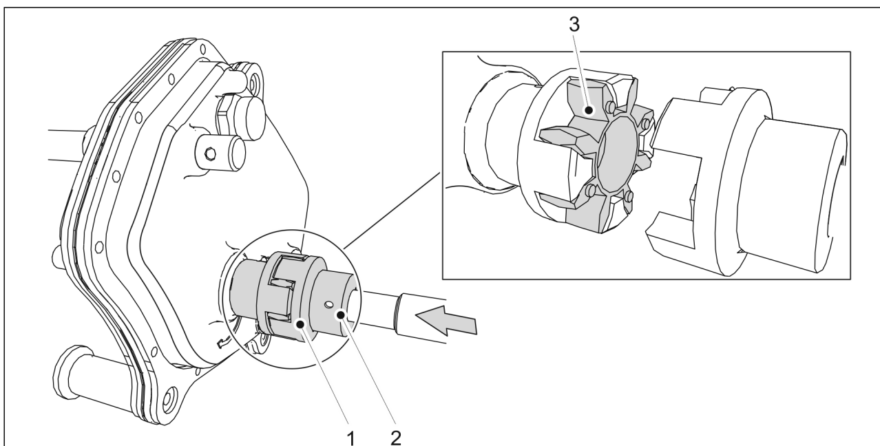
Kuva. 7.7.2.2. - 241. Kytkimen asennus
