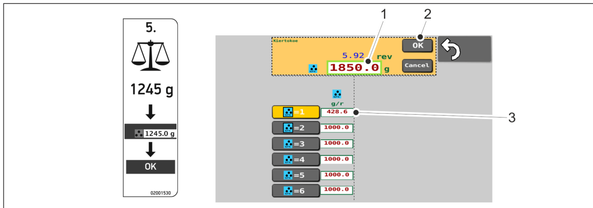
Kuva. 6.8.3. - 145. Punnitustuloksen syöttäminen
