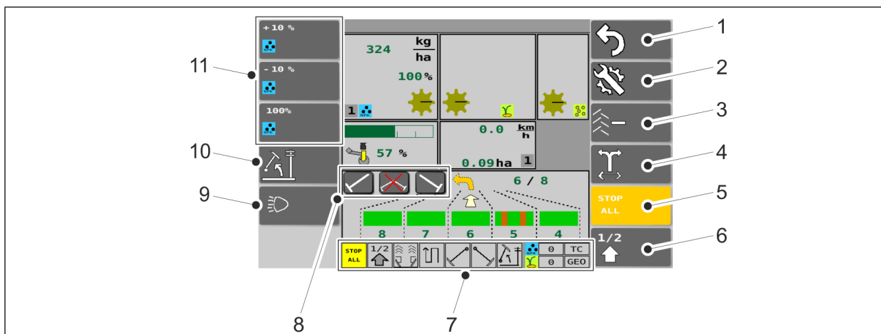
Kuva. 4.2.4.1. - 42. Ajonäyttö-sivun painikkeet
