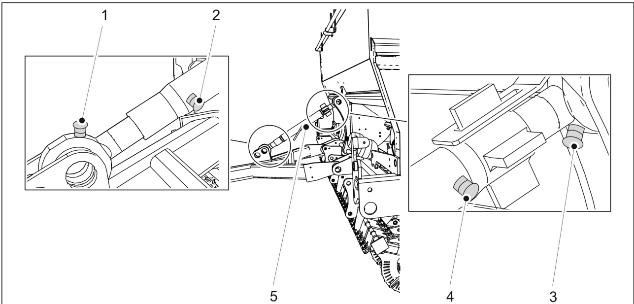
Kuva. 7.2.13. - 211. Vanttiruuvi
