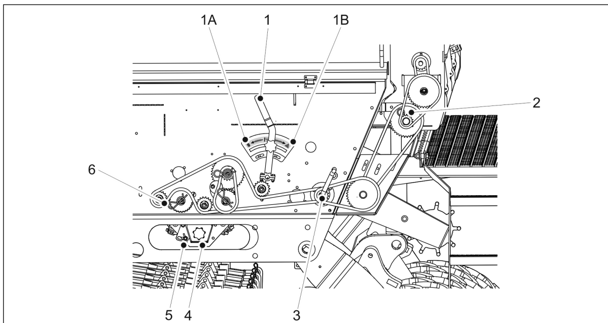
Kuva. 6.8.5. - 156. Siementen kiertokoe koneessa, jossa ei ole vaihdelaatikkoo.
