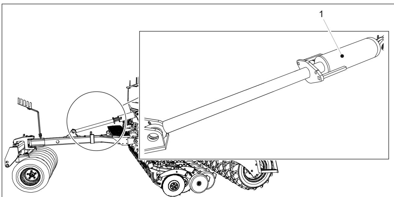
Kuva. 7.2.12. - 210. Aisasyylinteri
