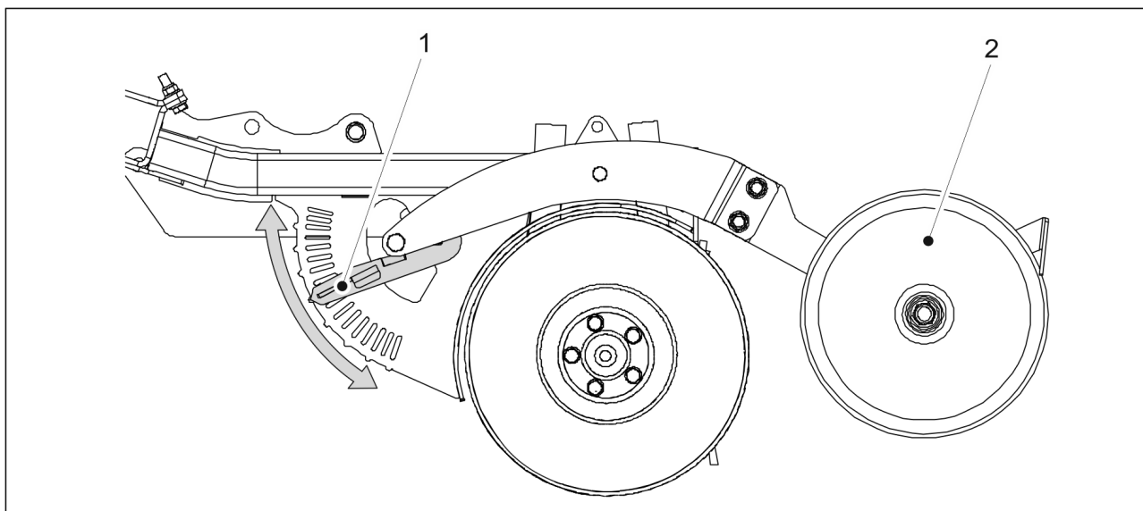
Kuva. 6.9. - 160. Vantaan kylvösyvyyden säätäminen
