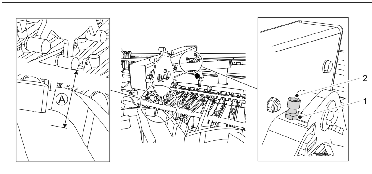
Kuva. 7.1.8. - 188. Pyörävedon toimintavälyksen tarkastus
