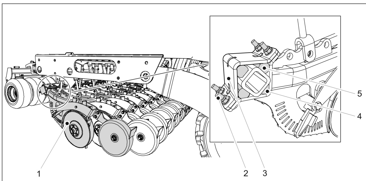
Kuva. 7.9.1.2. - 247. Vantaan kiinnitys
