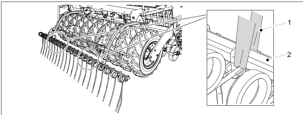
Kuva. 5.1.8. - 65. Jälkiharan nostaminen
