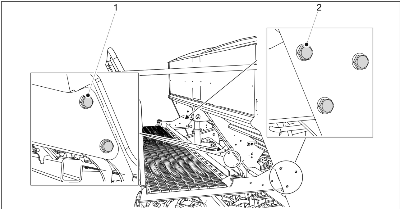
Kuva. 7.1.2.5. - 177. Hoitotason pultit
