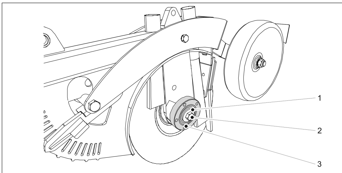
Kuva. 7.9.2.1. - 251. Laakeripesän irrotus
