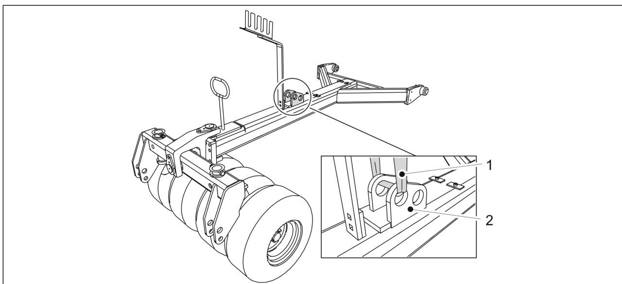
Kuva. 5.1.1. - 51. Pyöränvälijyrän nostaminen
