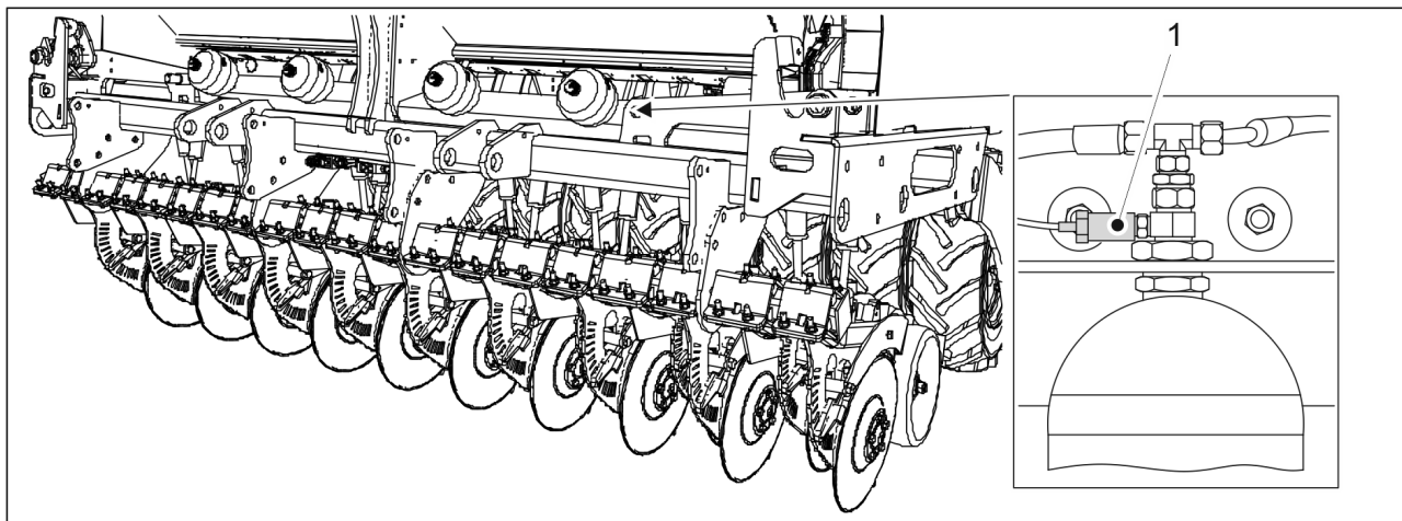
Kuva. 4.2.1.9. - 23. Vannaspainatusanturi
