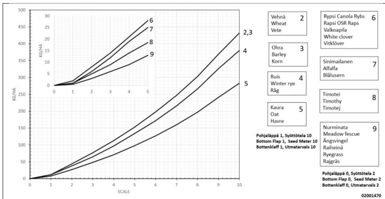
Kuva. 6.5. - 116. Kylvötaulukko, siemen- ja lannoitevaihdelaatikko 1
