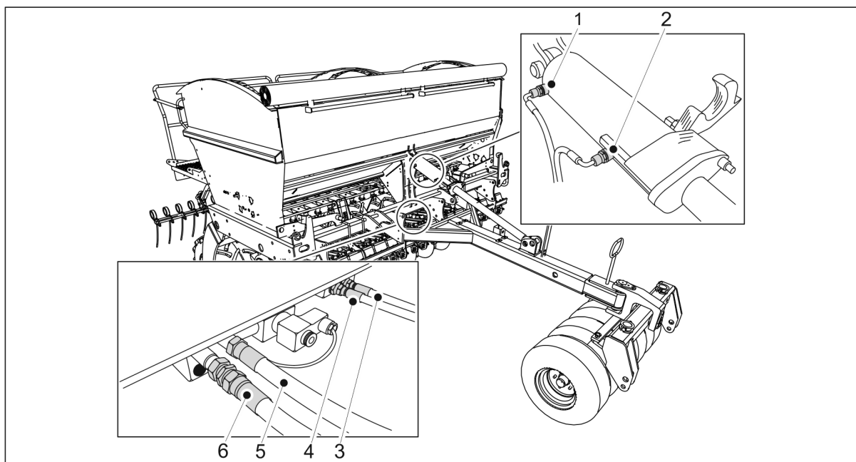
Kuva. 5.1.1. - 54. Hydrauliletkujen kytkentä
