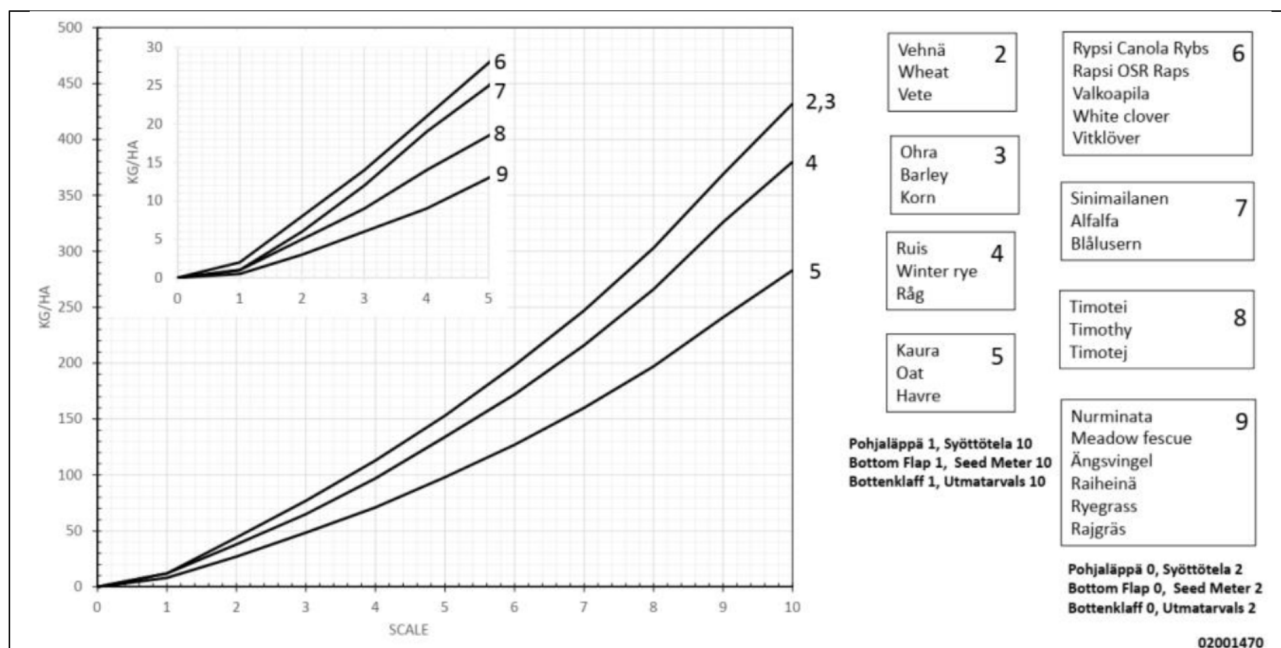
Kuva. 6.5. - 113. Kylvötaulukko, siemenvaihdelaatikko 1
