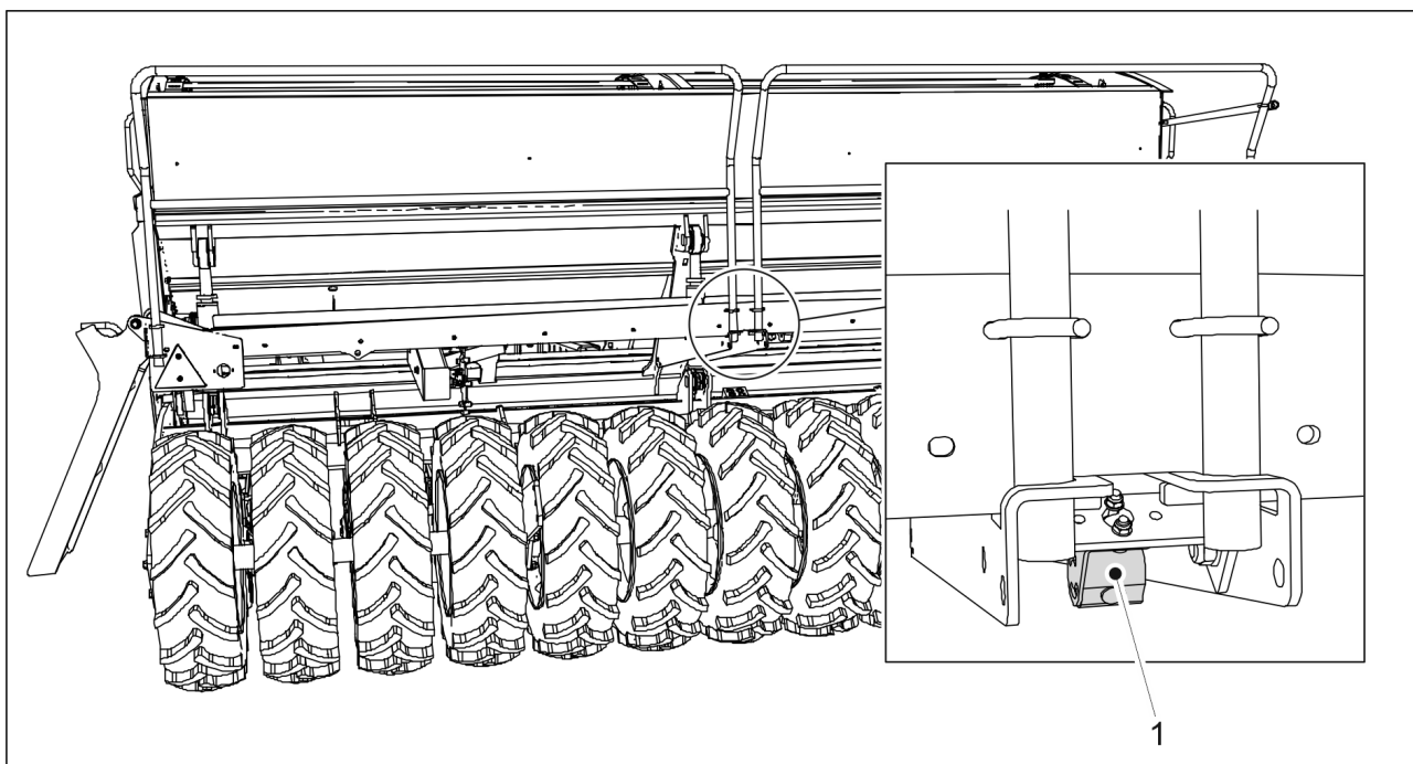
Kuva. 4.2.1.12. - 26. Peruutuskamera
