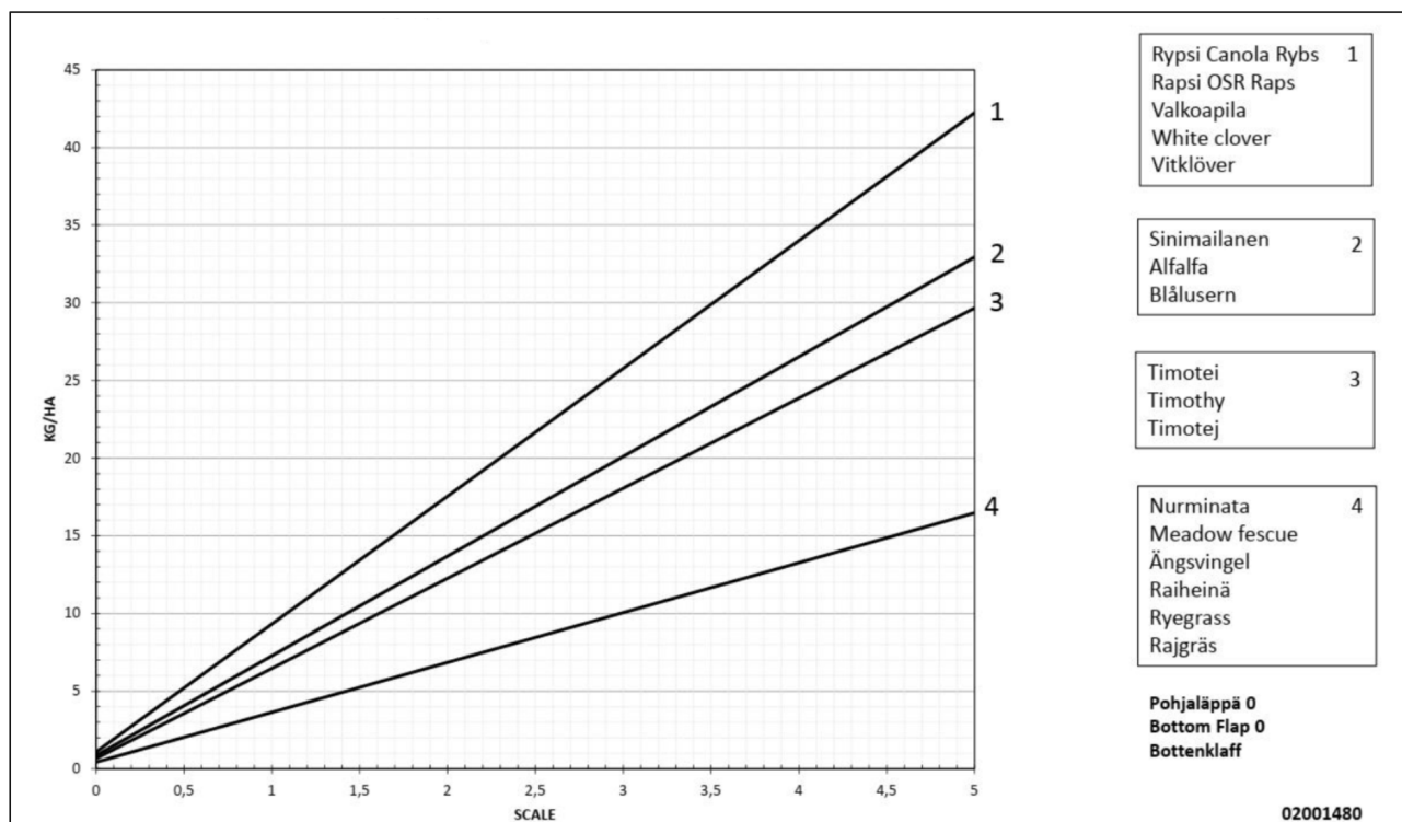
Kuva. 6.5. - 112. Kylvötaulukko, piensiemensäiliö
