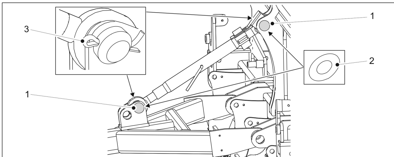
Kuva. 5.1.3. - 56. Vanttiruuvi
