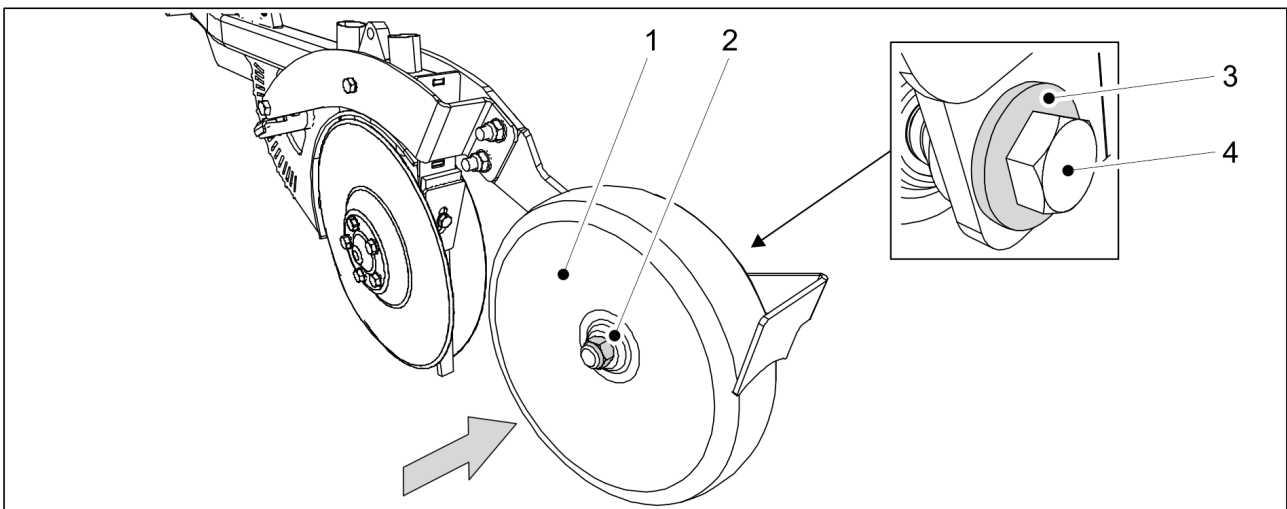
Kuva. 7.9.4.2. - 259. Peittopyörän asennus
