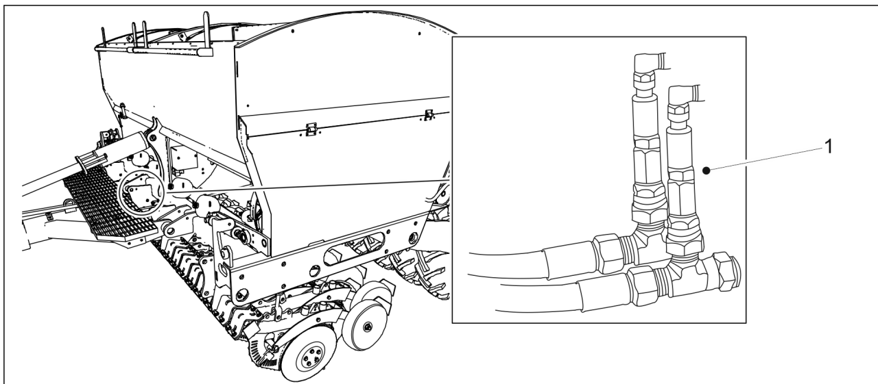
Kuva. 4.2.1.10. - 24. Nosto- ja laskupiirin paineanturit
