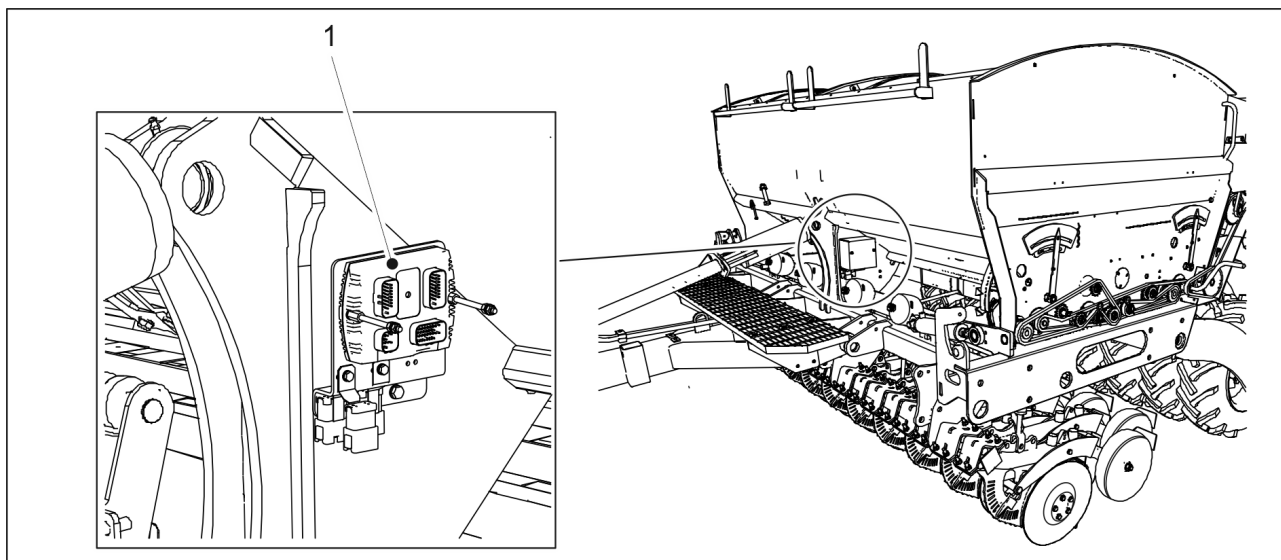
Kuva. 4.2.1.1. - 14. Ohjausyksikkö
