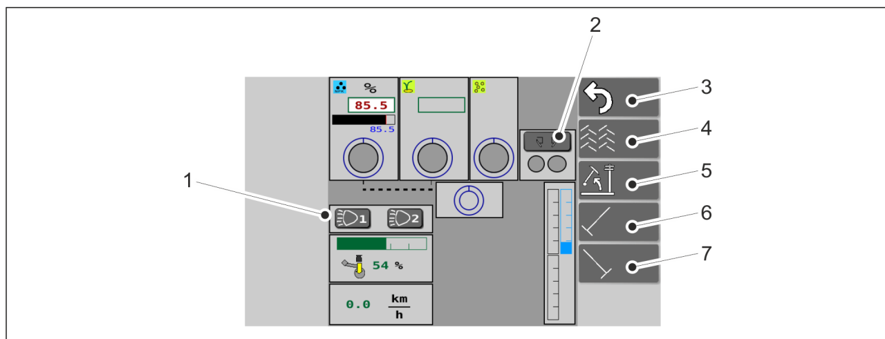
Kuva. 4.2.4.3. - 47. Manuaalikäyttö-sivun painikkeet
