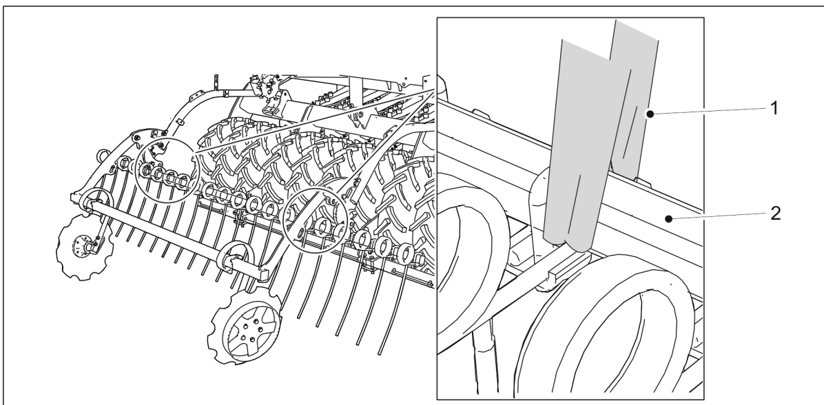
Kuva. 7.4.1. - 222. Jälkiharan nostaminen
