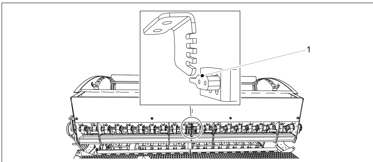
Kuva. 7.3.2. - 214. Pohjaläppä auki
