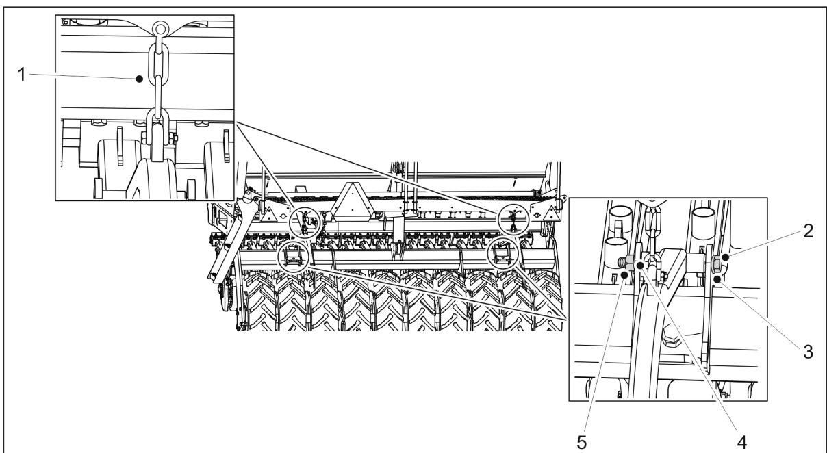
Kuva. 7.4.1. - 221. Jälkiharan irrotus
