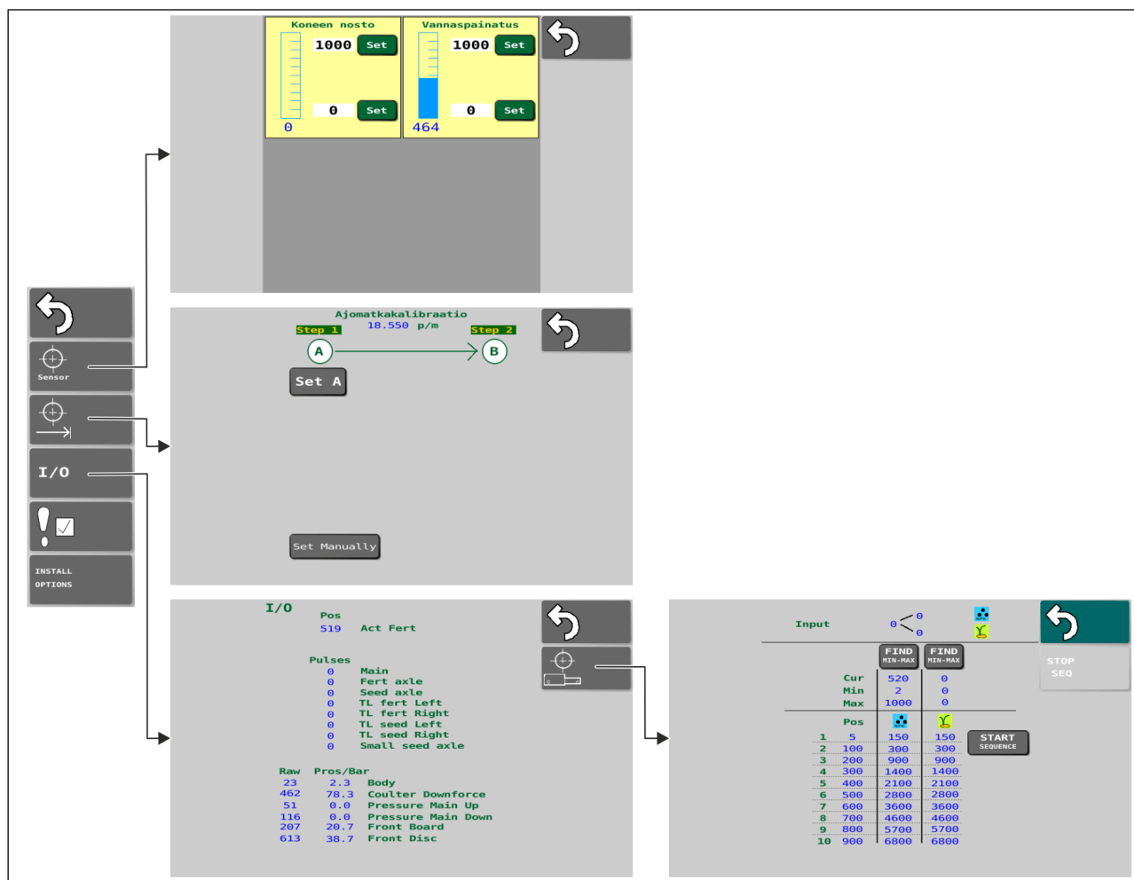
Kuva. 4.2.3. - 40. Anturien asetukset
