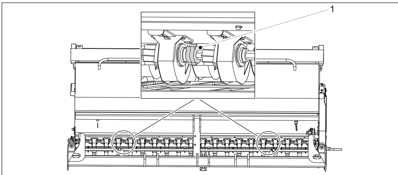
Kuva. 4.2.1.6. - 19. Ajourakytkimet
