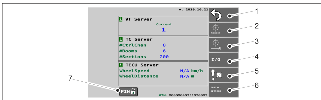
Kuva. 4.2.4.4. - 49. Perusasetukset
