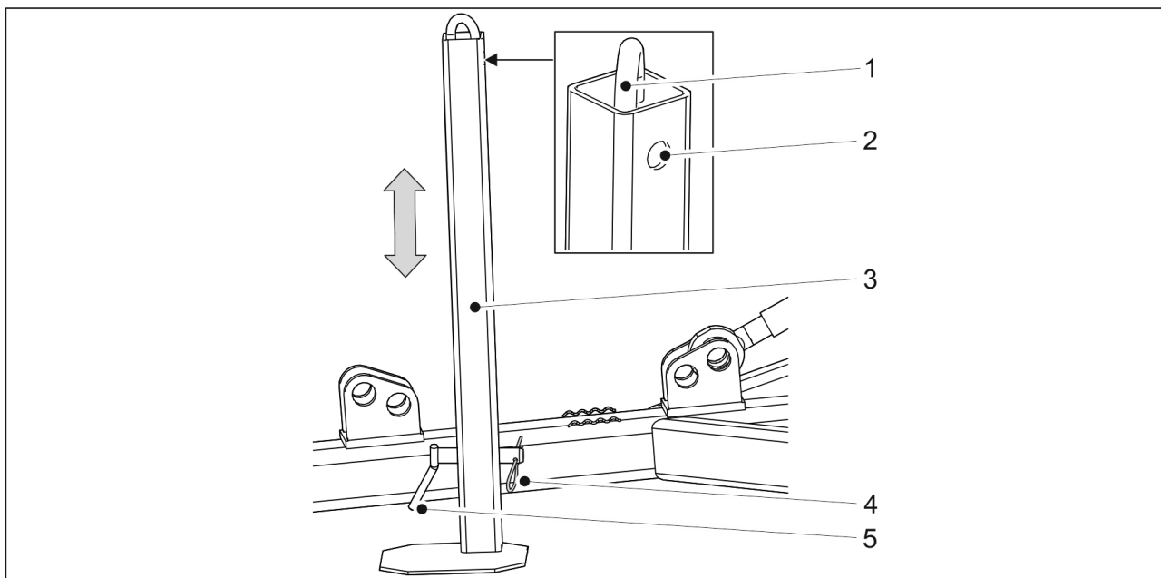
Kuva. 5.3.2. - 84. Maatuki
