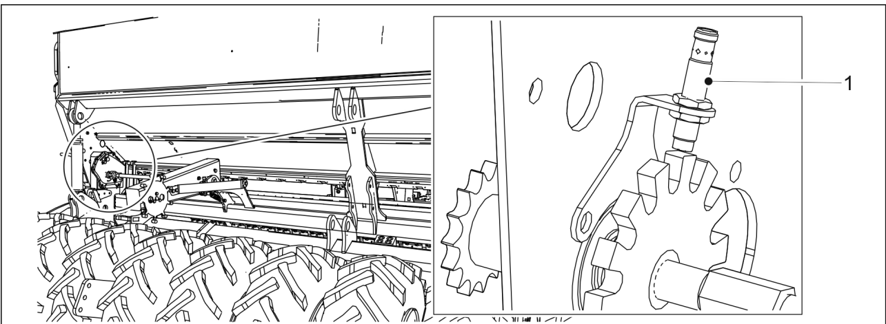
Kuva. 4.2.1.3. - 16. Nopeusanturi
