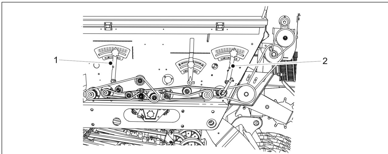
Kuva. 6.6.7. - 123. Vaihdelaatikoiden säätövivut
