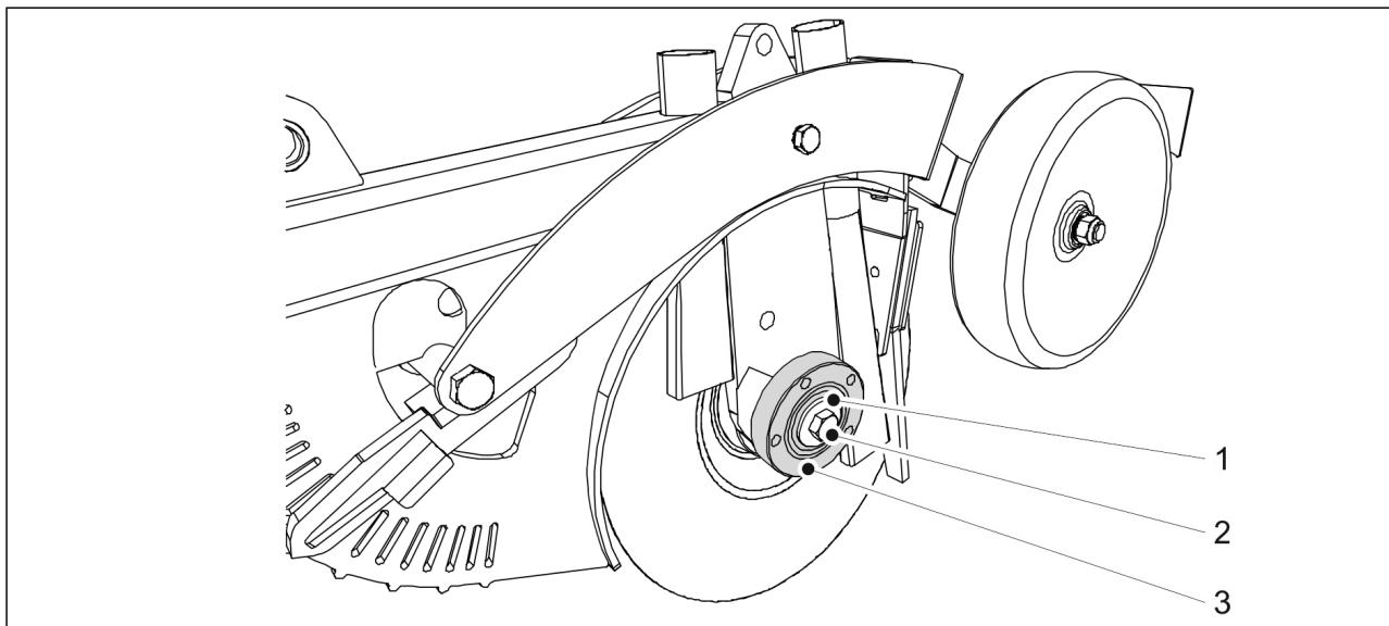
Kuva. 7.9.2.2. - 252. Laakeripesän asennus
