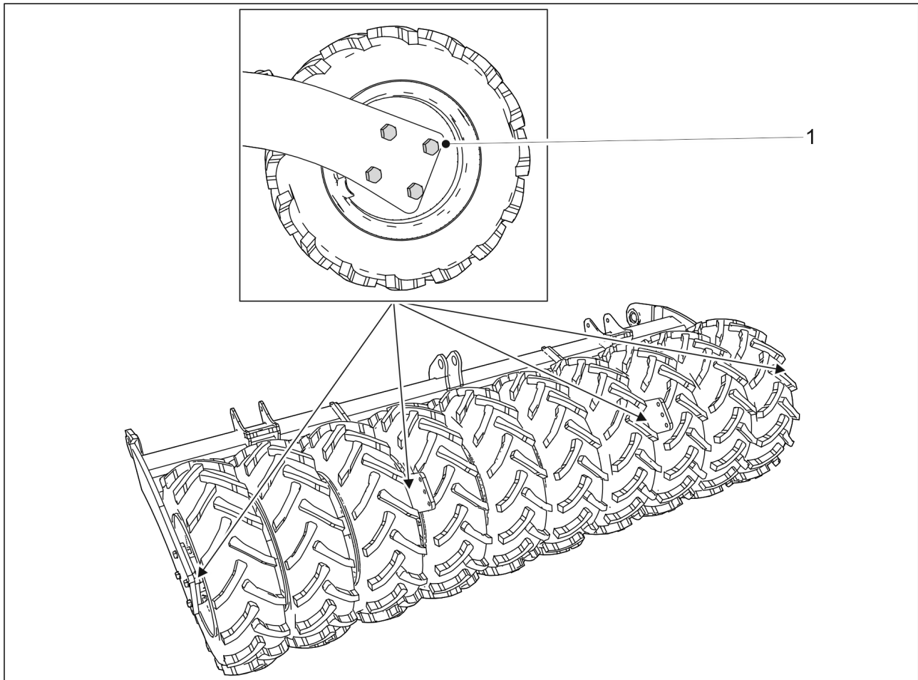
Kuva. 7.1.2.2. - 172. Kuljetuspyörästäön laippalaakereiden pultit
