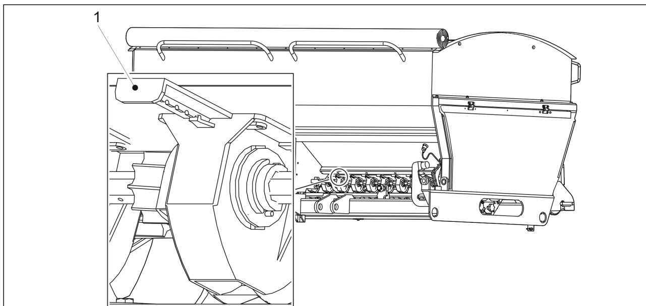
Kuva. 6.6.9. - 126. Sulkuluukun asennon säätäminen
