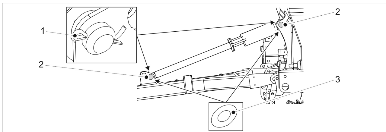
Kuva. 5.1.2. - 55. Aisasyylinteri
