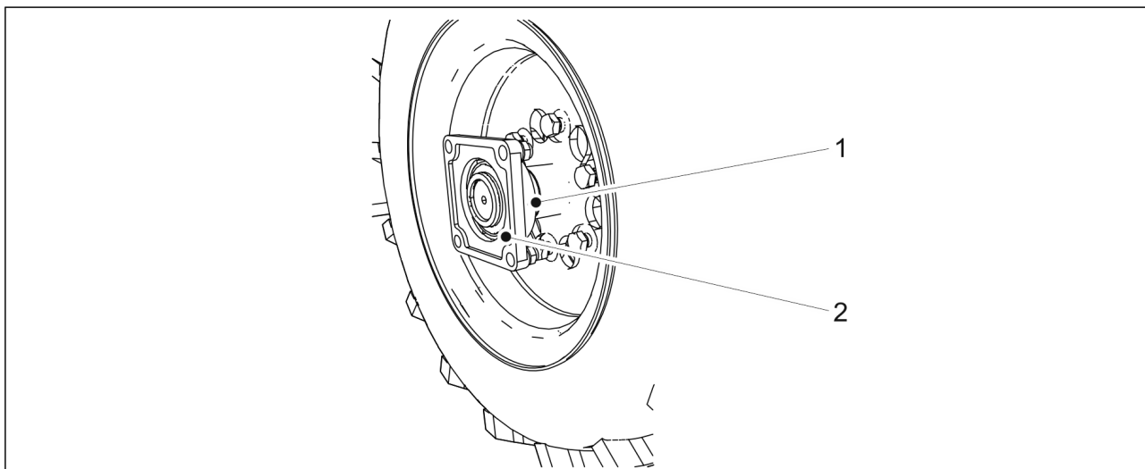
Kuva. 7.4.2. - 227. Laippalaakerin irrotus
