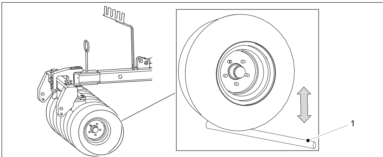
Kuva. 7.1.4. - 180. Pyöränvälilyrjän napojen laakerivällyksen tarkistus
