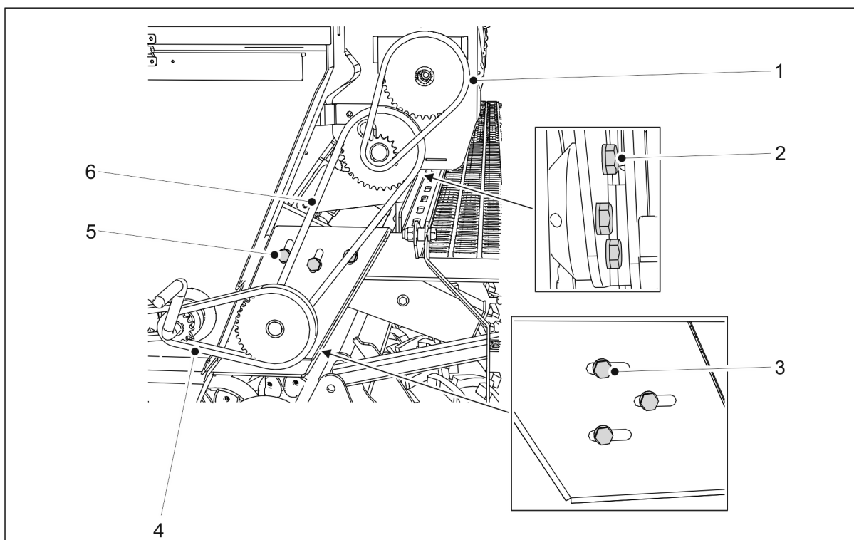
Kuva. 7.5.4. - 235. Piensiemensäiliön voimansiirron ketjujen kiristys
