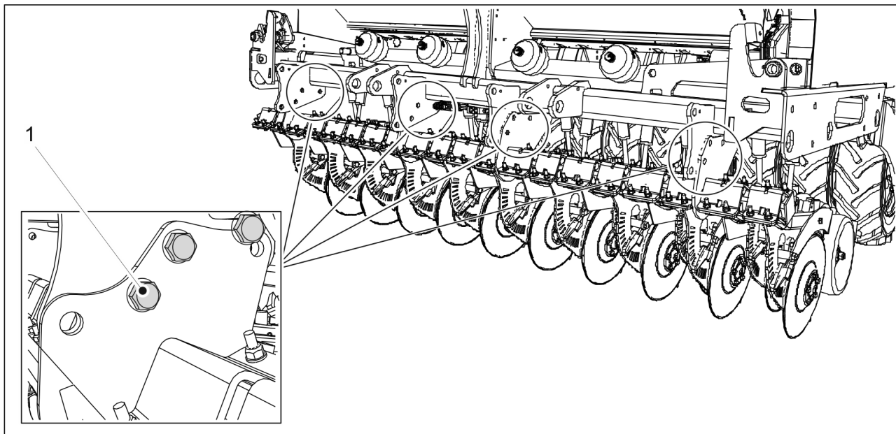
Kuva. 7.1.2.4. - 175. Vannasvarren pultit
