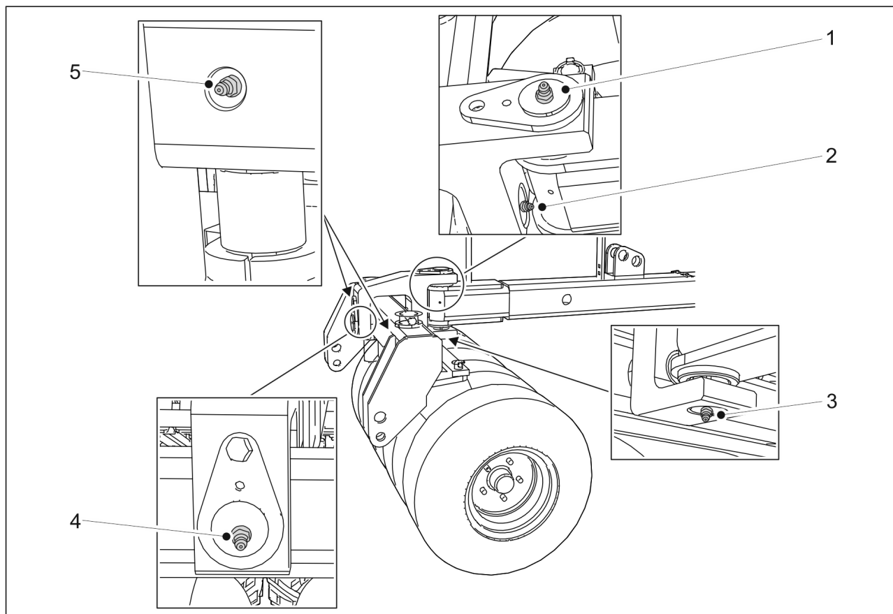
Kuva. 7.2.10. - 206. Pyöränvälilyyrän tapit
