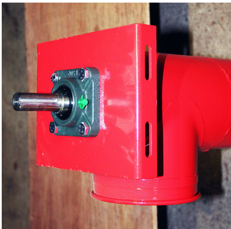
Yläpään laakeri asennettuna paikalleen
