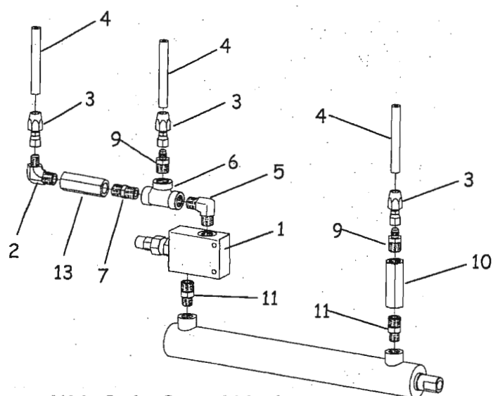
Vérin Cadre Central / 1er bras
