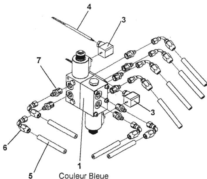
Montage avec sélecteur filt. 3/8 Couleur BLEUE
