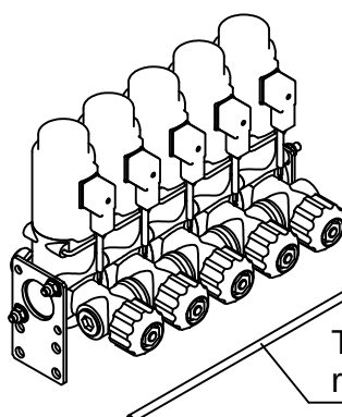
Bloc complet 5 vannes réf : G9000294
