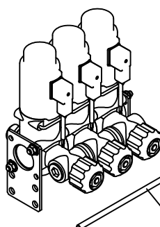
Bloc complet 4 vannes réf : G9000293
