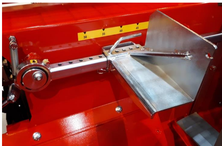
Kuva 15: Mittalaitteen asento suurille, halkaisijaltaan yli 25cm puille
