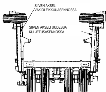
KUVASSA 4.6 METRIN KONE ALIMMASSA KÄYTTÖASENNOSSA
