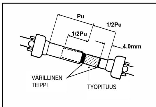
Nivelakseli maksimipituudessaan Kuva 11
