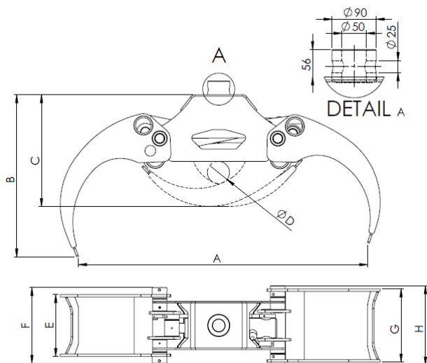
Kuva 3 0,15 / 0,12 / 0,24 / 0,27 tarraimen (mm) mitat
