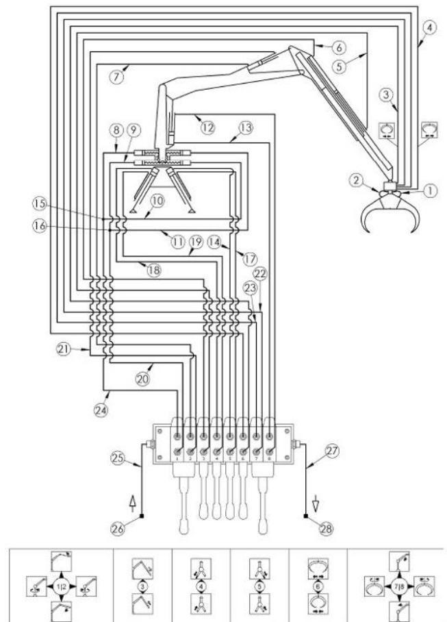
Kuva 2 Hydraulikaavio 6/8 XY -ohjausventtiilillä
