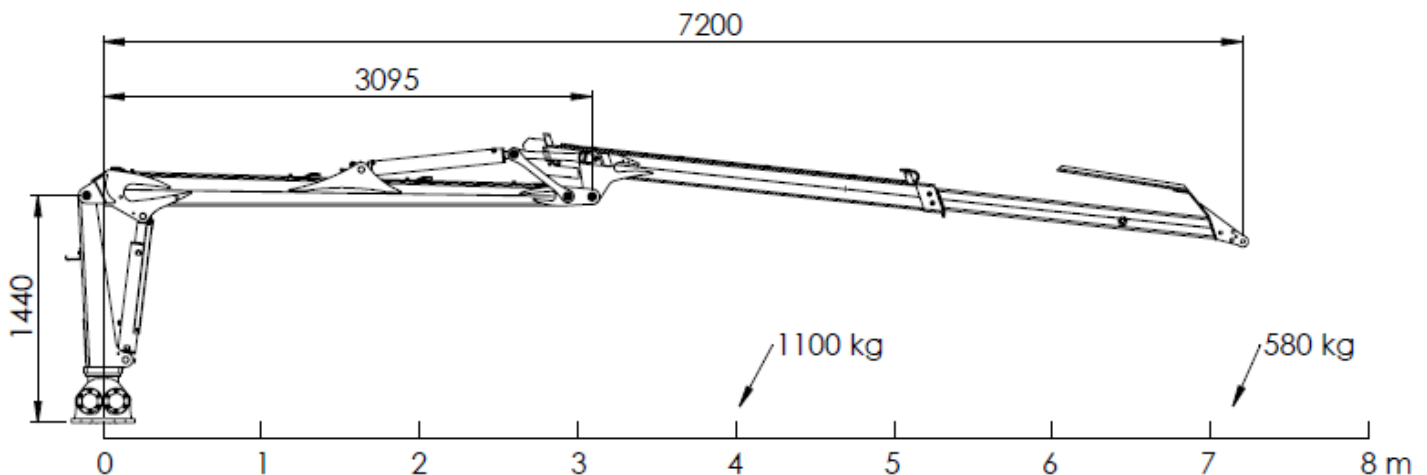
Kuva 1 BMF 720 mitat ( mm)
