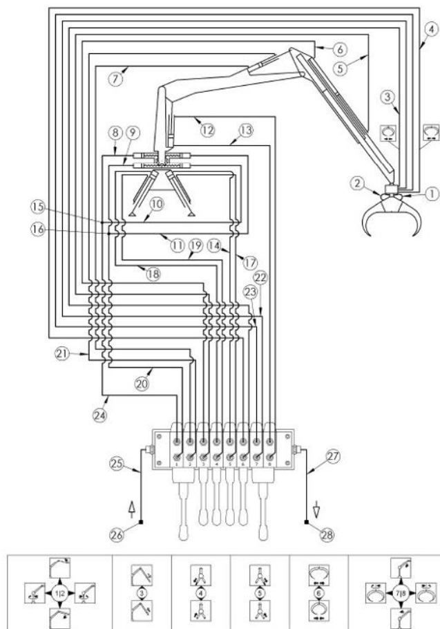
Kuva 2 Hydraulikaavio 6/8 XY -ohjausventtiilillä
