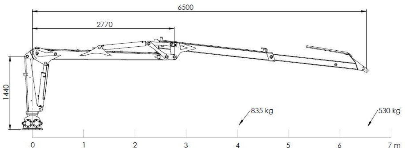
Kuva 1 BMF 650 mitat ( mm)
