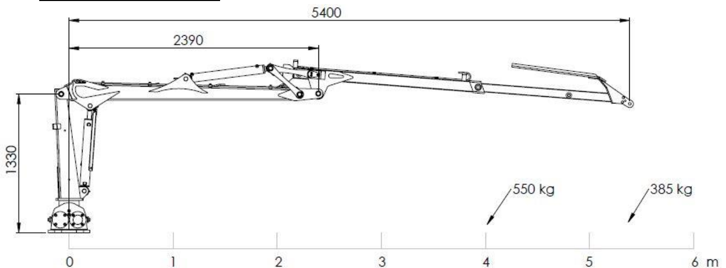
Kuva 1 BMF 540 mitat ( mm)
