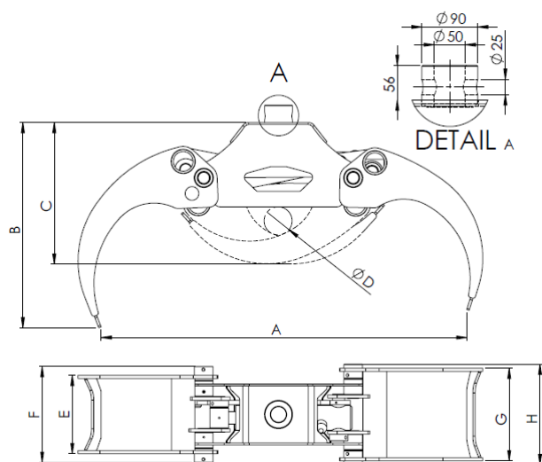
Kuva 3 0,15 / 0,2 / 0,24 / 0,27 tarraimen (mm) mitat
